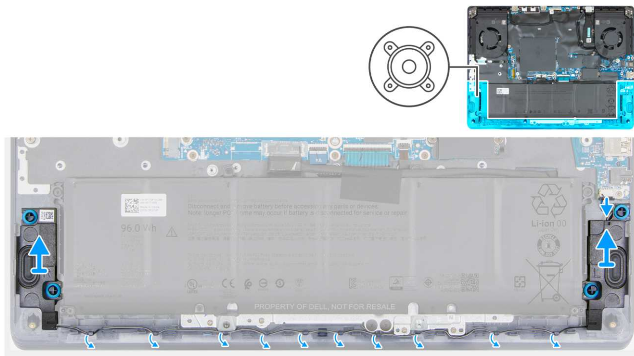
Rysunek 35. Wymontowywanie głośników
