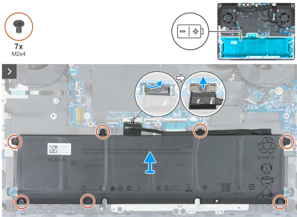
Rysunek 17. Wymontowywanie baterii
