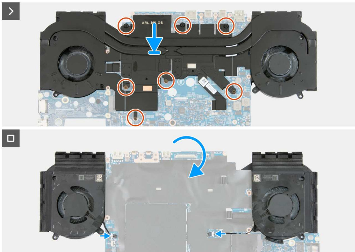
Rysunek 54. Instalowanie zestawu wentylatora i radiatora
