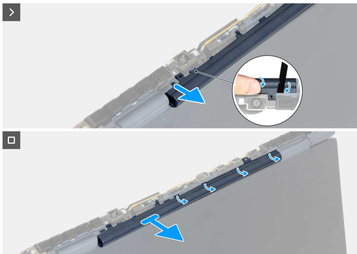
Rysunek 68. Wymontowywanie listwy środkowej
