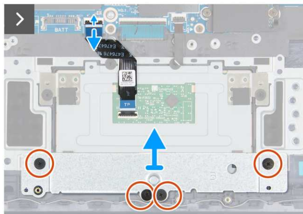
Rysunek 43. Wymontowywanie touchpada
