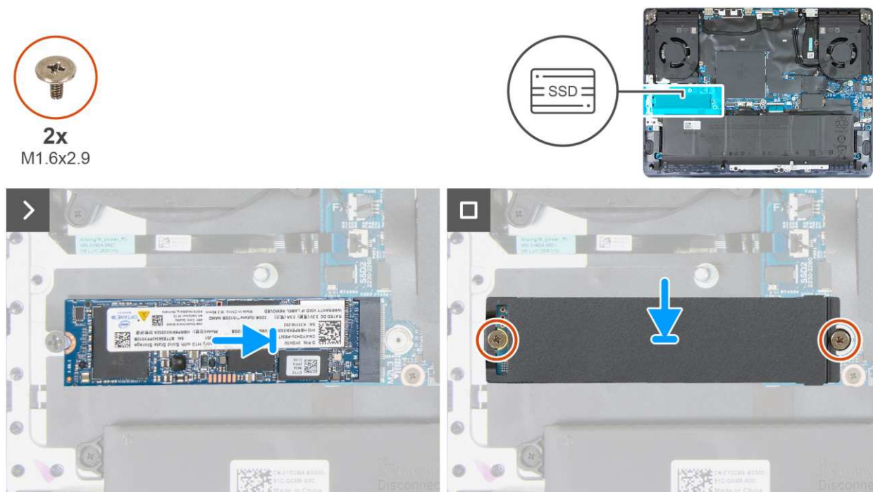
Rysunek 30. Instalacja dysku SSD M.2 2280 w gnieździe SSD2
