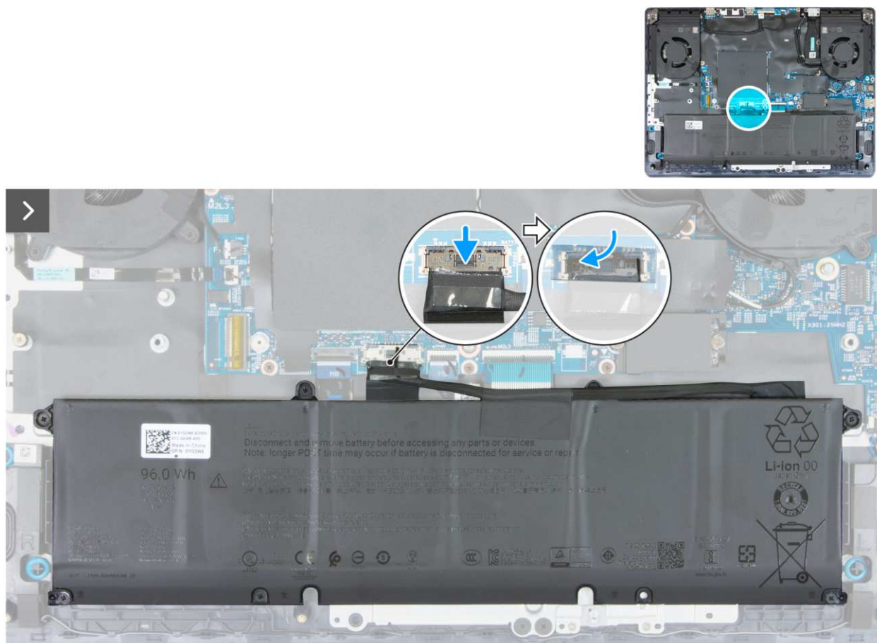
Rysunek 14. Podłączanie kabla baterii
