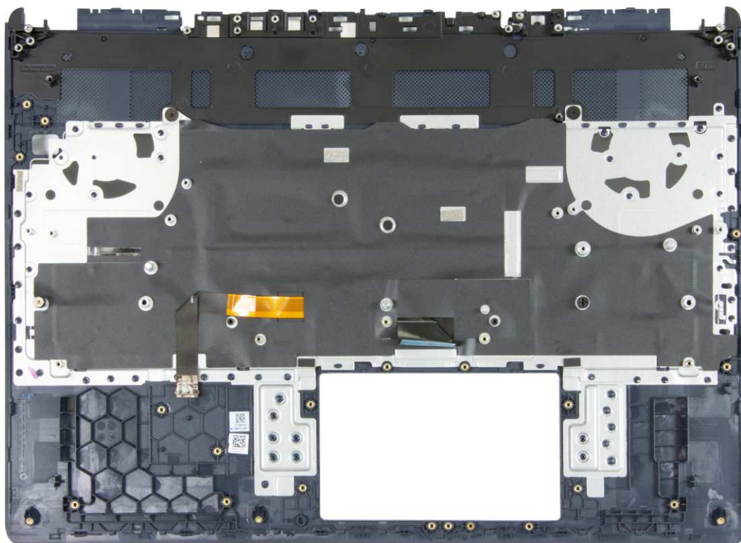
Rysunek 76. Wymontowywanie zestawu podparcia dłoni i klawiatury
