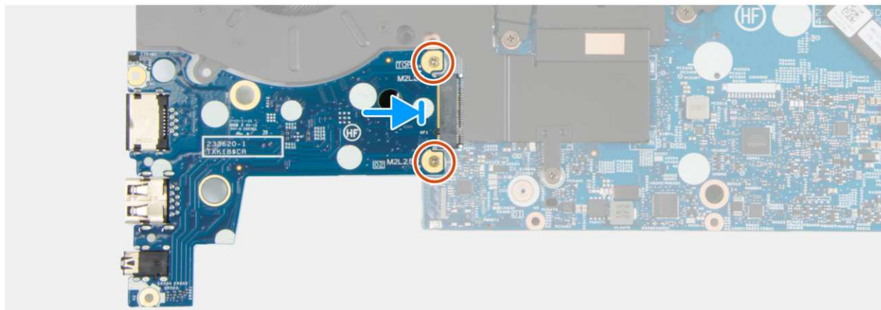
Rysunek 53. Instalowanie płyty we/wy
