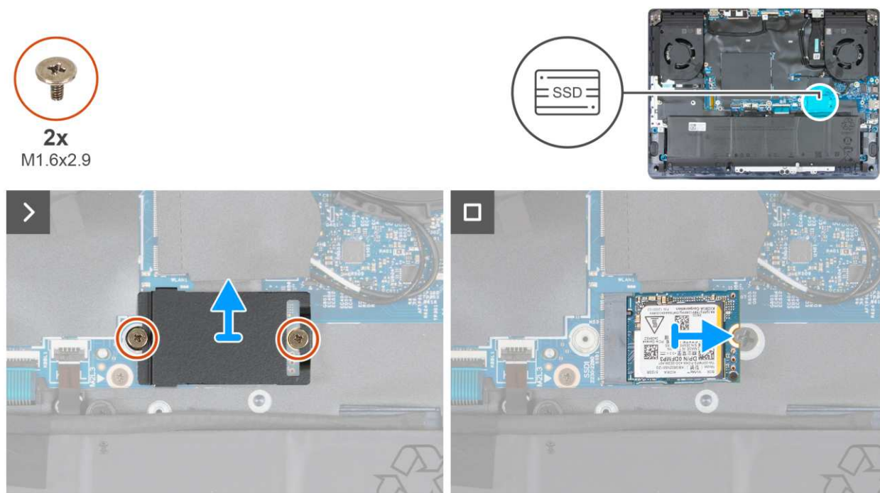
Rysunek 23. Wymontowywanie dysku SSD M.2 2230 z gniazda SSD1
