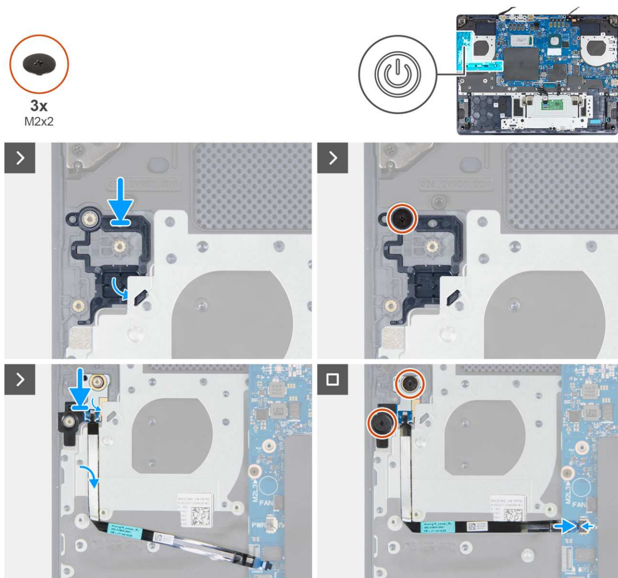
Rysunek 59. Instalacja przycisku zasilania i płyty przycisku zasilania
