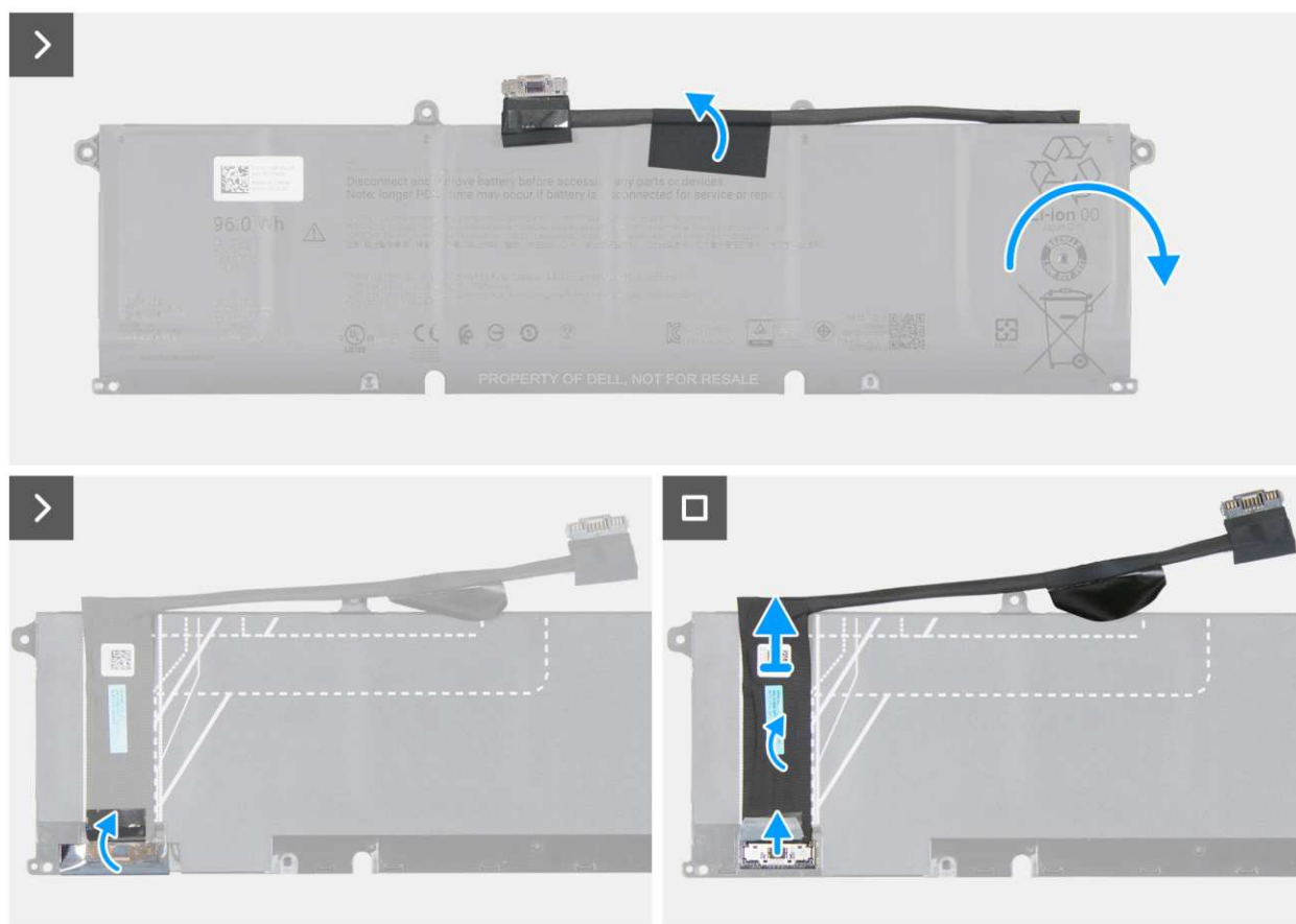
Rysunek 19. Wymontowywanie kabla baterii
