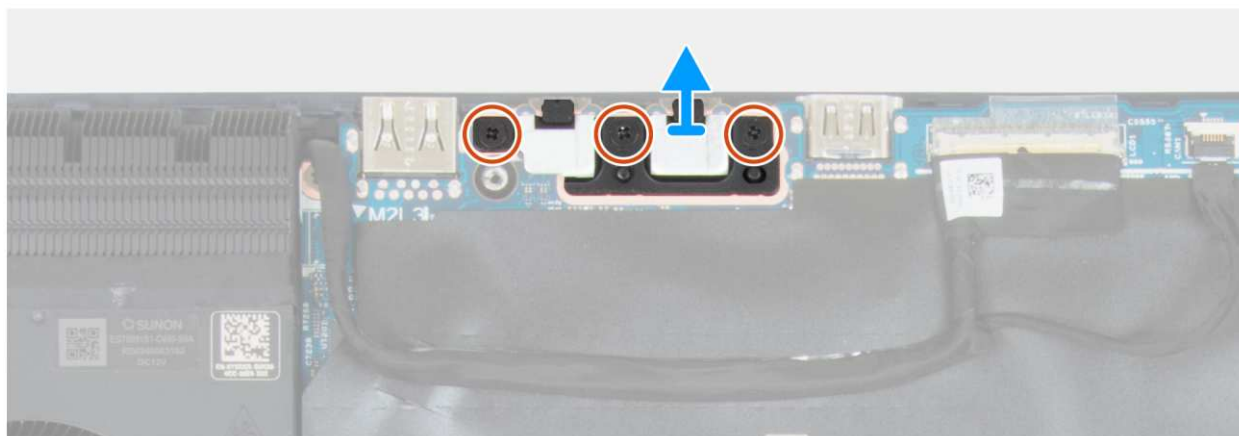
Rysunek 39. Wymontowywanie klamry złącza Type-C
