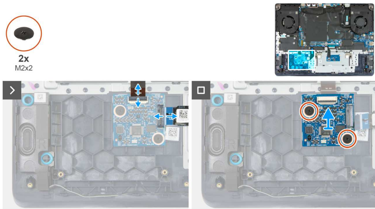
Rysunek 45. Wymontowywanie płyty kontrolera podświetlenia klawiatury (ELC)
