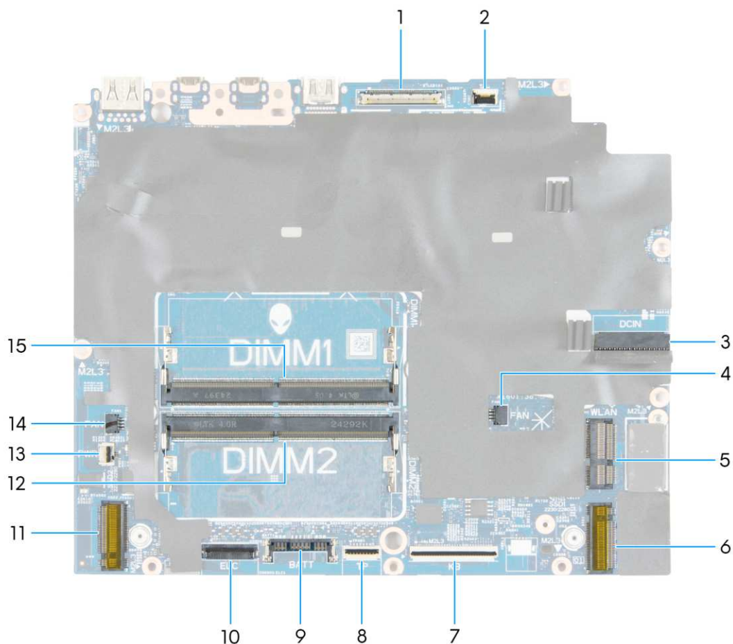
Rysunek 47. Złącza płyty głównej
