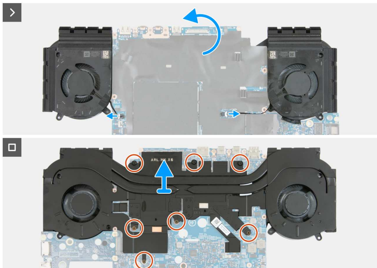
Rysunek 60. Wymontowywanie zestawu wentylatora i radiatora
