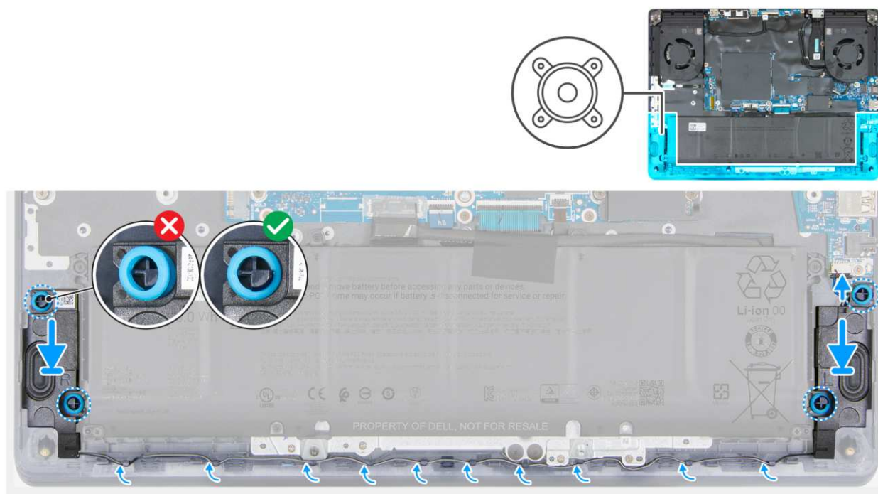
Rysunek 36. Instalowanie głośników
