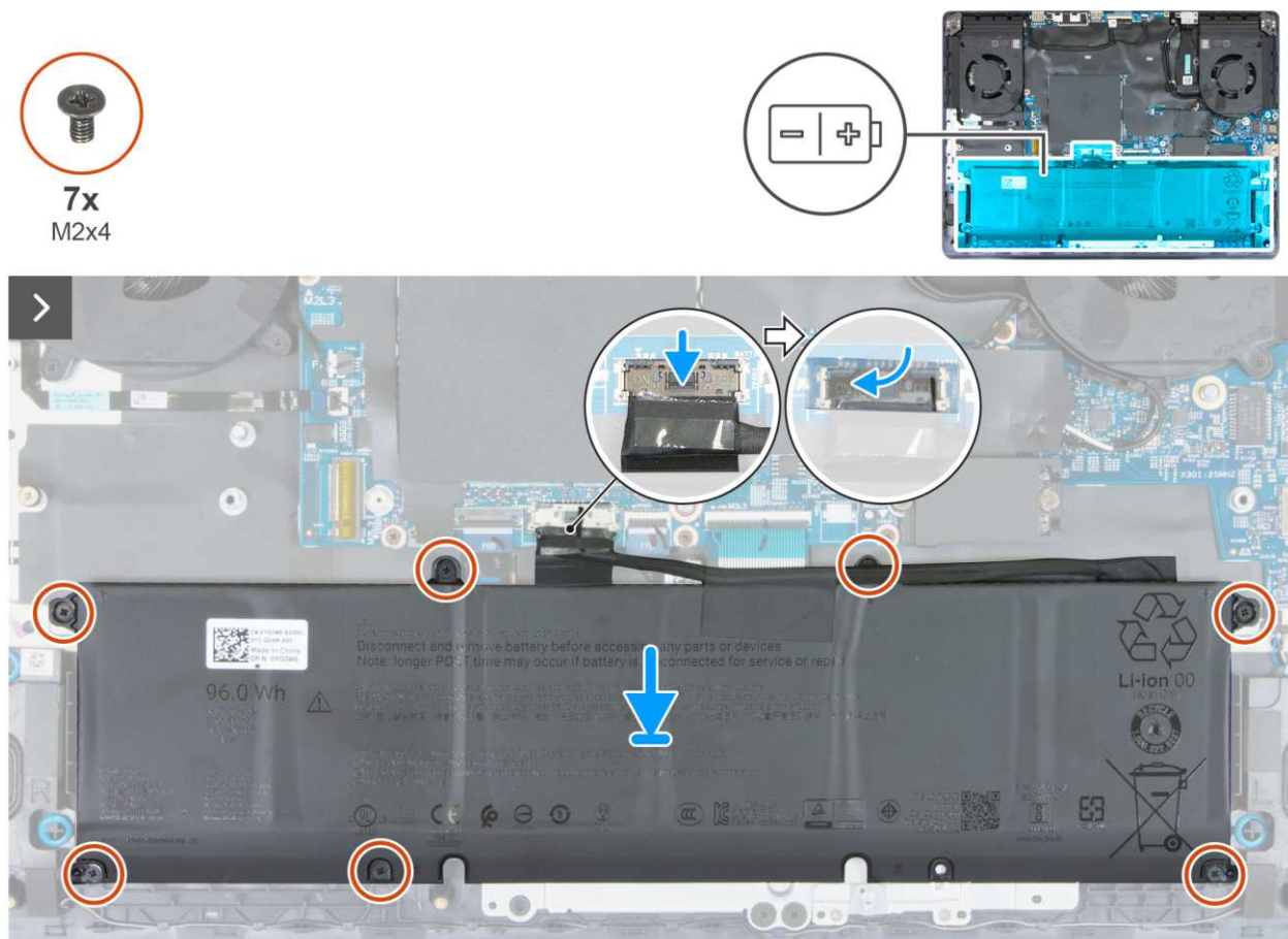
Rysunek 18. Instalowanie baterii
