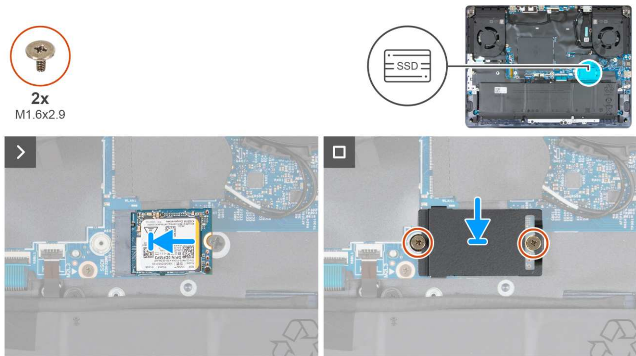
Rysunek 24. Instalacja dysku SSD M.2 2230 w gnieździe SSD1
