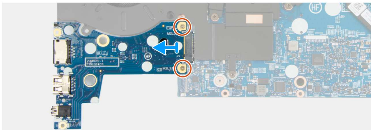
Rysunek 62. Wymontowywanie płyty we/wy
