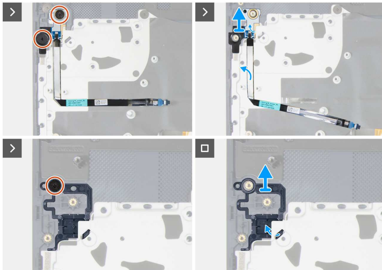
Rysunek 57. Wymontowywanie przycisku zasilania i płyty przycisku zasilania
