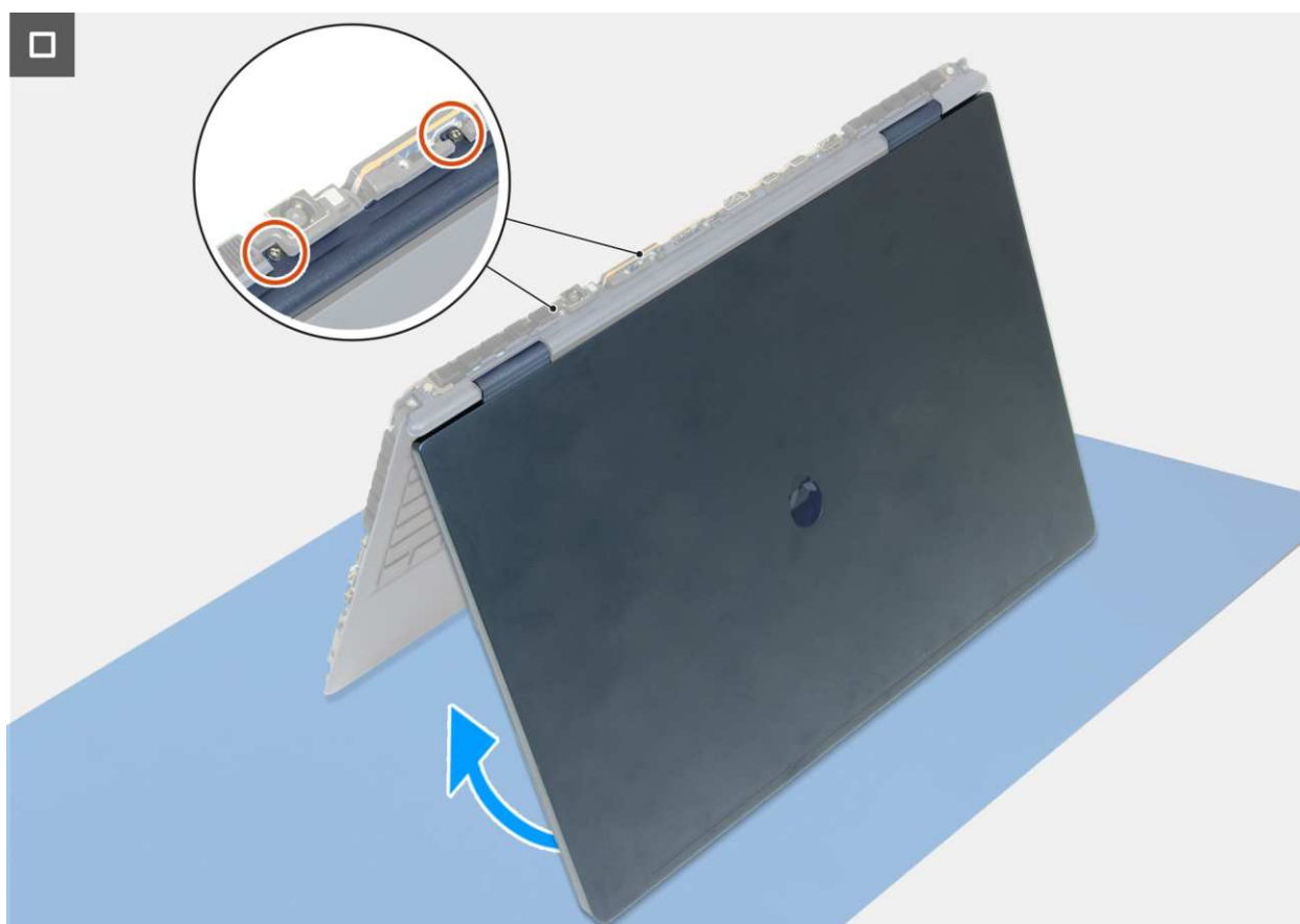
Rysunek 70. Instalacja listwy środkowej
