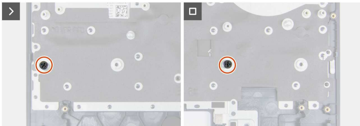
Rysunek 78. Wkręcanie uchwytów na śruby dysku SSD
