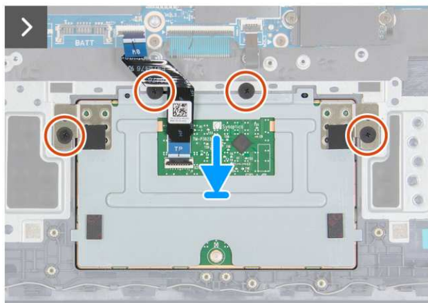
Rysunek 44. Instalowanie touchpada
