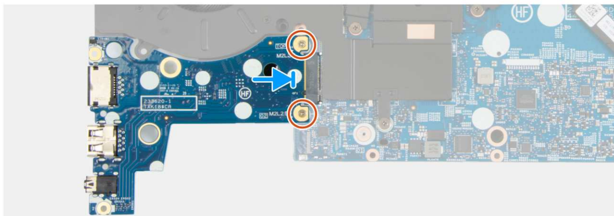
Rysunek 63. Instalowanie płyty we/wy
