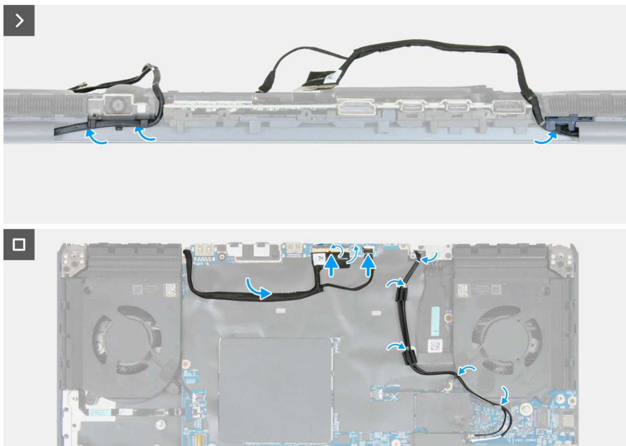
Rysunek 75. Instalowanie zestawu wyświetlacza
