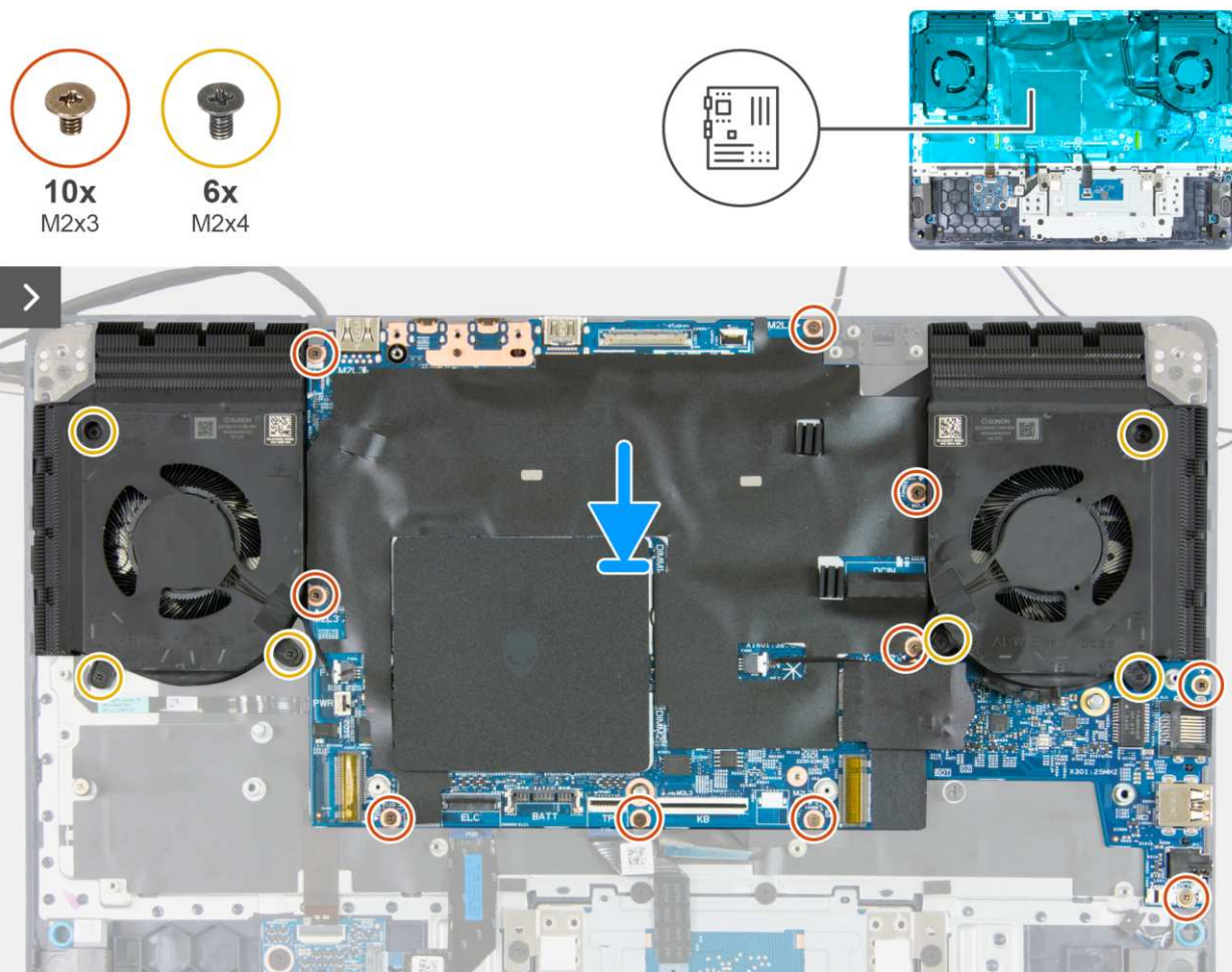
Rysunek 55. Instalowanie płyty głównej
