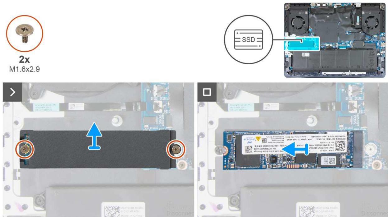
Rysunek 29. Wymontowywanie dysku SSD M.2 2280 z gniazda SSD2
