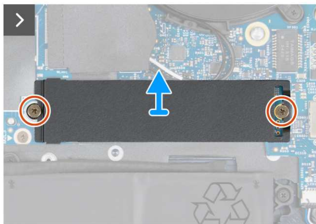
Rysunek 27. Wymontowywanie dysku SSD M.2 2280 z gniazda SSD1
