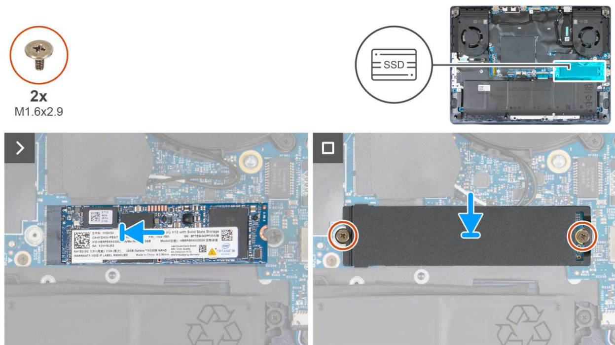
Rysunek 28. Instalacja dysku SSD M.2 2280 w gnieździe SSD1
