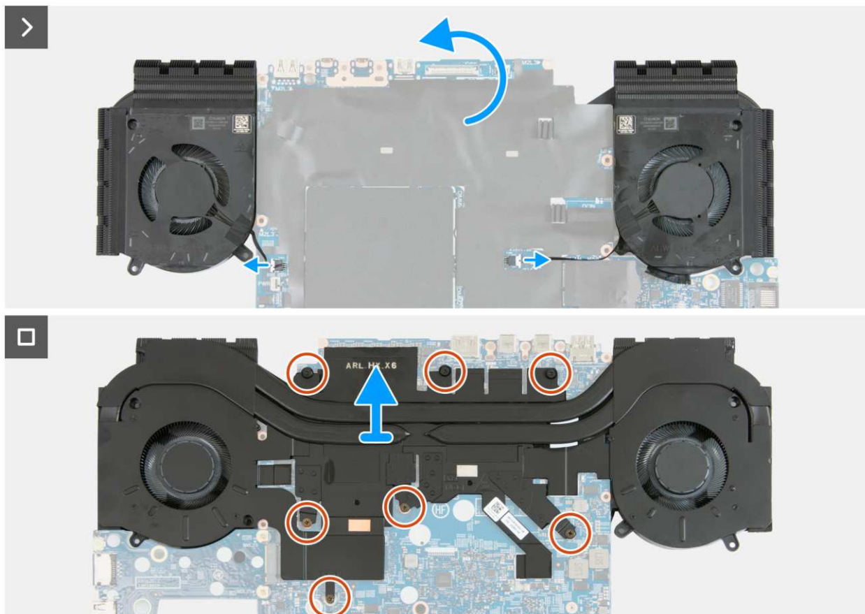
Rysunek 50. Wymontowywanie zestawu płyty głównej
