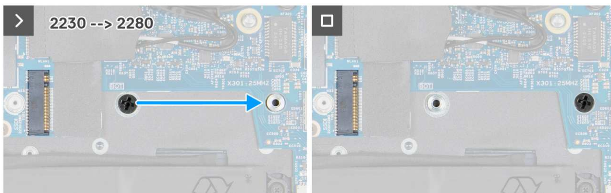
Rysunek 31. Procedura przenoszenia uchwyty śruby w celu zainstalowania dysku M2.2280
