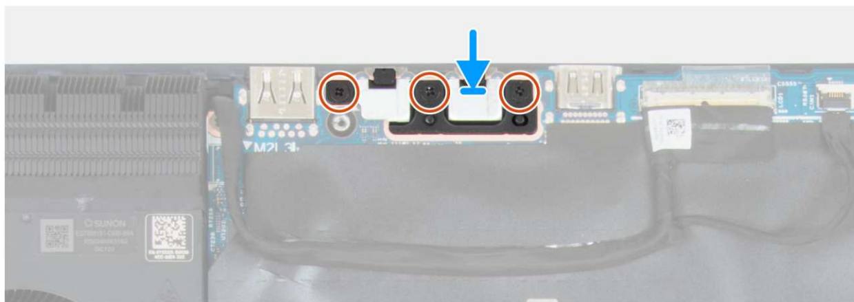
Rysunek 40. Instalowanie klamry złącza Type-C
