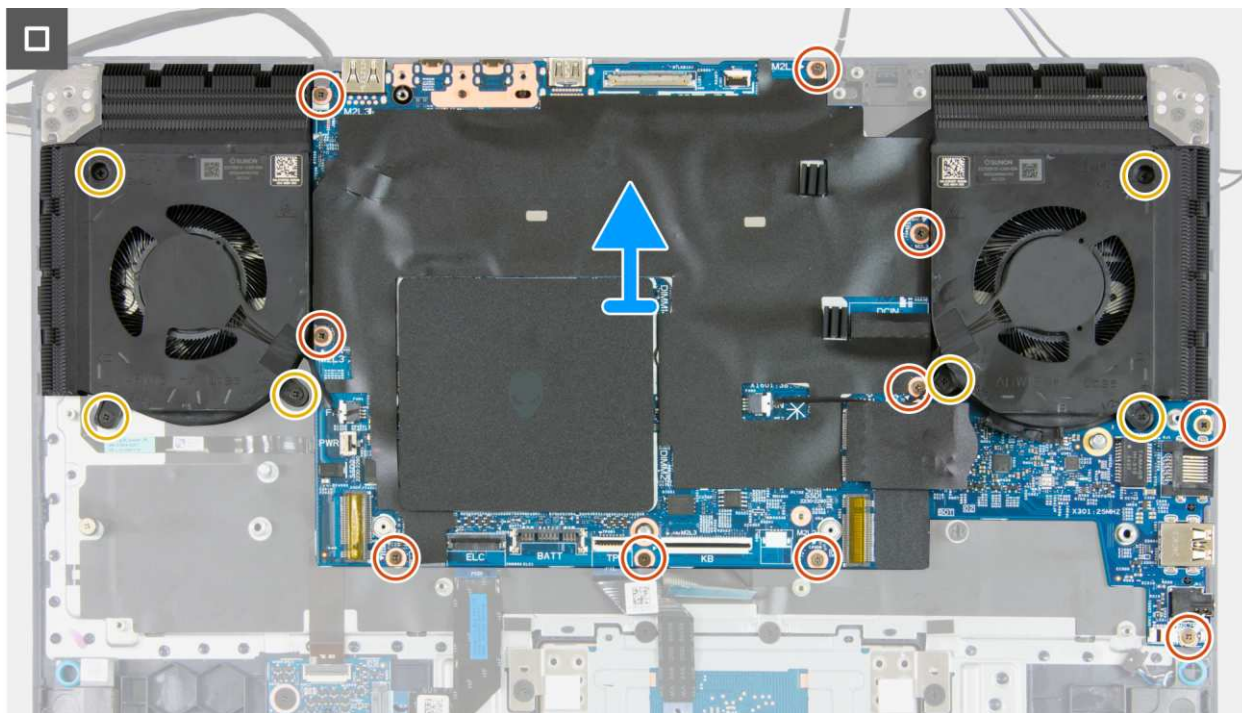
Rysunek 49. Wymontowywanie płyty głównej
