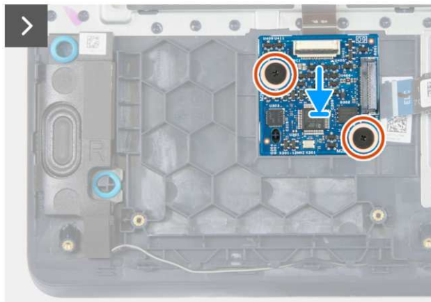
Rysunek 46. Instalowanie płyty kontrolera podświetlenia klawiatury (ELC)
