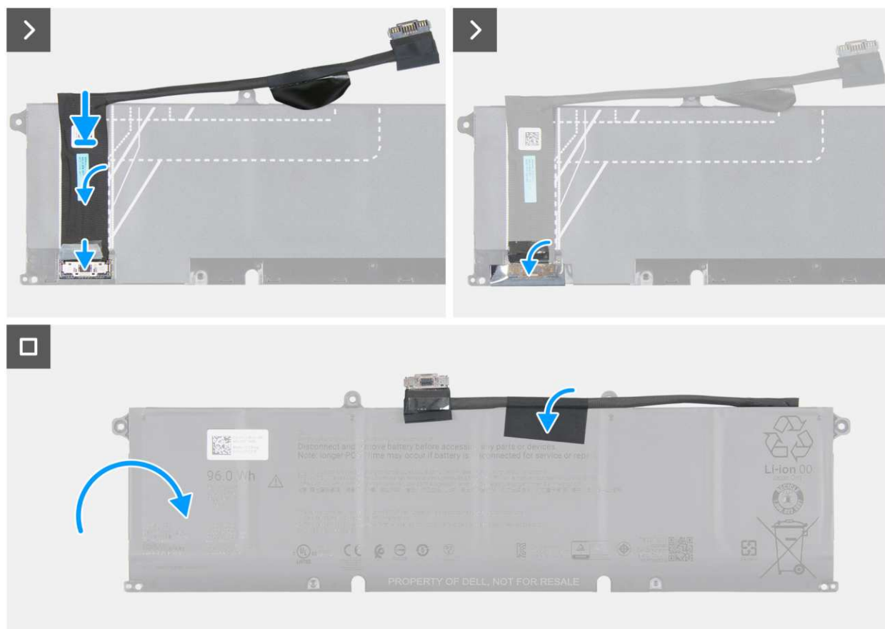
Rysunek 20. Instalacja kabla baterii
