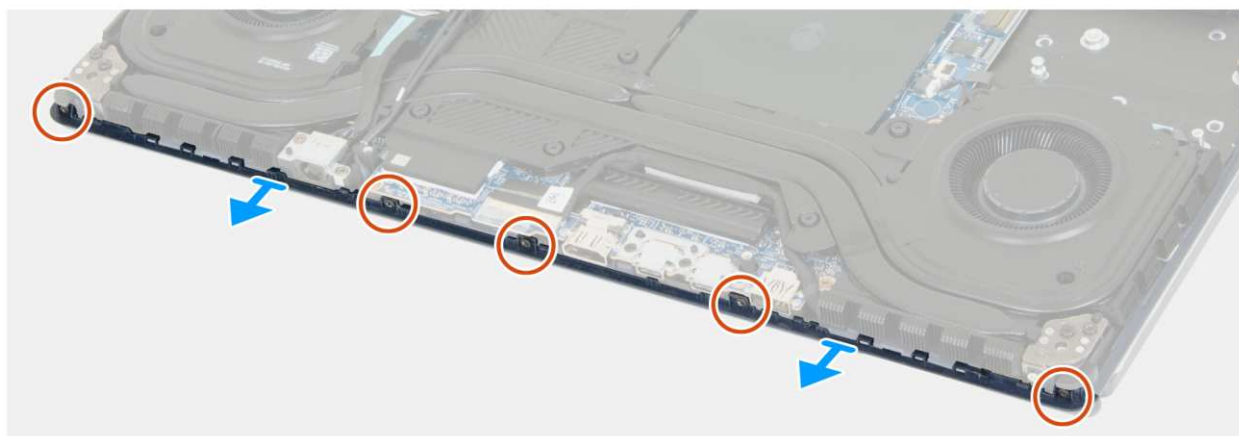
Rysunek 64. Wymontowywanie pokrywy tylnej
