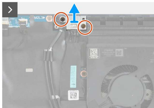
Rysunek 37. Wymontowywanie gniazda zasilacza
