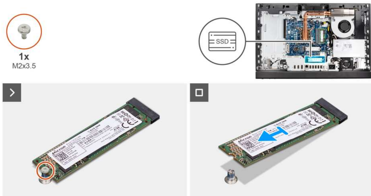
Rysunek 38. Wymontowywanie dysku SSD M.2 2280 z gniazda M.2 nr 1
