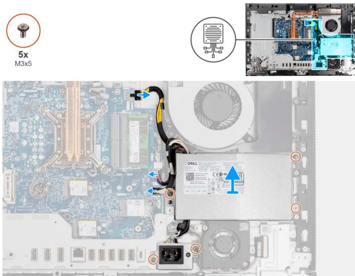
Rysunek 51. Wymontowywanie zasilacza
