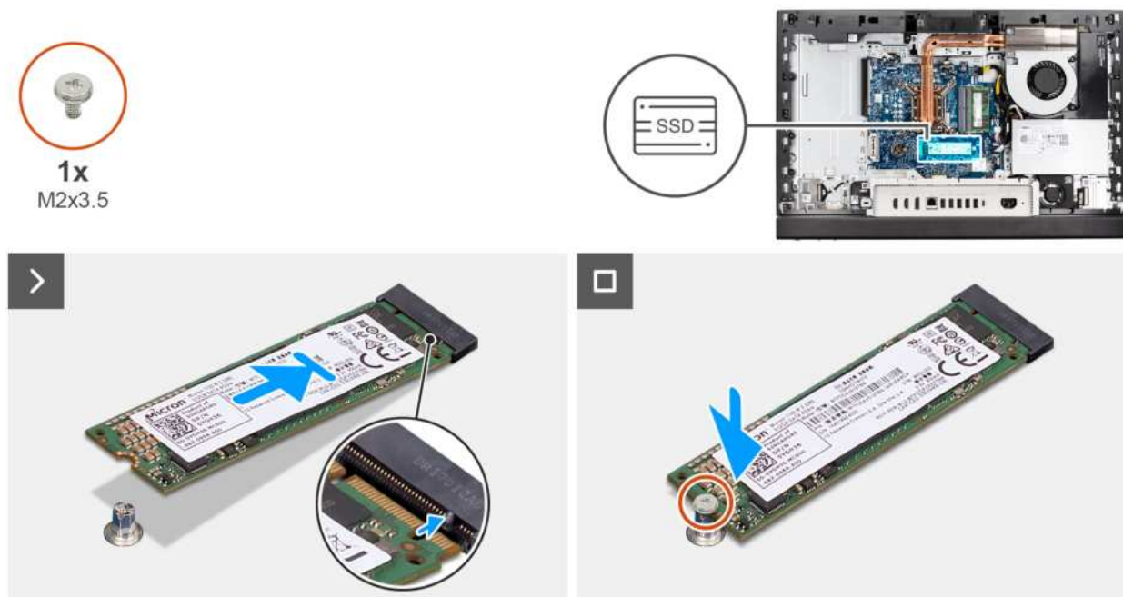
Rysunek 34. Instalowanie dysku SSD M.2 2280 w gnieździe M.2 nr 0
