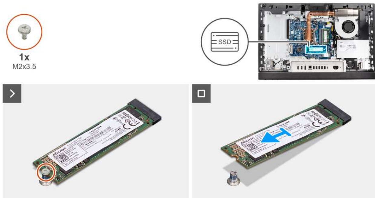
Rysunek 33. Wymontowywanie dysku SSD M.2 2280 z gniazda M.2 nr 0
