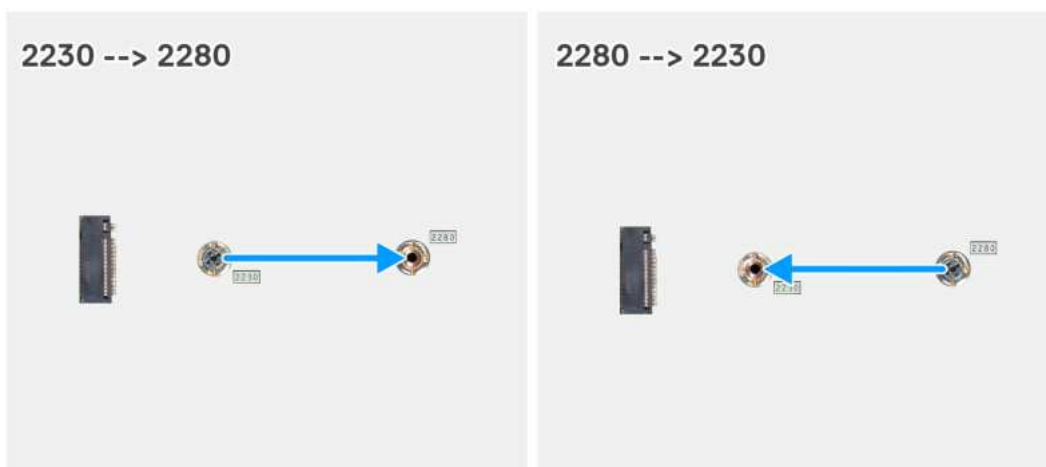
Rysunek 35. Przenoszenie uchwytu na śrubę w gnieździe SSD M.2 nr 0
