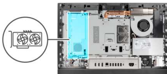
Rysunek 23. Wymontowywanie zestawu karty graficznej (model z ekranem dotykowym)
