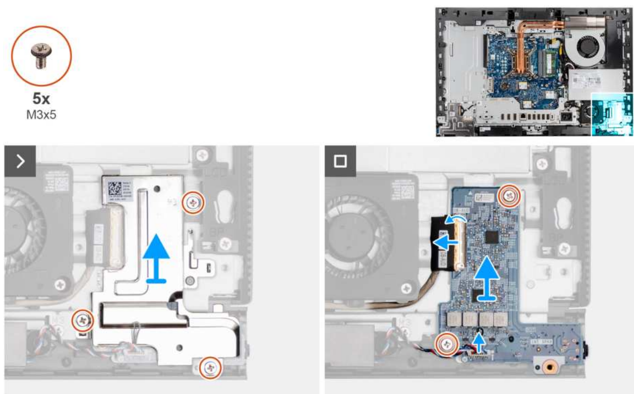
Rysunek 71. Wymontowywanie karty dźwiękowej
