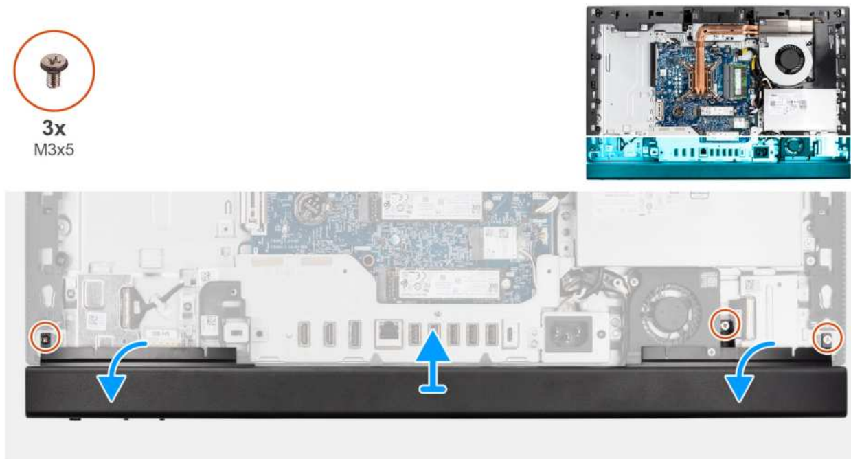
Rysunek 45. Wymontowywanie pokrywy dolnej
