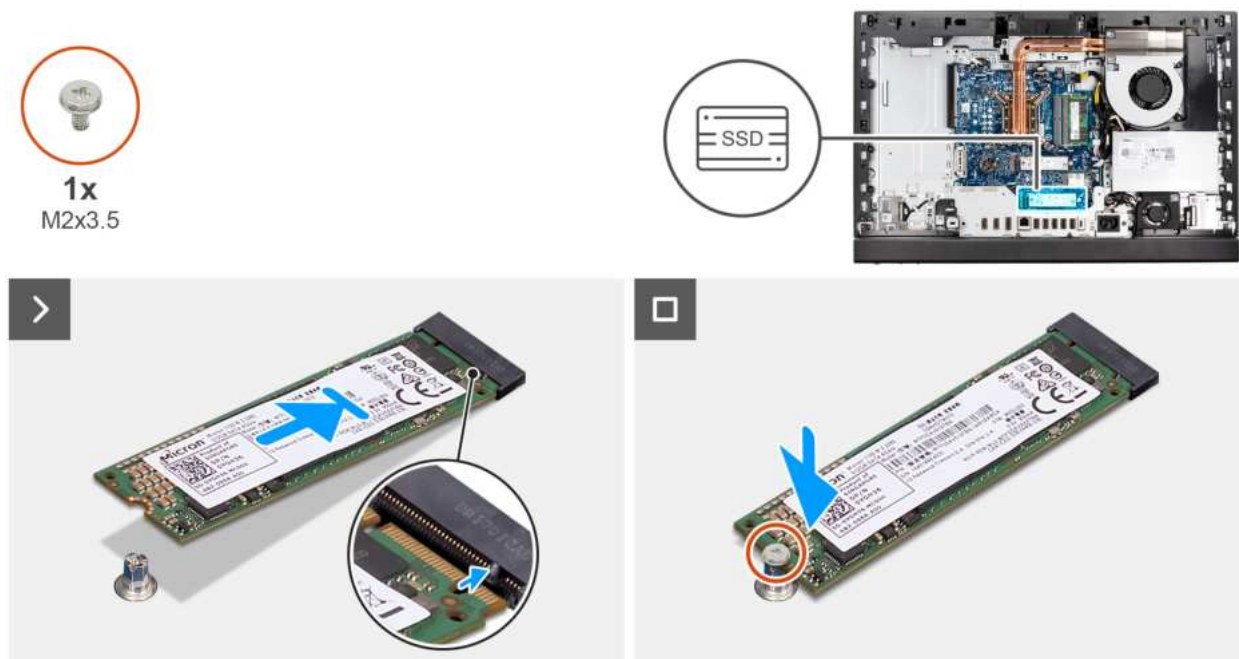
Rysunek 39. Instalowanie dysku SSD M.2 2280 w gnieździe M.2 nr 1
