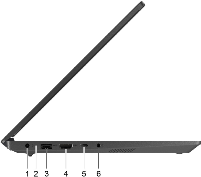
Rysunek 6. Widok z lewej strony—modele 14-calowe
