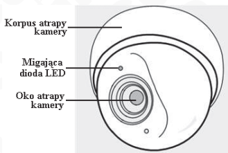
Rys. 1. Budowa atrapy kamery monitorującej AK-02B3
