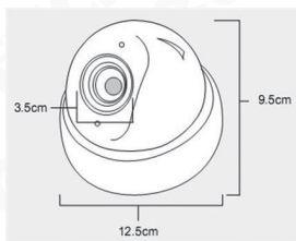
Rys. 2. Wymiary zewnętrzne atrapy AK-02B3
