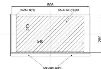
Rys.4: Przygotowanie szafki
