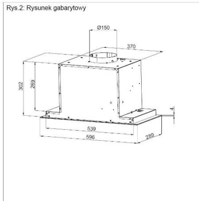
Rys. 2: Rysunek gabarytowy
