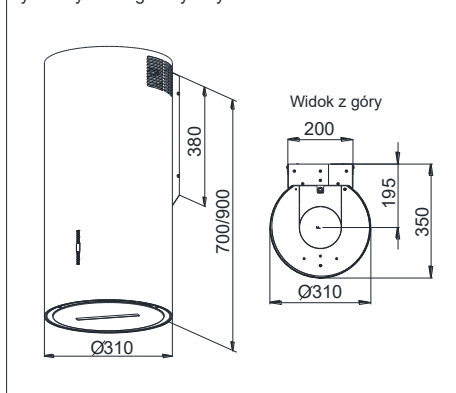
Rys. 2 Rysunek gabarytowy.
