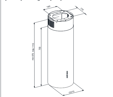
Rys. 2 Rysunek gabarytowy.
