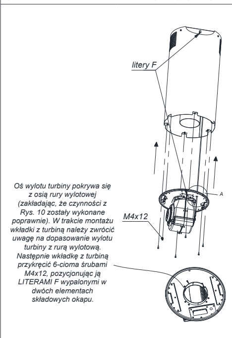
Rys.13 Mocowanie okapu do sufitu. Montaż turbiny do rury wylotowej.
