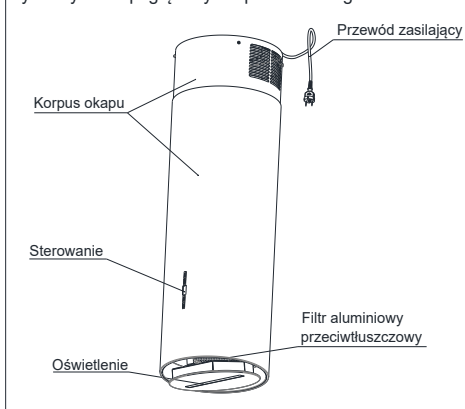
Rys.1 Rysunek poglądowy okapu kuchennego.
