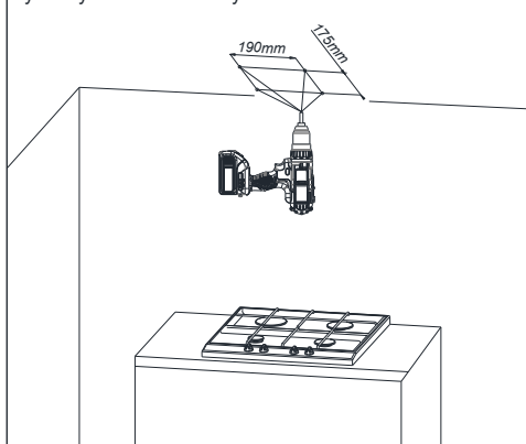
Rys.4 Rysunek montażowy do sufitu.
