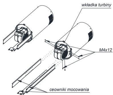
Rys. 7 Demontaż wsporników.
