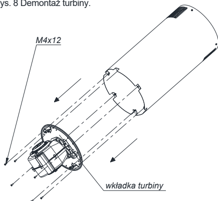
Rys. 8 Demontaż turbiny.
