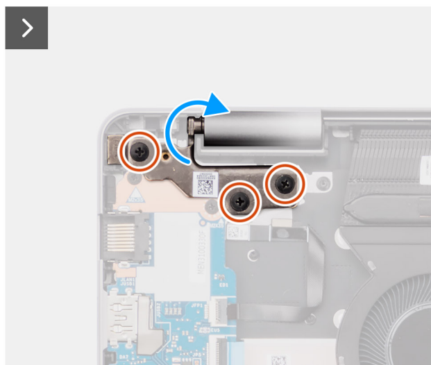
Rysunek 47. Wymontowywanie zestawu wyświetlacza
