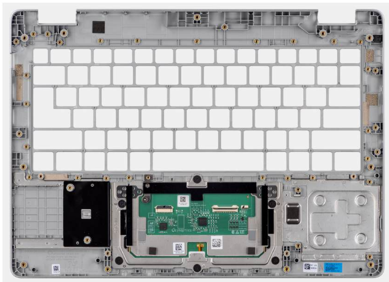
Rysunek 98. Instalowanie zestawu podpórki na nadgarstek
