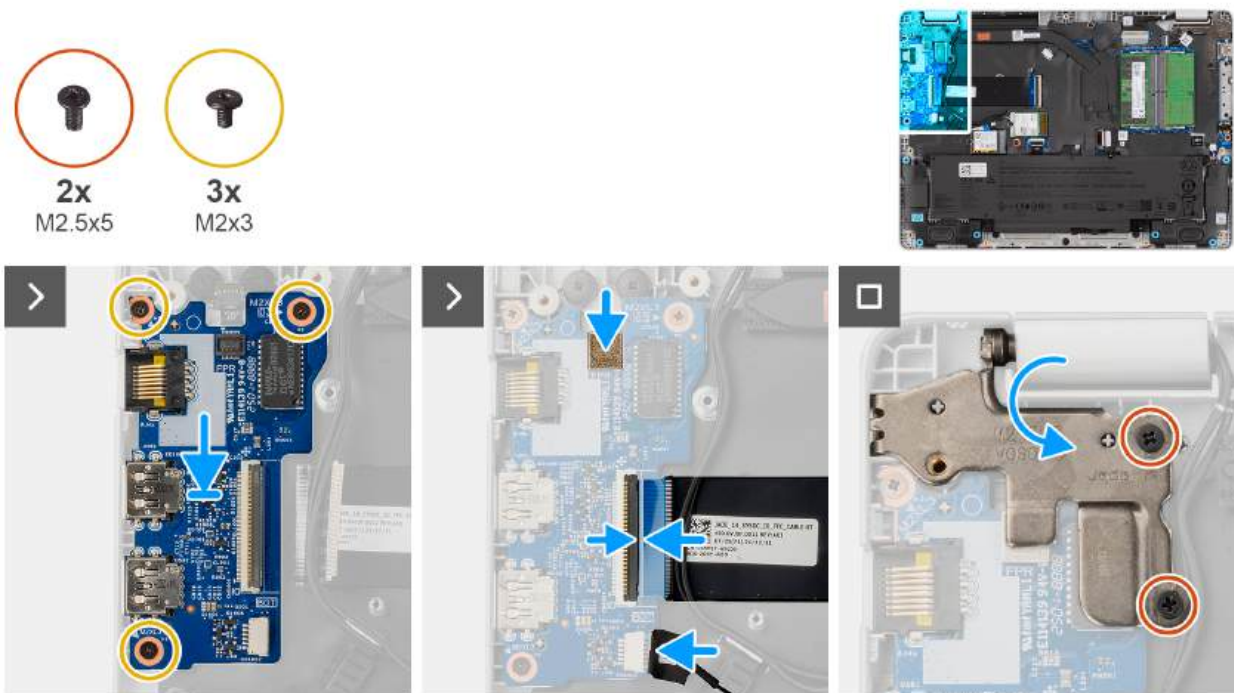
Rysunek 52. Instalowanie płyty we/wy
