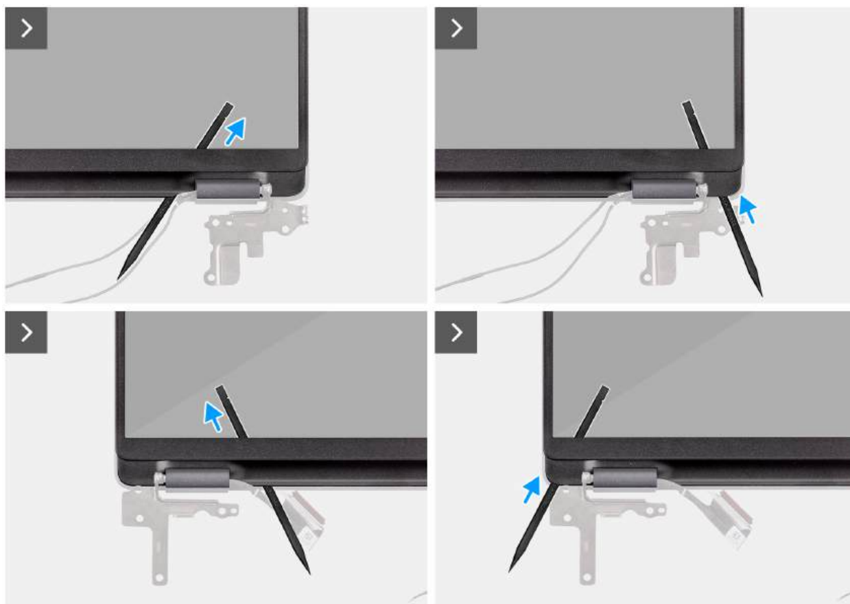
Rysunek 106. Wymontowywanie ramki wyświetlacza
