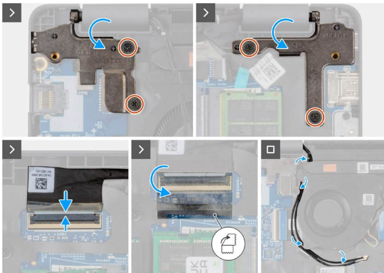
Rysunek 103. Instalowanie zestawu wyświetlacza
