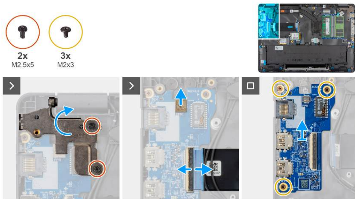
Rysunek 49. Wymontowywanie płyty we/wy
