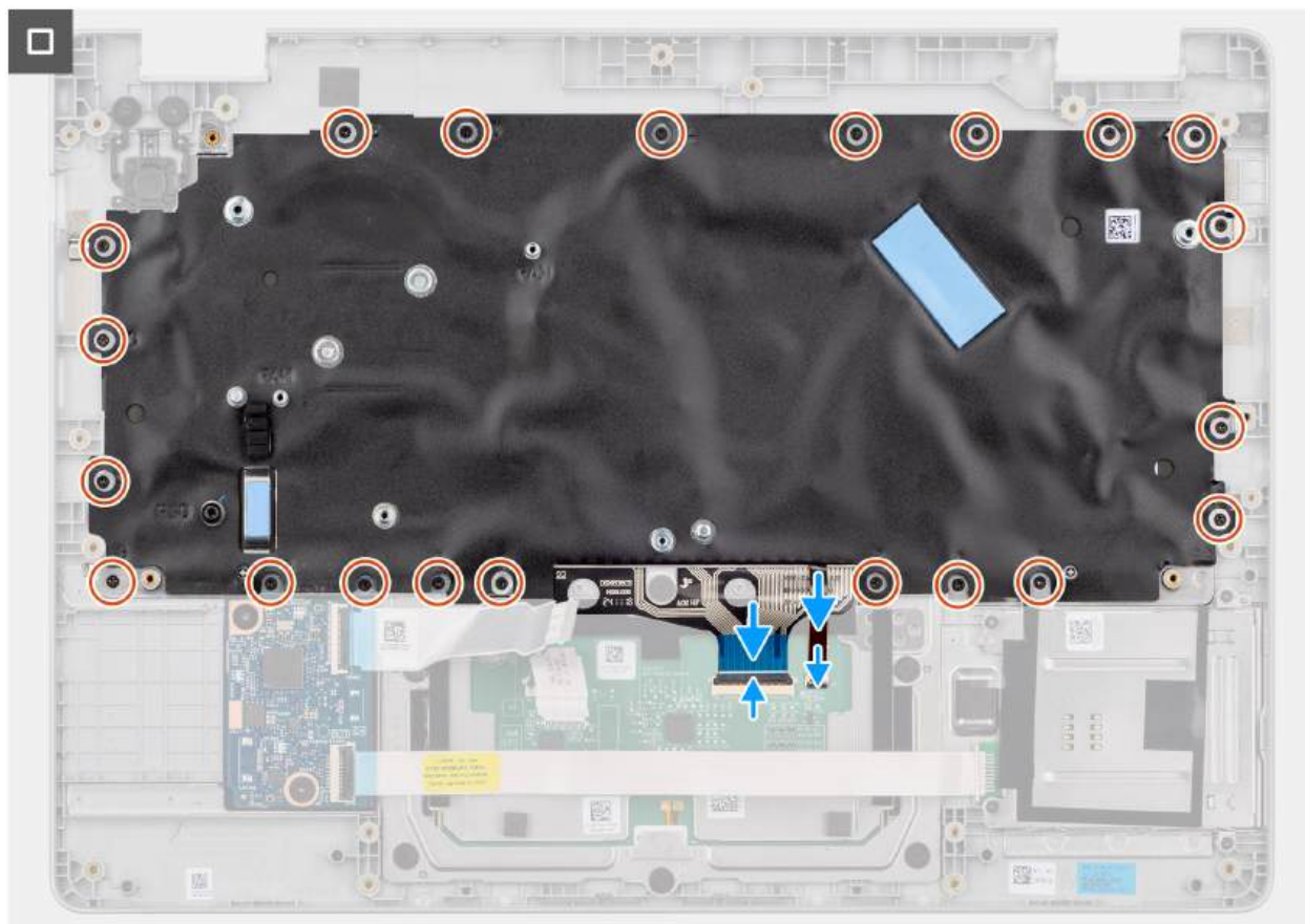
Rysunek 90. Instalowanie klawiatury
