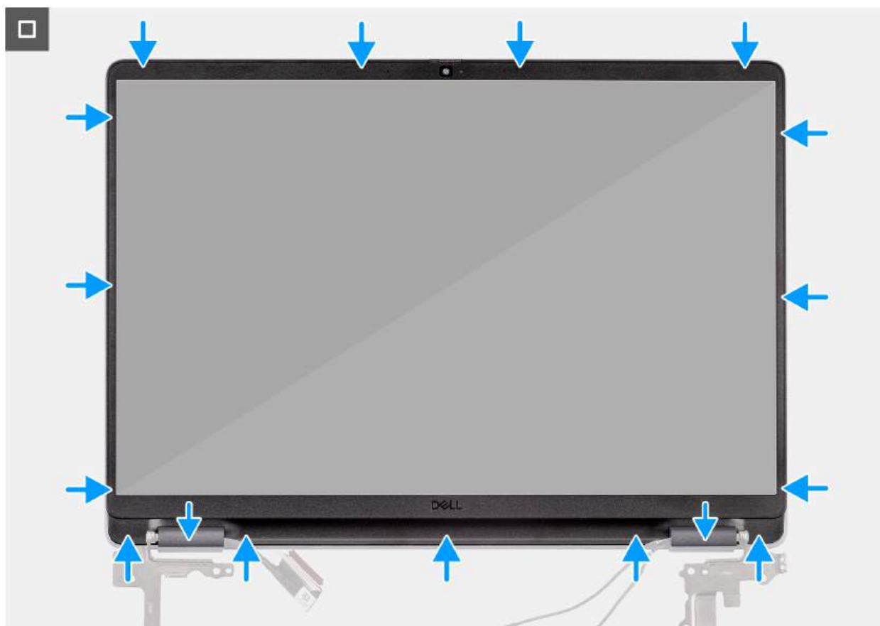
Rysunek 110. Instalowanie ramki wyświetlacza
