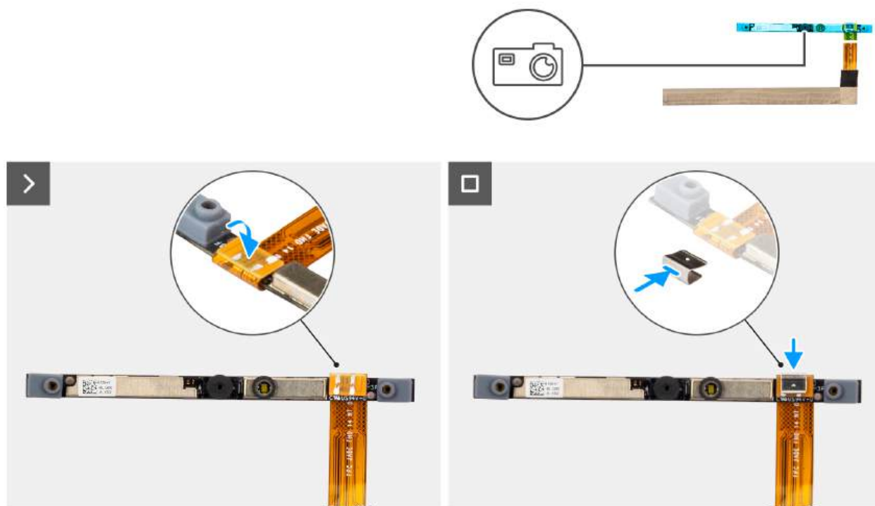
Rysunek 120. Instalowanie kamery
