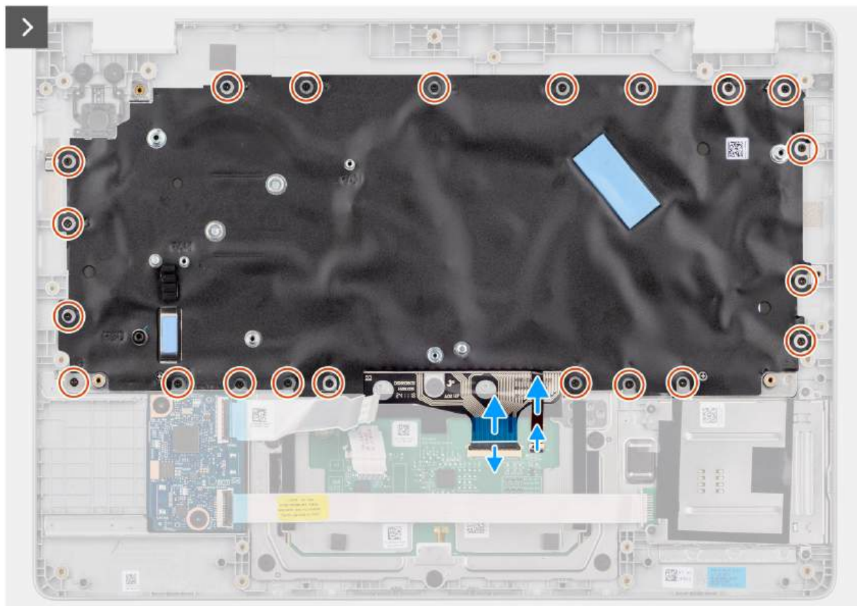
Rysunek 85. Wymontowywanie klawiatury
