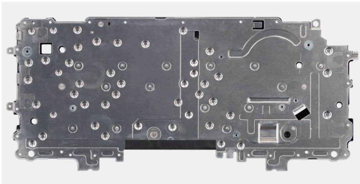
Rysunek 93. Instalowanie płyty nośnej klawiatury
