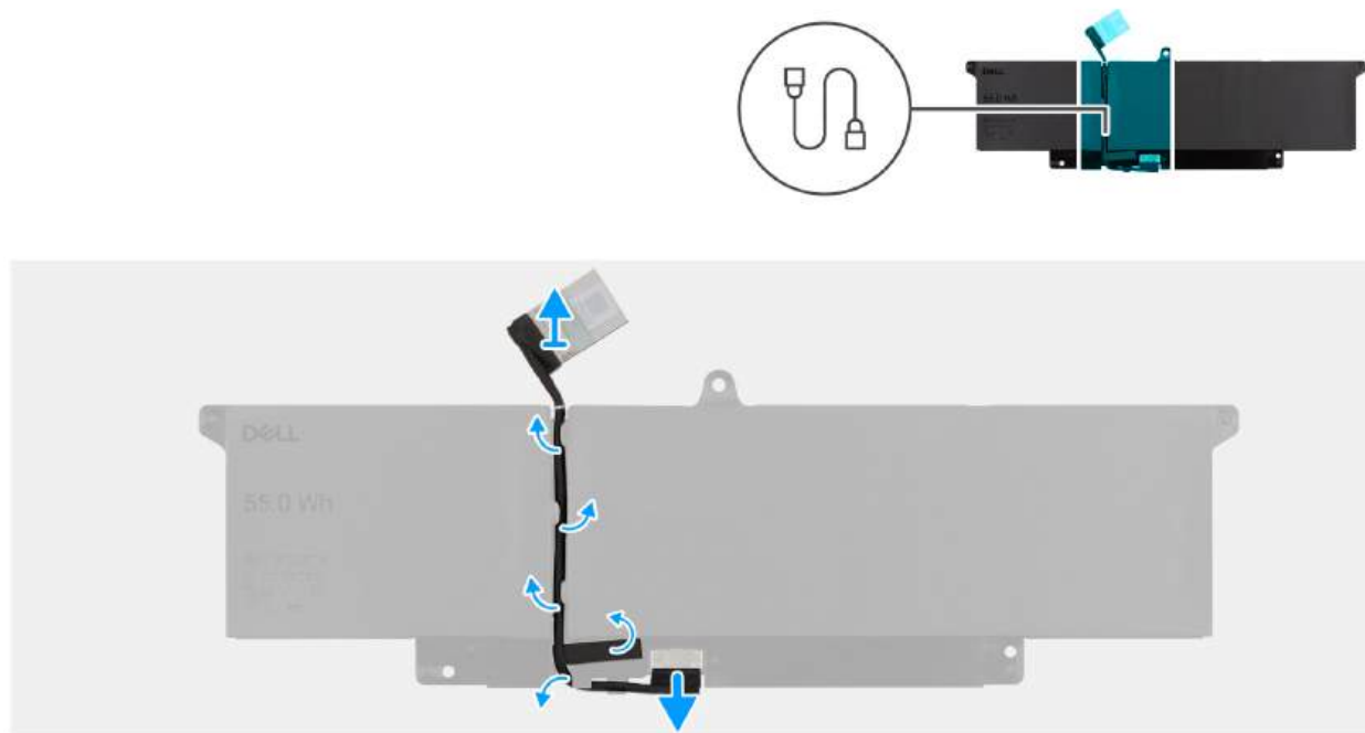
Rysunek 19. Wymontowywanie kabla baterii
