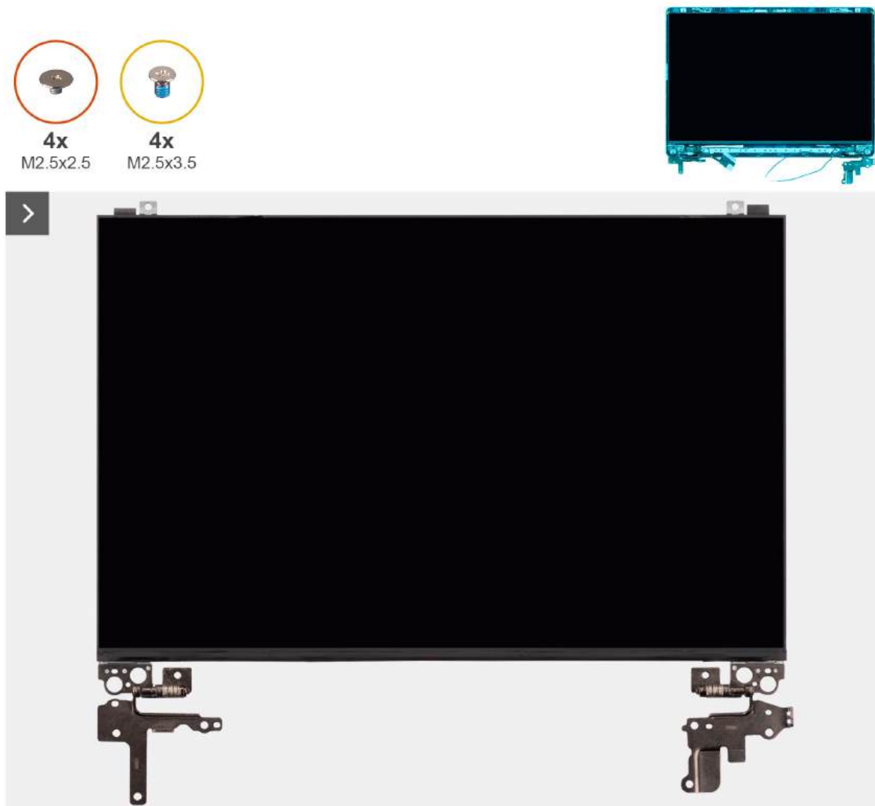
Rysunek 115. Instalowanie zestawu panelu wyświetlacza
