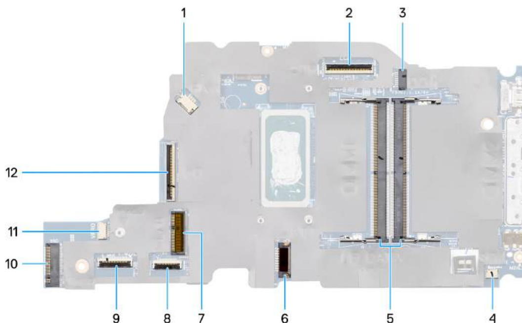
Rysunek 69. Złącza płyty głównej
