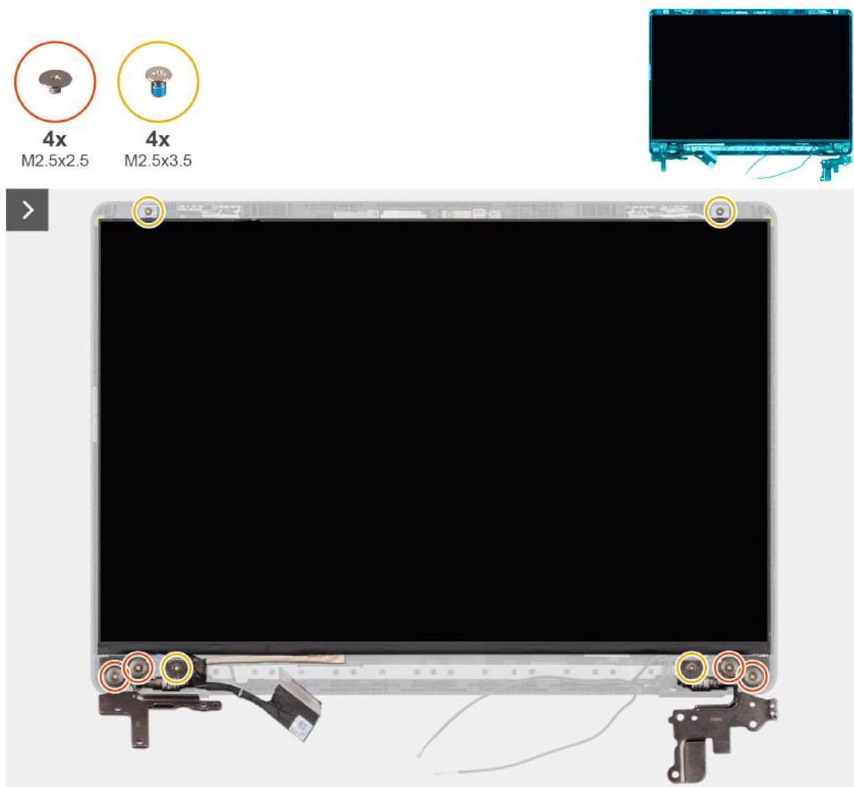
Rysunek 111. Wymontowywanie zestawu panelu wyświetlacza
