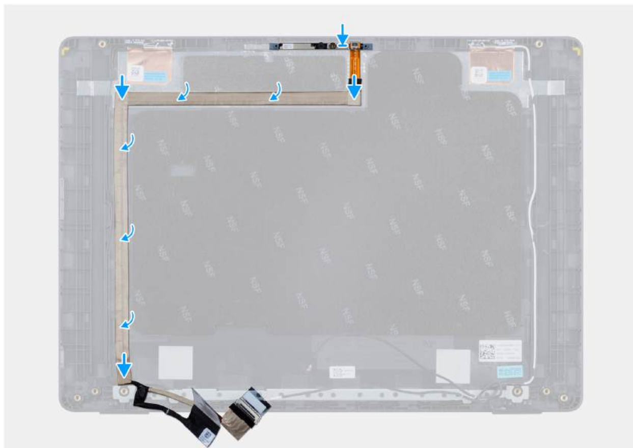
Rysunek 122. Instalowanie kabla eDP
