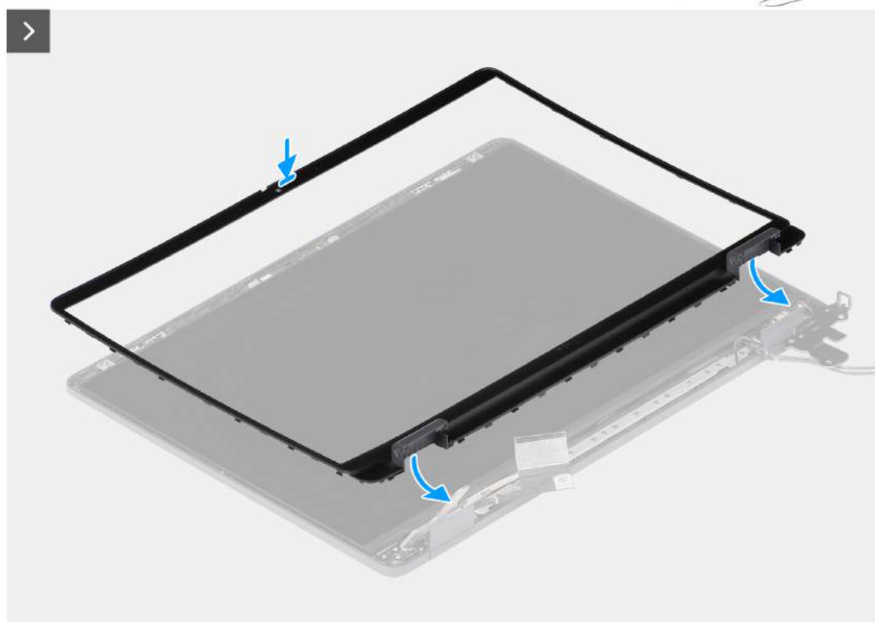
Rysunek 109. Instalowanie ramki wyświetlacza
