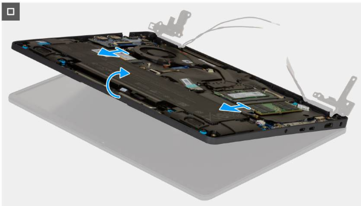
Rysunek 100. Wymontowywanie zestawu wyświetlacza
