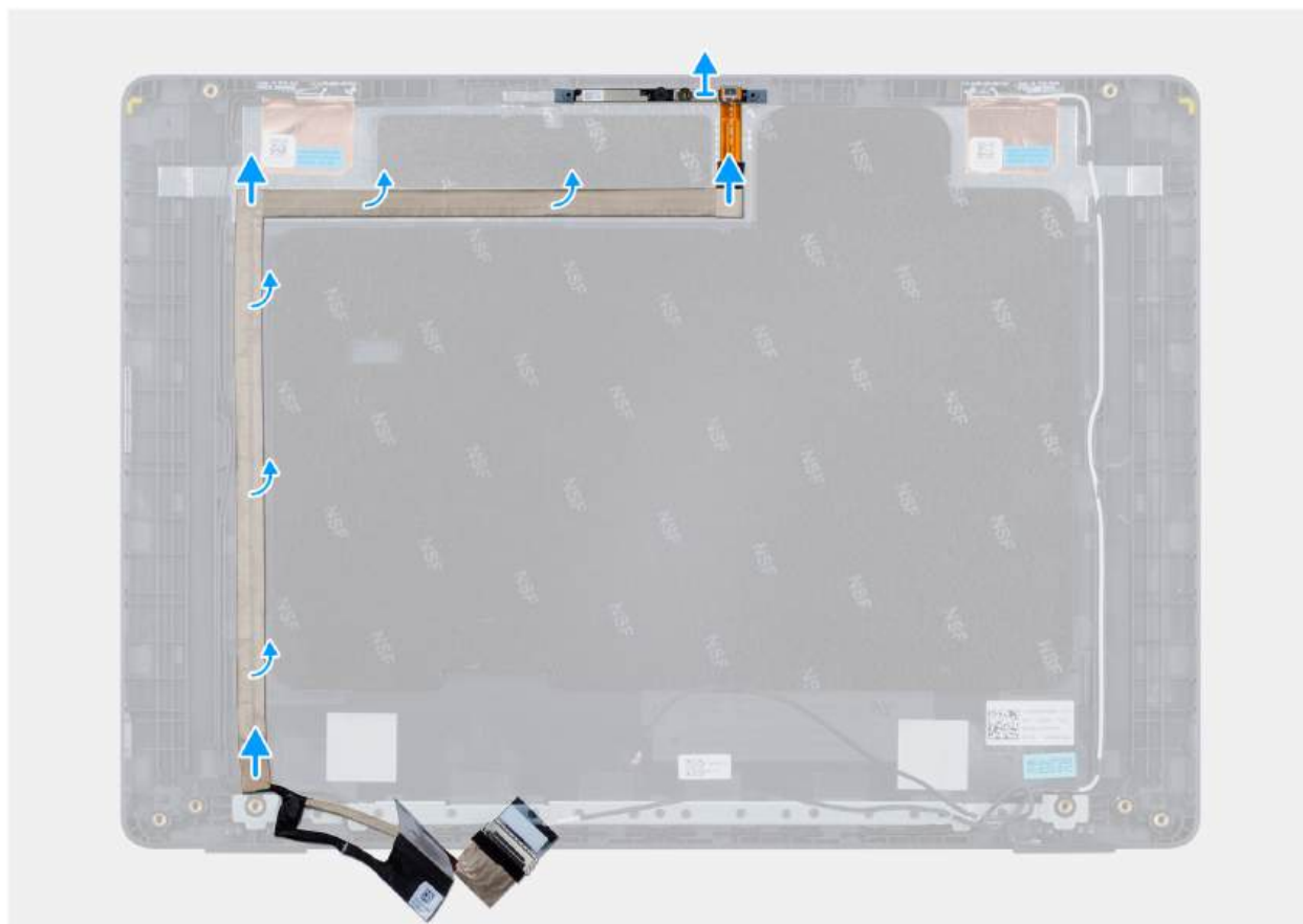
Rysunek 121. Wymontowywanie kabla eDP
