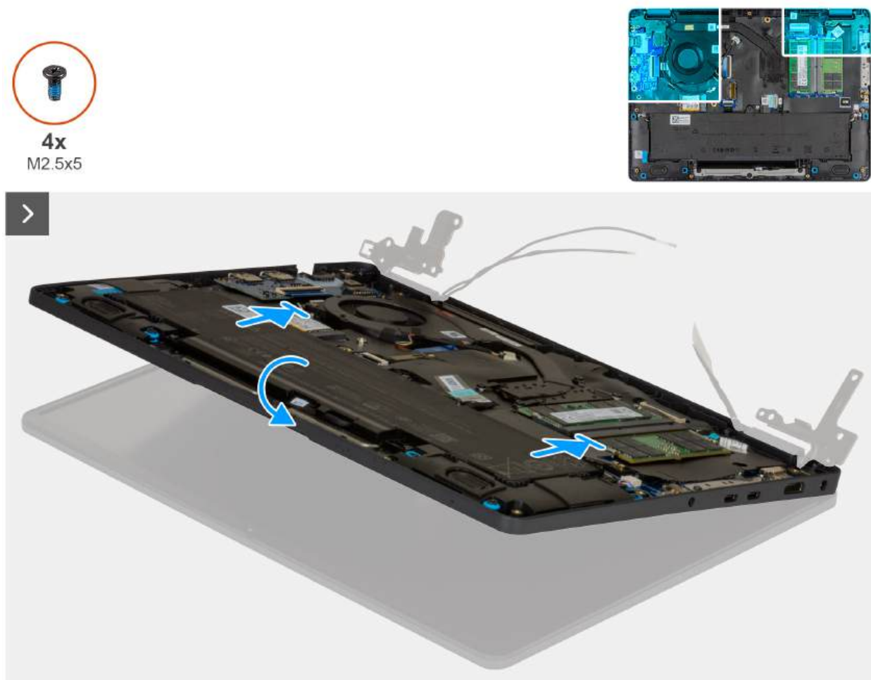
Rysunek 102. Instalowanie zestawu wyświetlacza
