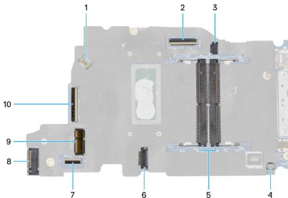
Rysunek 60. Złącza płyty głównej
