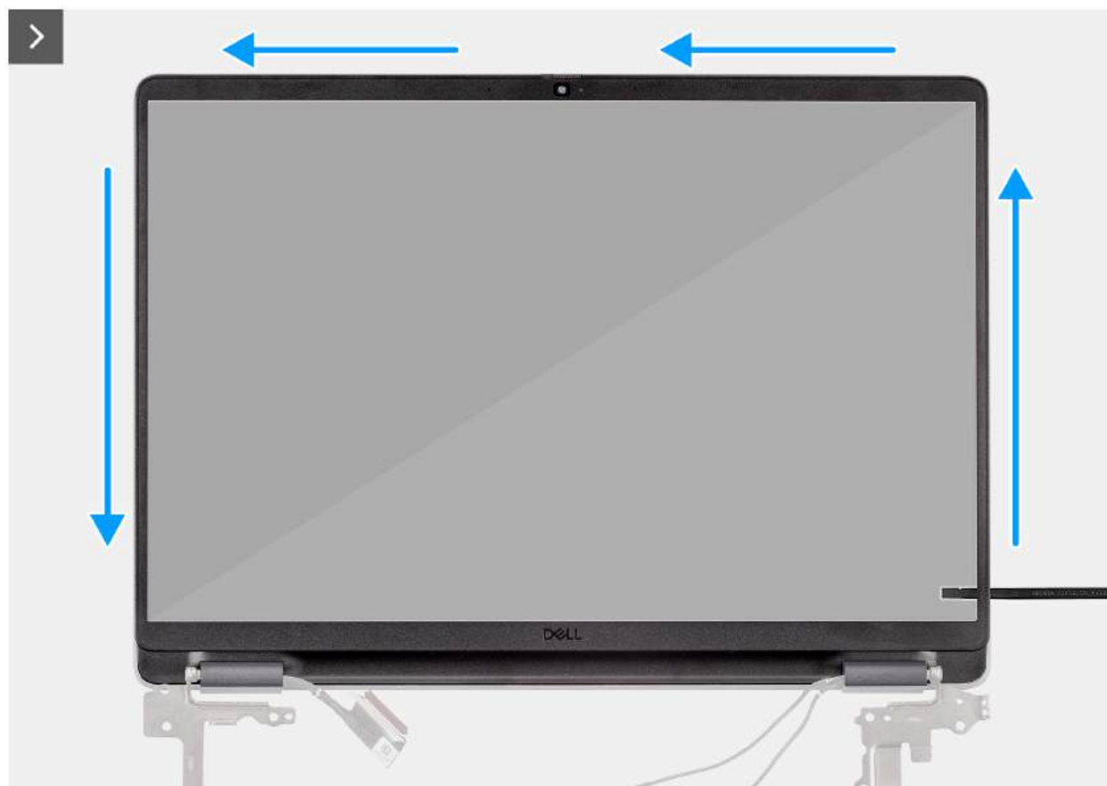
Rysunek 107. Wymontowywanie ramki wyświetlacza
