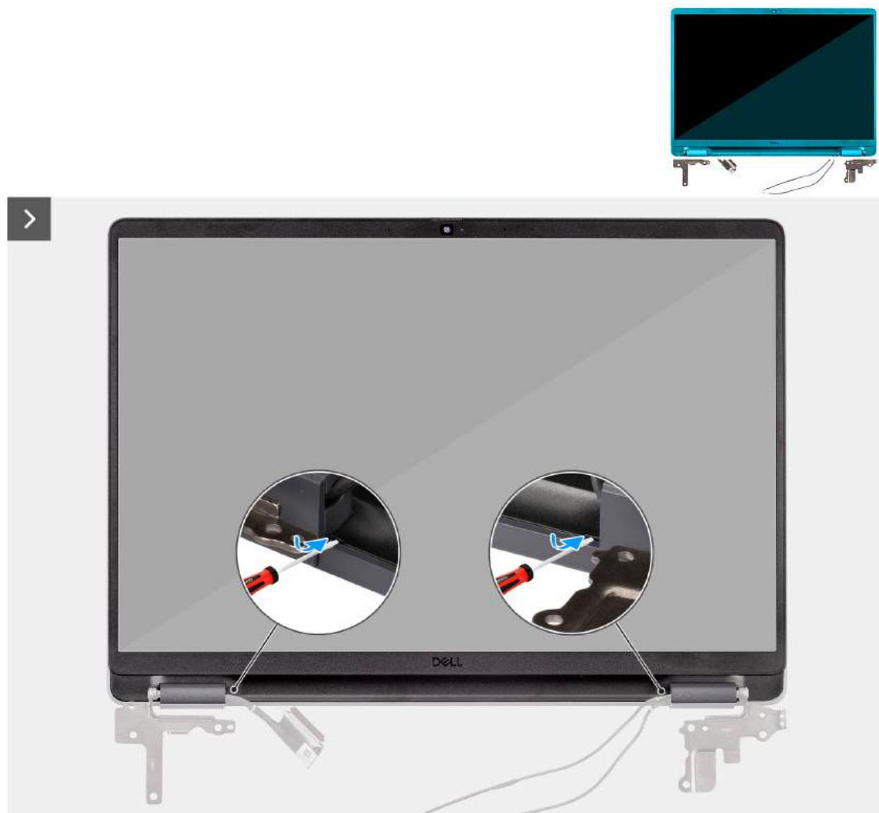
Rysunek 104. Wymontowywanie ramki wyświetlacza
