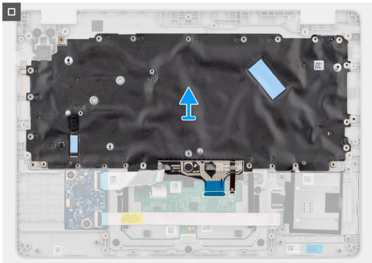
Rysunek 86. Wymontowywanie klawiatury
