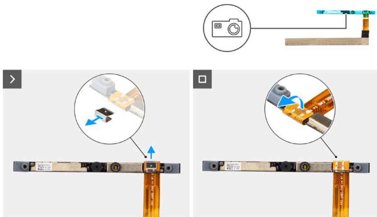
Rysunek 119. Wymontowywanie kamery
