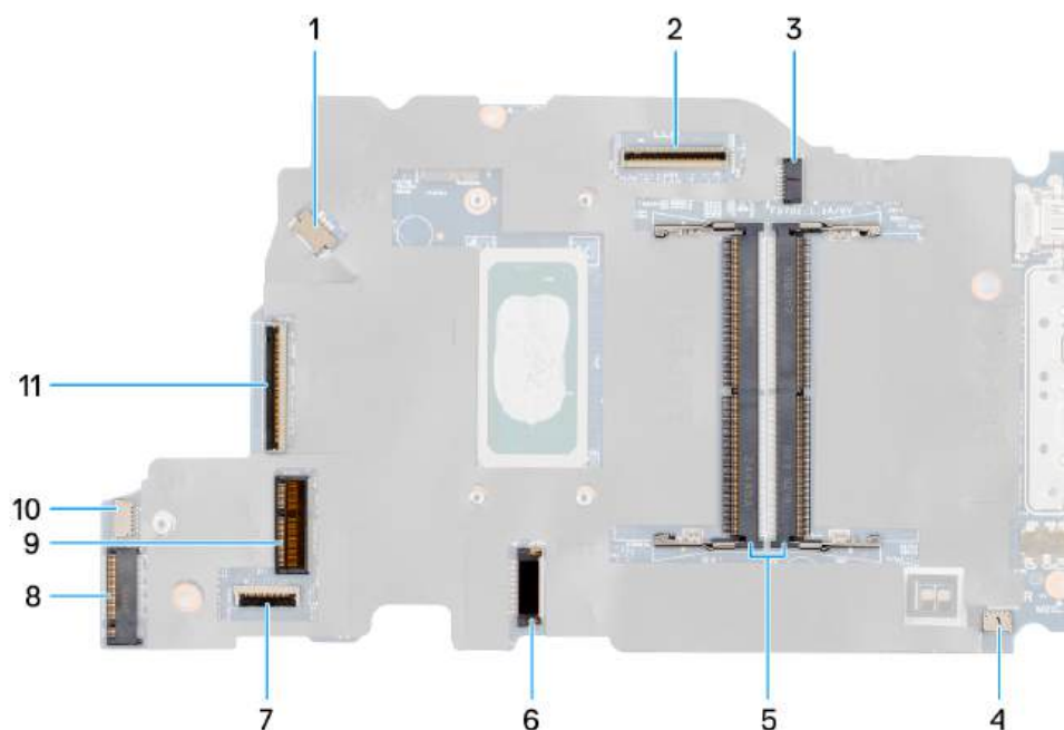
Rysunek 63. Złącza płyty głównej
