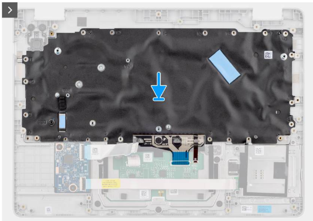
Rysunek 89. Instalowanie klawiatury
