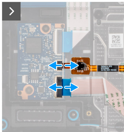
Rysunek 43. Wymontowywanie karty USH
