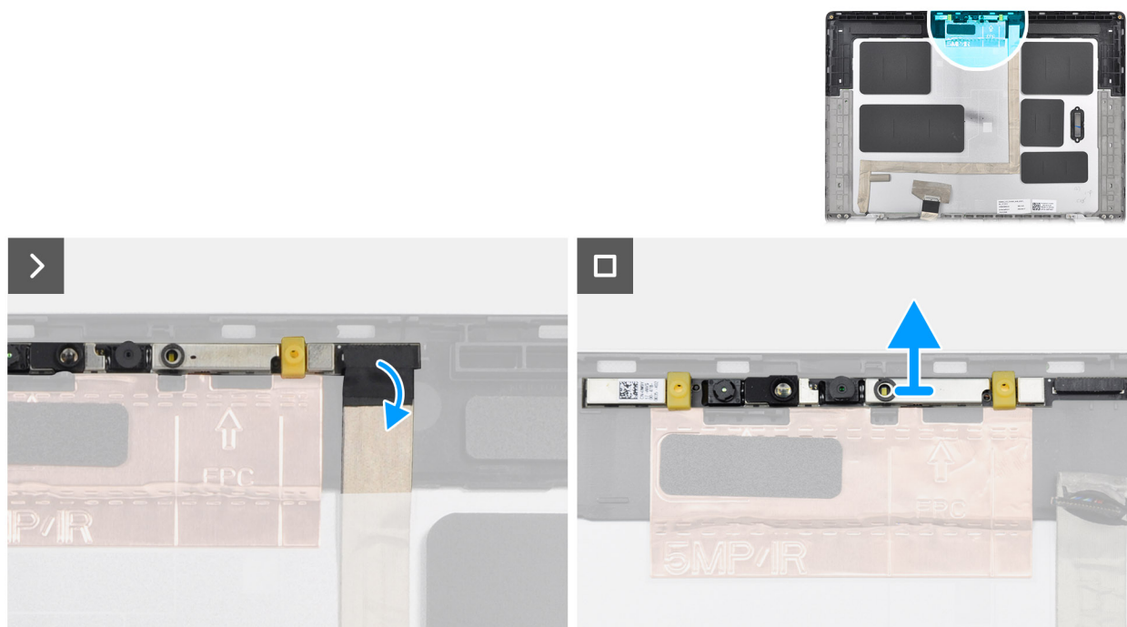
Rysunek 75. Wymontowywanie kamery RGB/IR
