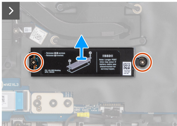
Rysunek 35. Wymontowywanie dysku SSD M.2 2280
