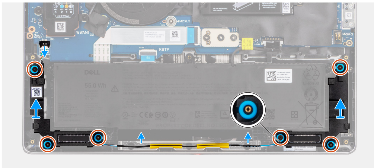
Rysunek 37. Wymontowywanie głośników
