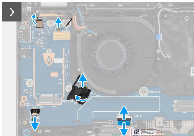
Rysunek 53. Wymontowywanie płyty we/wy
