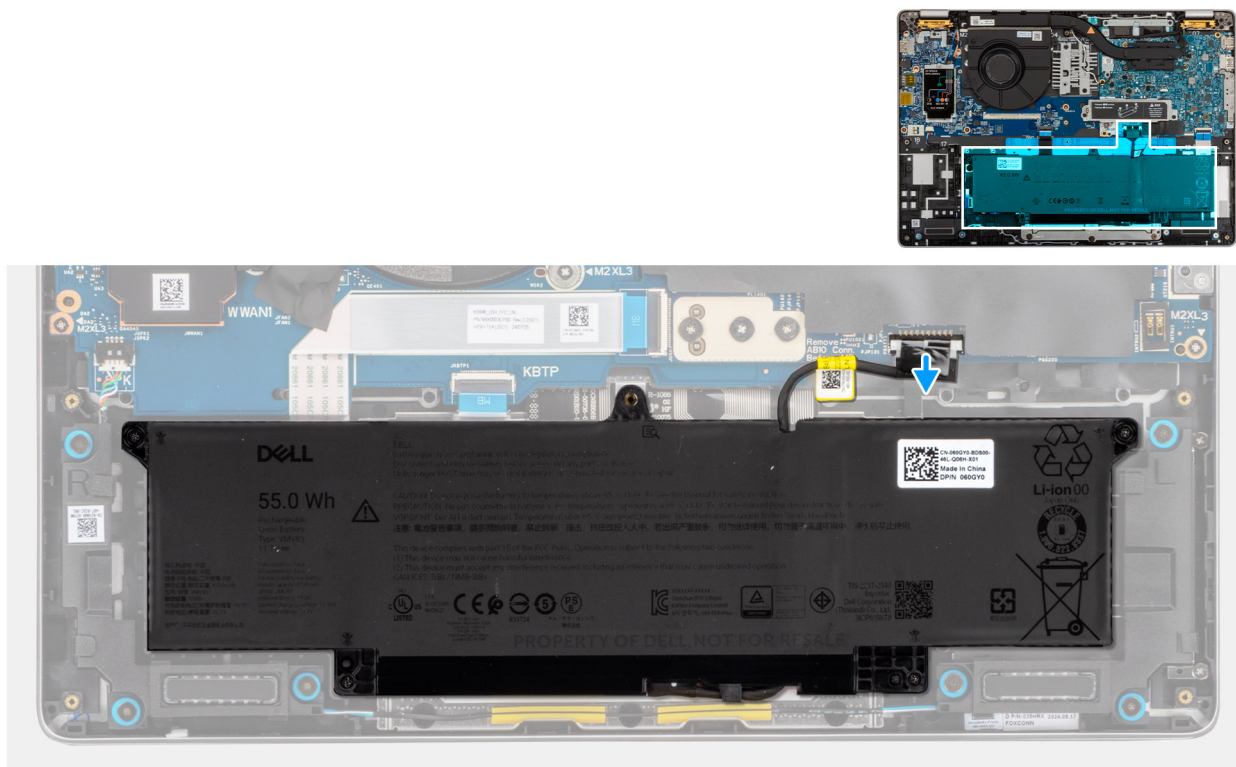
Rysunek 24. Odłączanie kabla baterii
