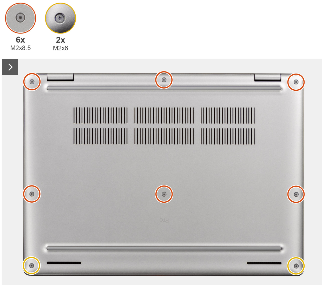
Rysunek 22. Wymontowywanie pokrywy dolnej
