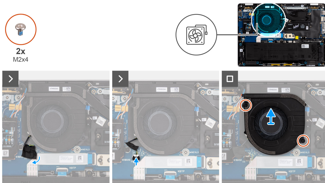
Rysunek 39. Wymontowywanie wentylatora
