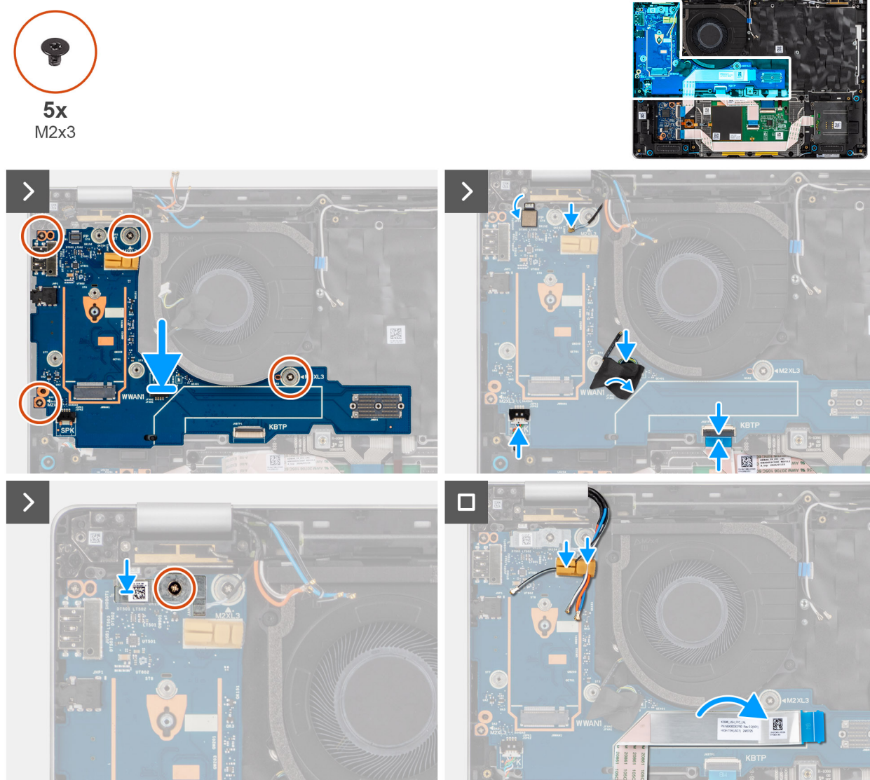
Rysunek 54. Instalowanie płyty we/wy
