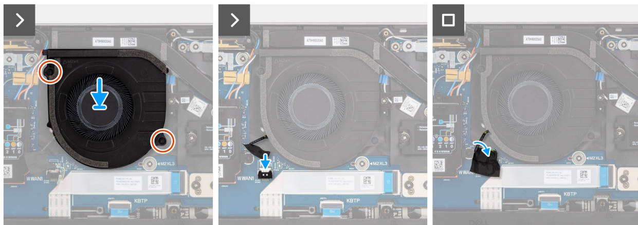
Rysunek 40. Sprzedaż wentylatora
