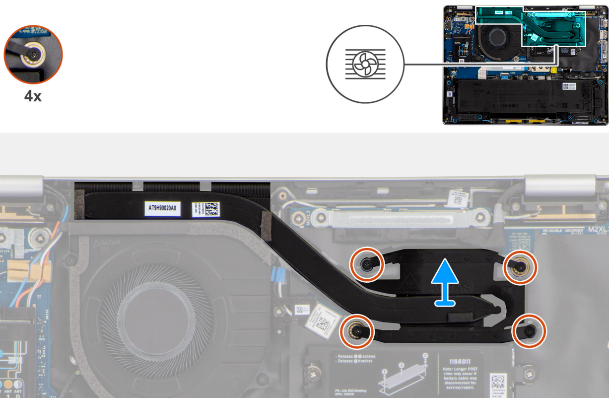
Rysunek 41. Wymontowywanie radiatora
