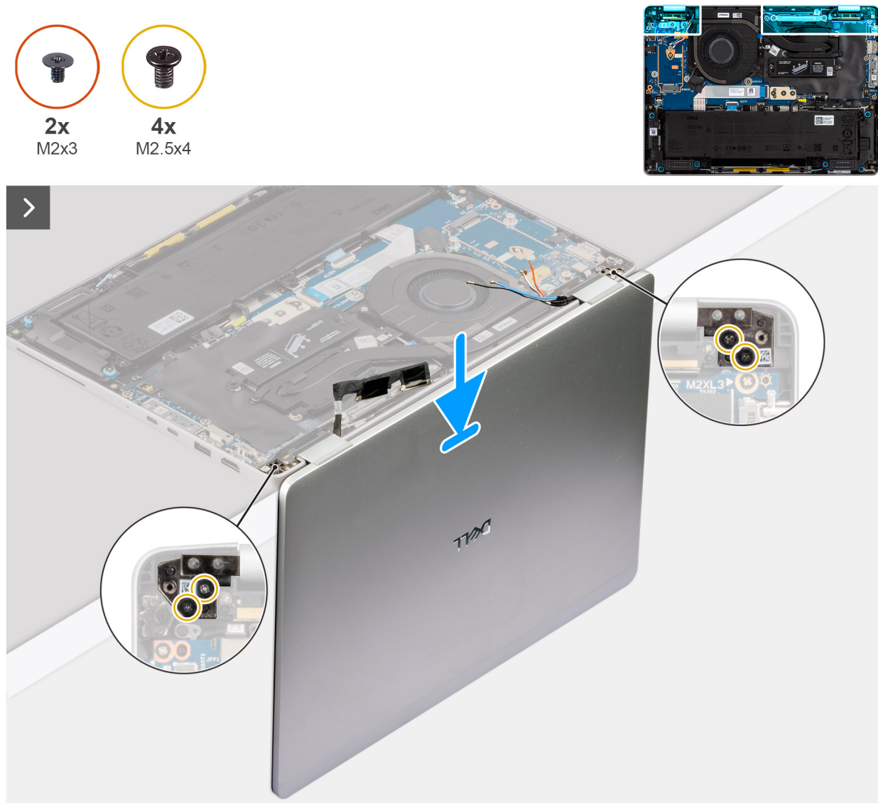
Rysunek 59. Instalowanie zestawu wyświetlacza
