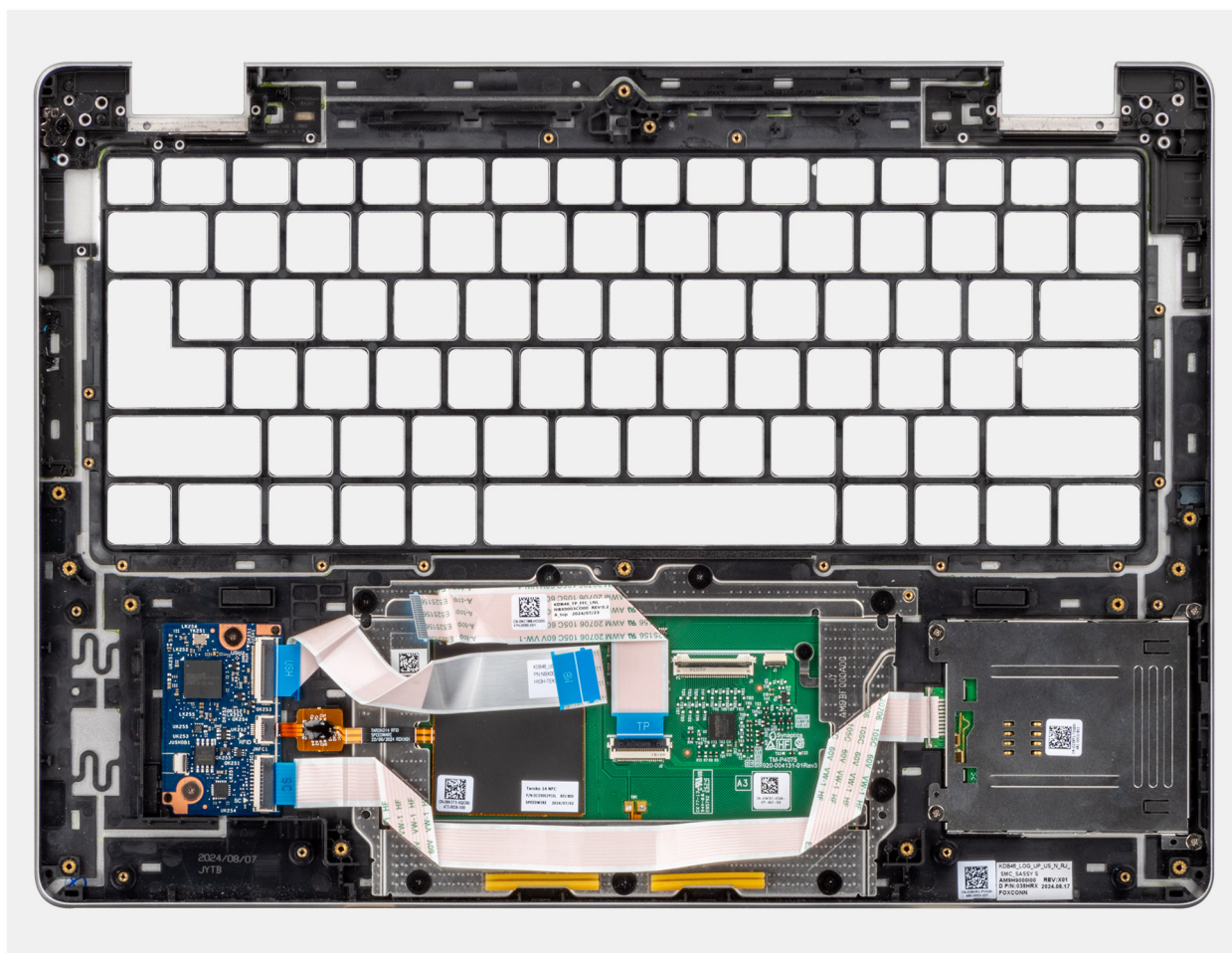
Rysunek 86. Zestaw podpórki na nadgarstek
