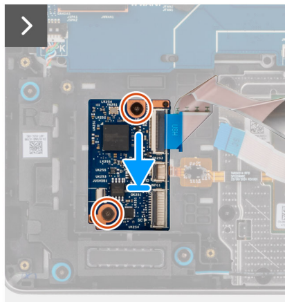
Rysunek 44. Instalowanie karty USH
