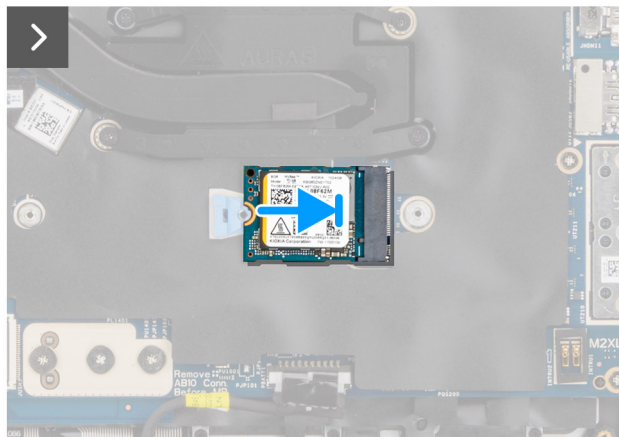
Rysunek 34. Instalowanie dysku SSD M.2 2230
