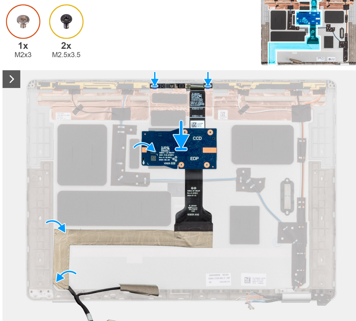
Rysunek 76. Instalowanie kamery i wyświetlacza
