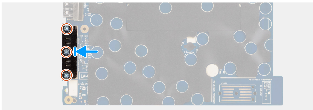
Rysunek 52. Instalowanie modułu złącza USB Type-C
