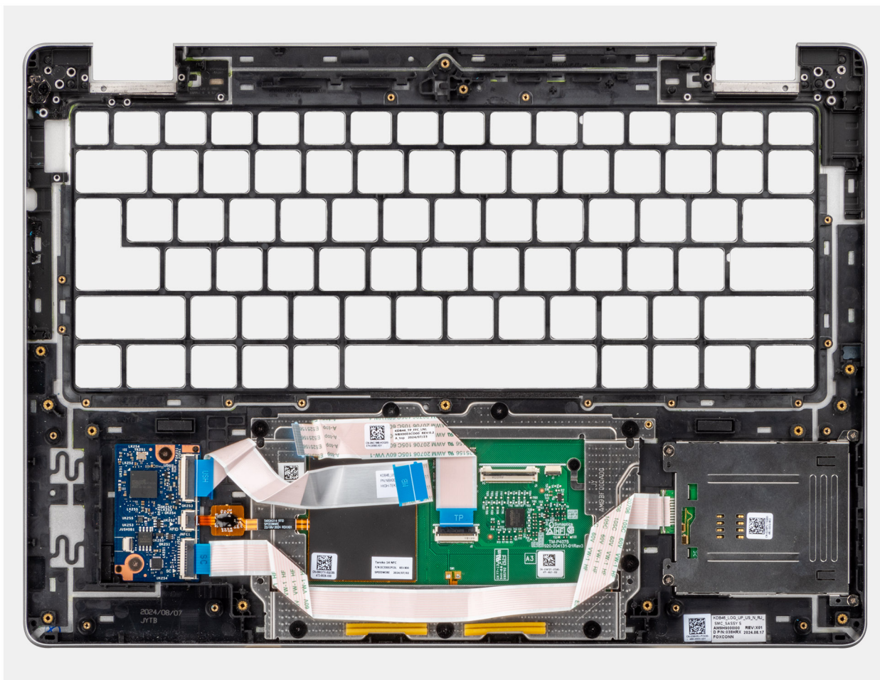
Rysunek 85. Zestaw podpórki na nadgarstek
