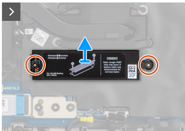
Rysunek 33. Wymontowywanie dysku SSD M.2 2230
