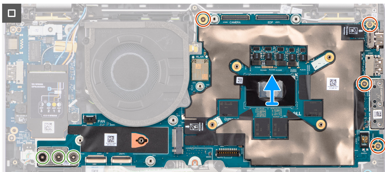
Rysunek 47. Wymontowywanie płyty głównej
