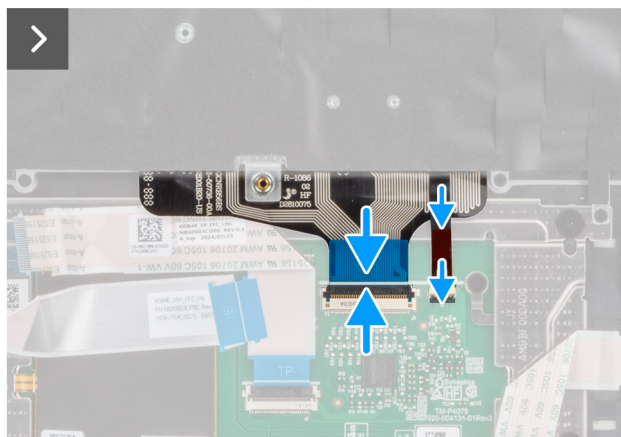
Rysunek 100. Instalowanie klawiatury
