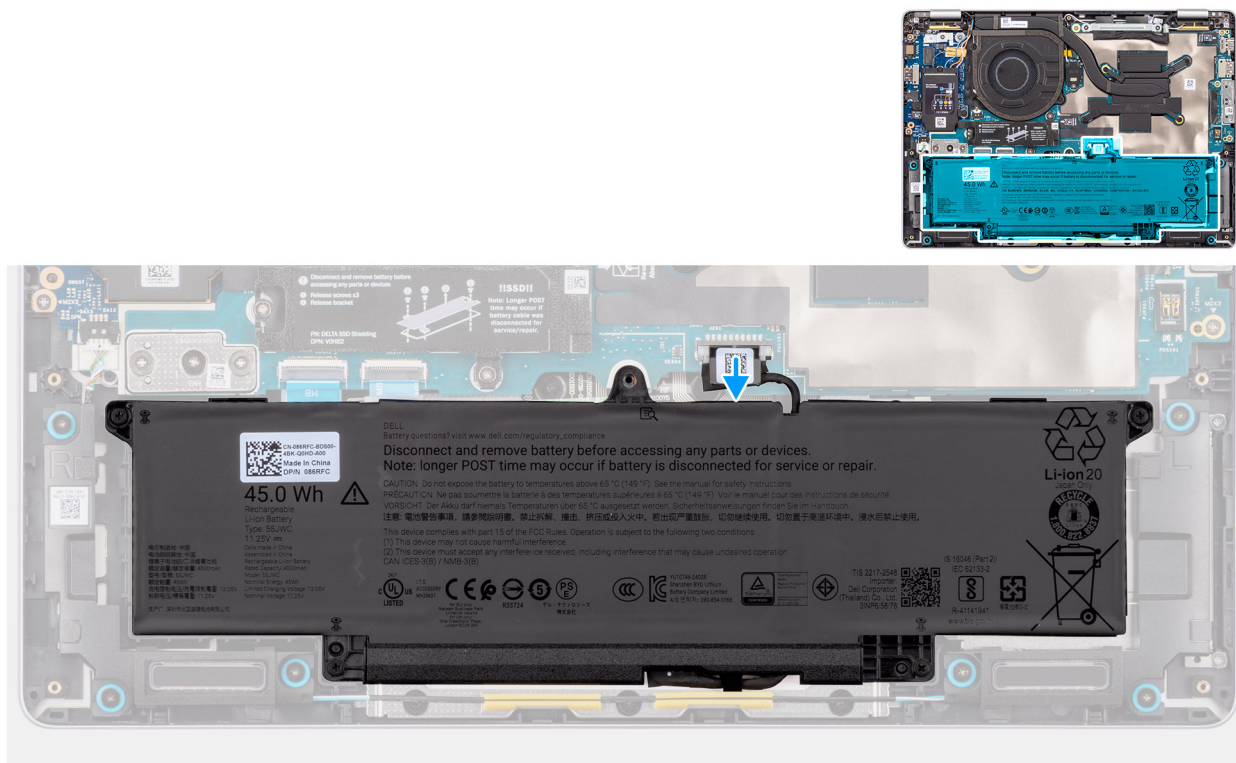
Rysunek 19. Odłączenie kabla baterii
