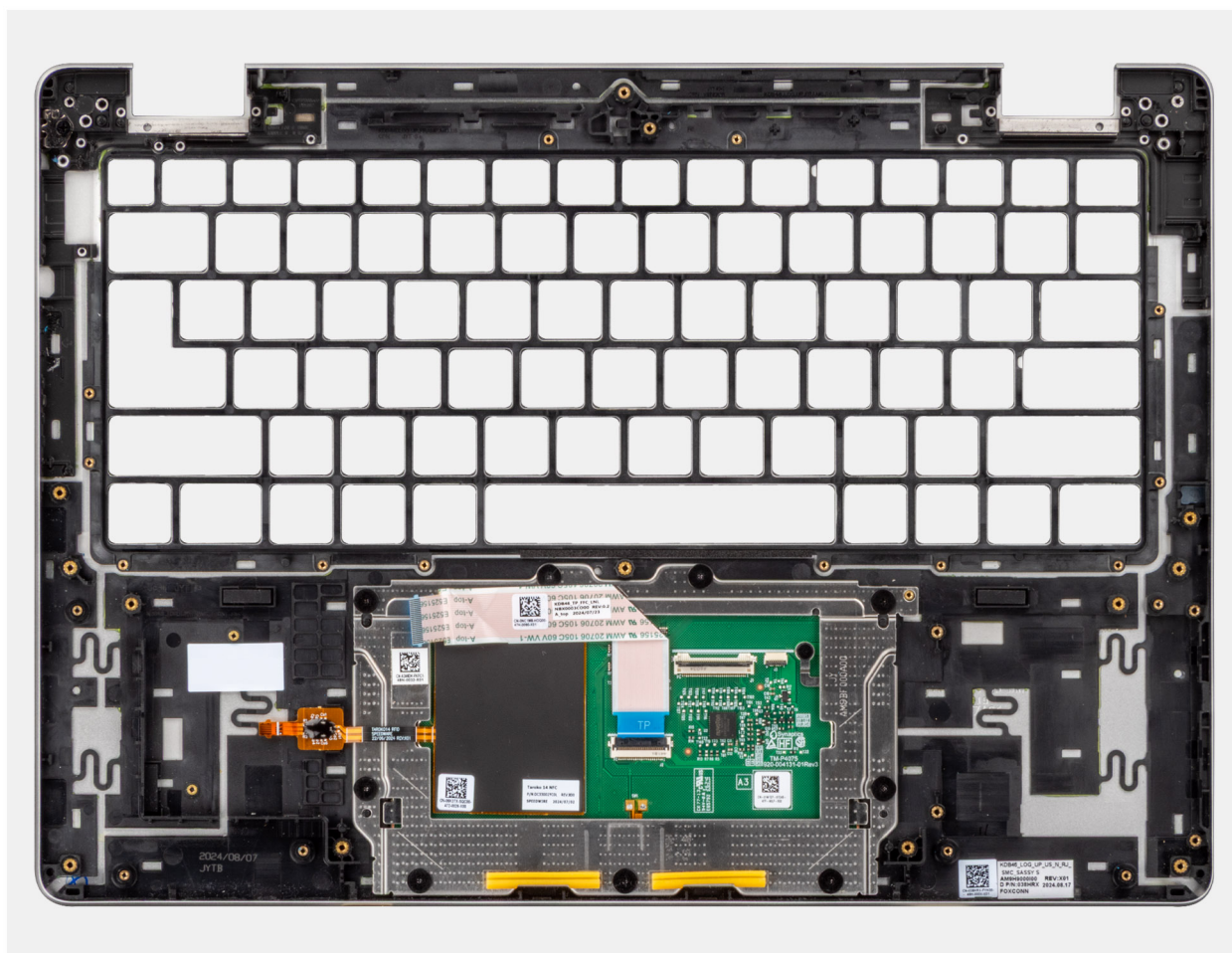
Rysunek 101. Zestaw podpórki na nadgarstek
