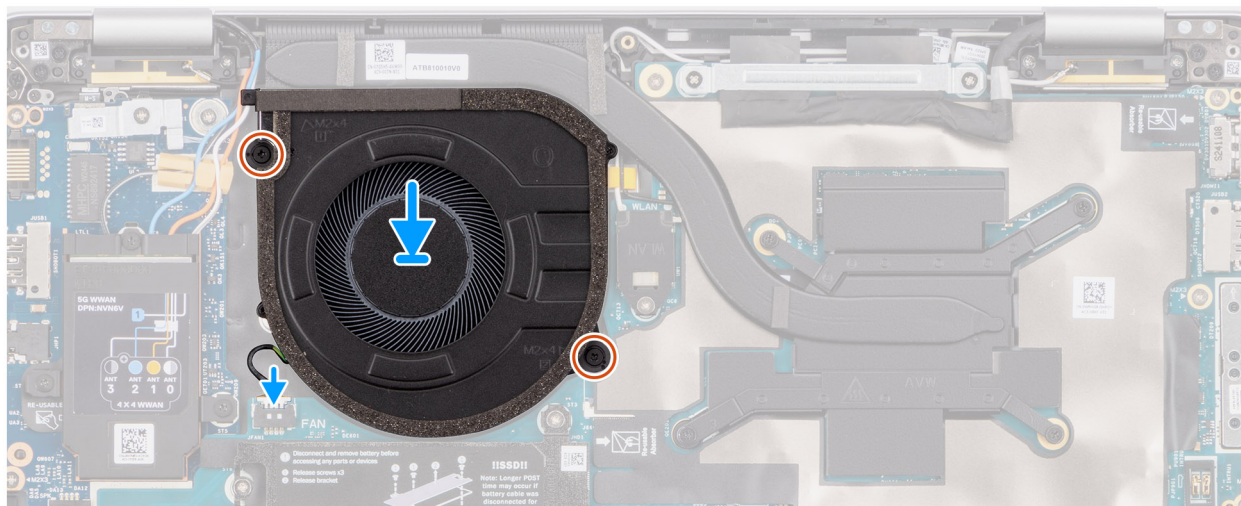
Rysunek 39. Instalowanie wentylatora
