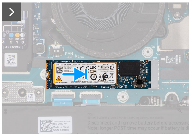
Rysunek 34. Instalowanie dysku SSD M.2 2280
