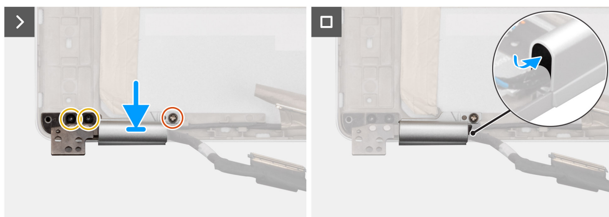
Rysunek 88. Instalowanie wyświetlacza kamery RGB/IR
