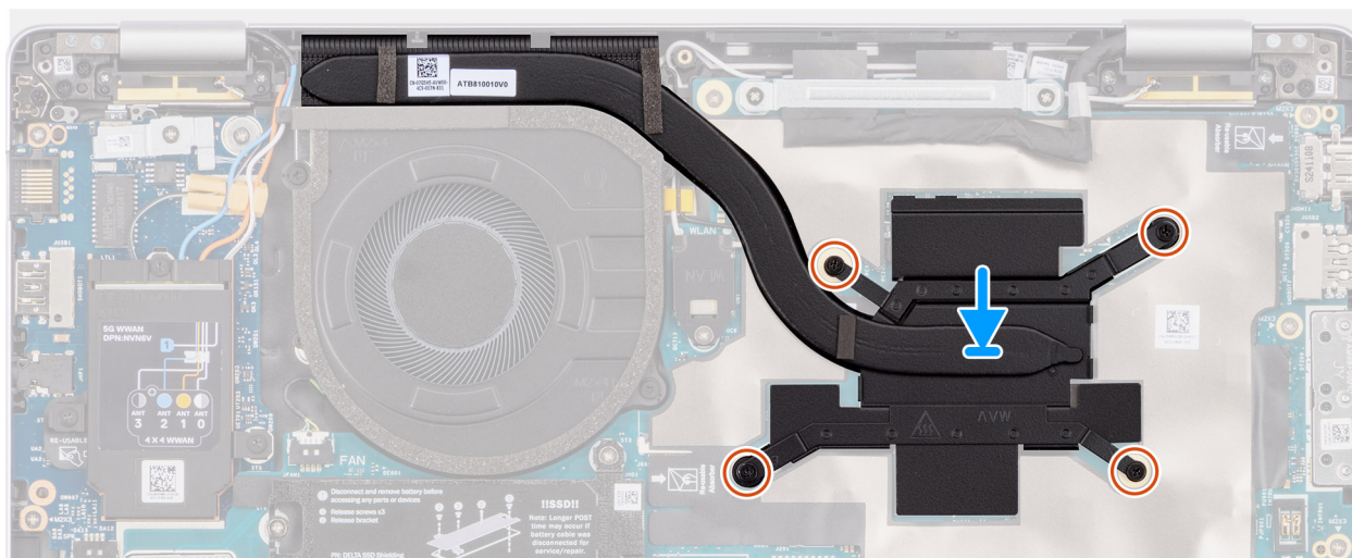
Rysunek 41. Instalowanie radiatora
