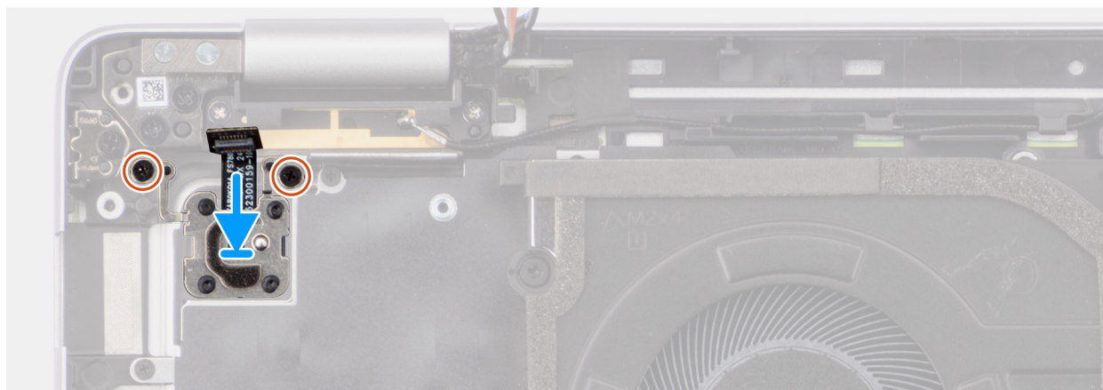
Rysunek 60. Instalowanie przycisku zasilania z opcjonalnym czytnikiem linii papilarnych
