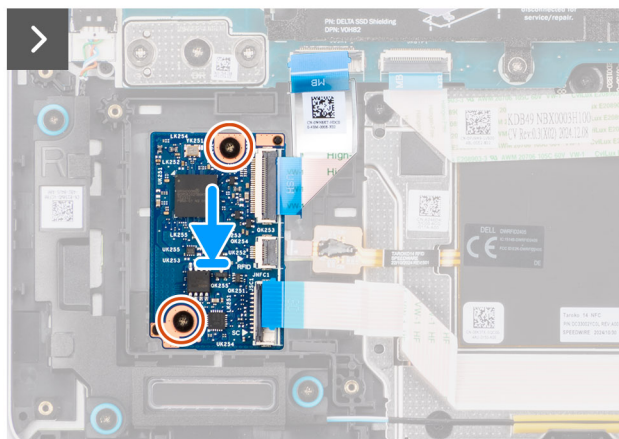
Rysunek 43. Instalowanie karty USH
