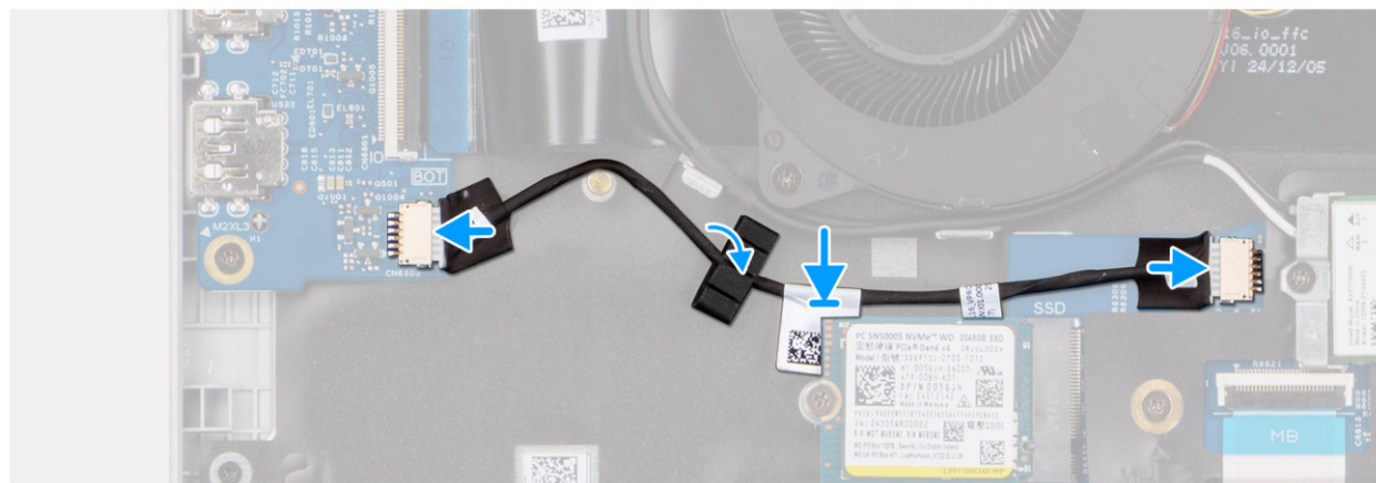
Rysunek 48. Instalowanie vPro
