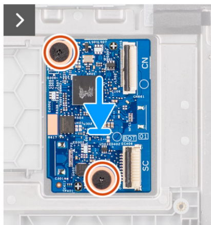
Rysunek 38. Instalowanie karty USH
