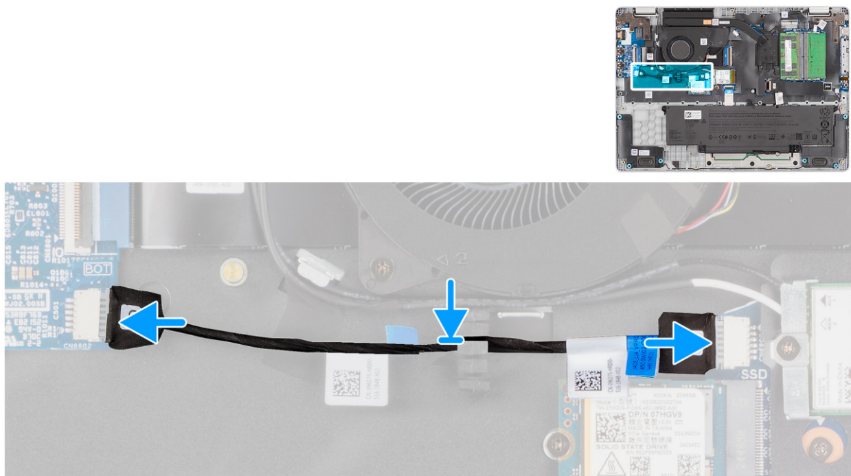
Rysunek 46. Instalowanie vPro
