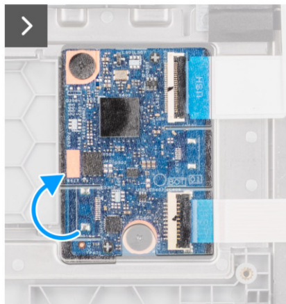
Rysunek 37. Wymontowywanie karty USH
