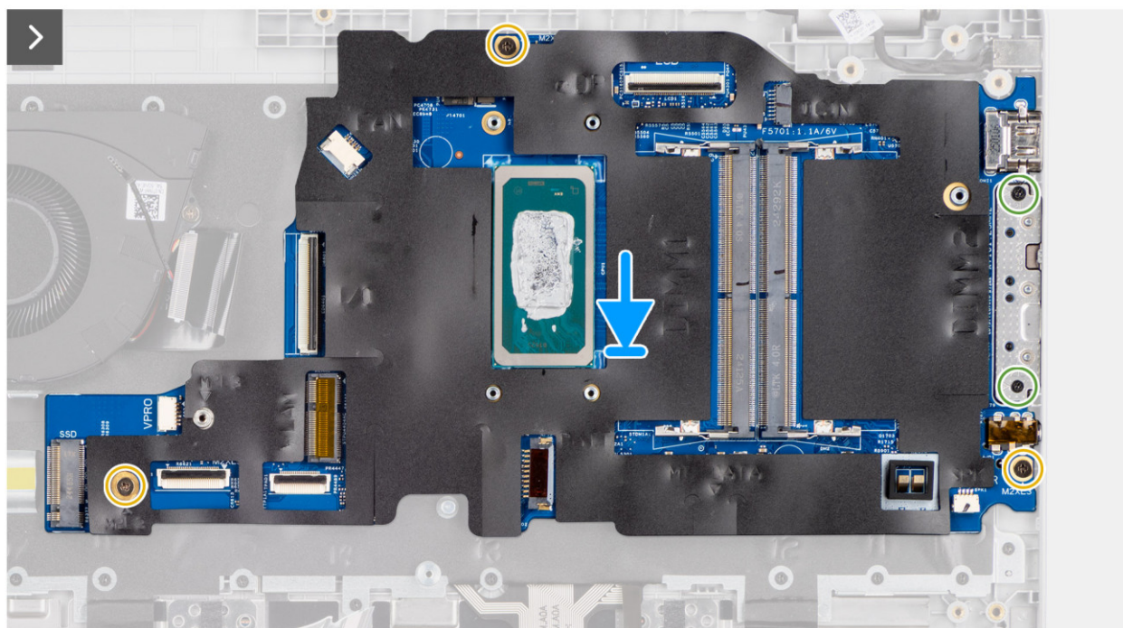
Rysunek 73. Instalowanie płyty głównej
