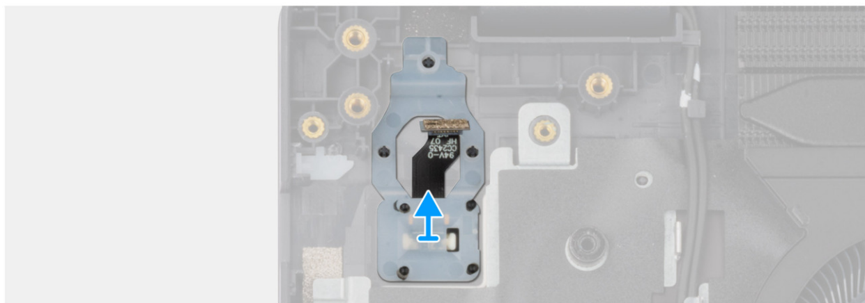
Rysunek 55. Wymontowywanie przycisku zasilania z czytnikiem linii papilarnych
