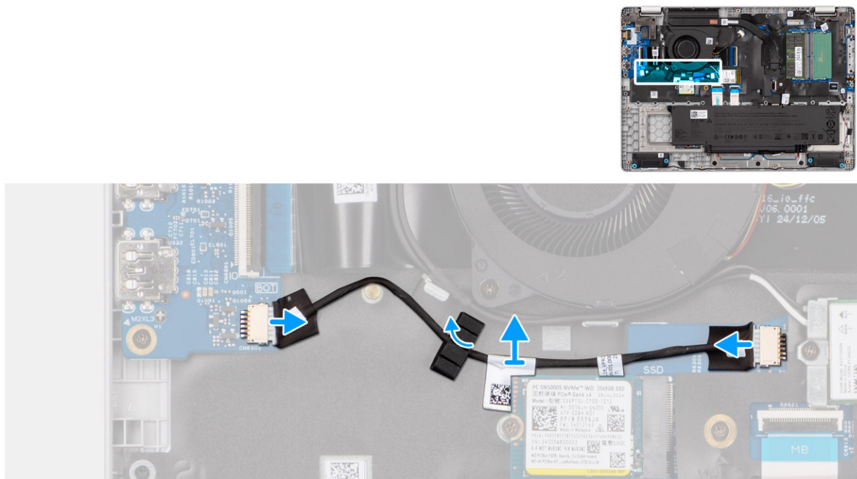
Rysunek 47. Wymontowywanie vPro
