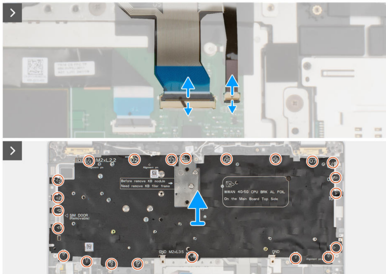
Rysunek 84. Wymontowywanie klawiatury
