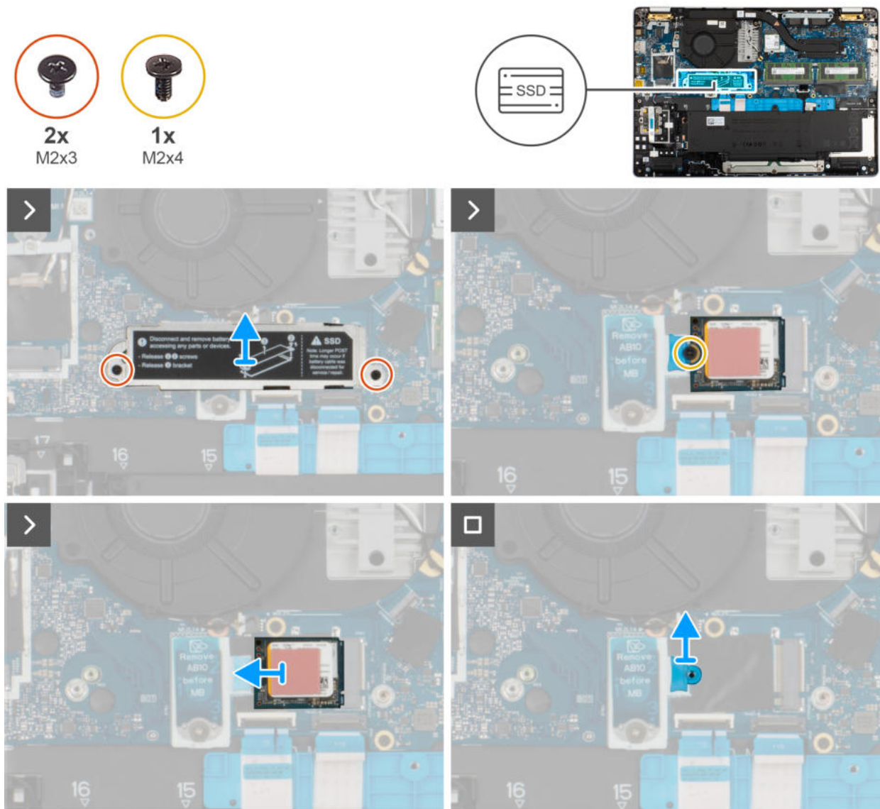
Rysunek 24. Wymontowywanie dysku SSD M.2 2230
