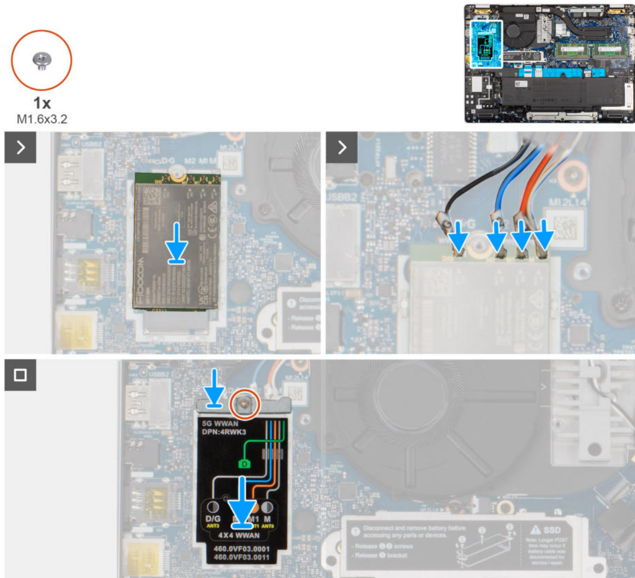
Rysunek 32. Instalowanie karty sieci WWAN 5G
