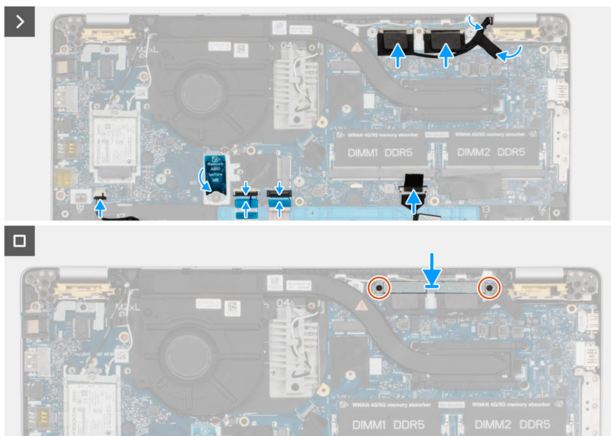
Rysunek 56. Instalowanie płyty głównej
