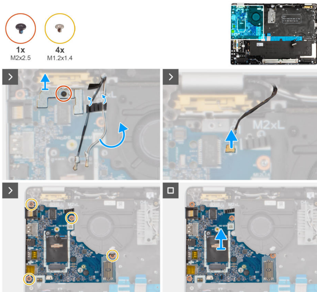
Rysunek 57. Wymontowywanie panelu we/wy
