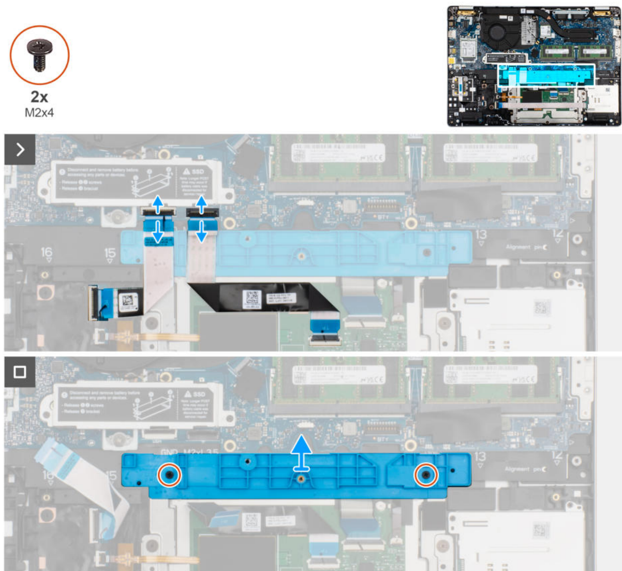
Rysunek 47. Wymontowywanie wspornika baterii
