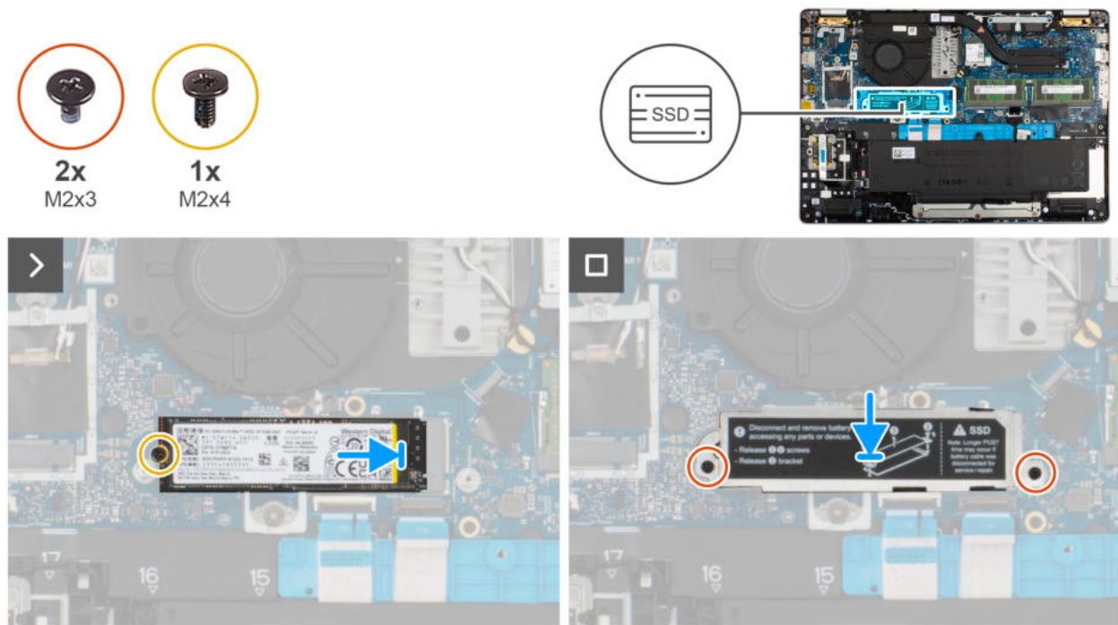
Rysunek 28. Instalowanie dysku SSD M.2230
