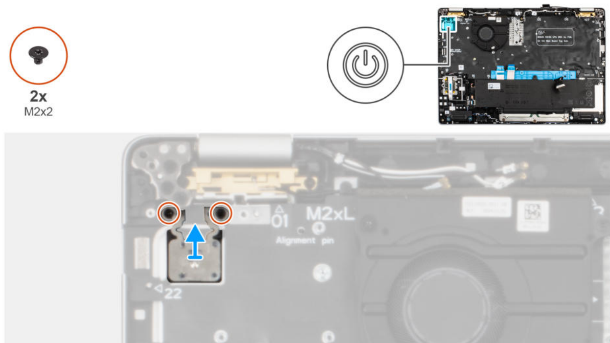
Rysunek 59. Instalowanie przycisku zasilania z opcjonalnym czytnikiem linii papilarnych
