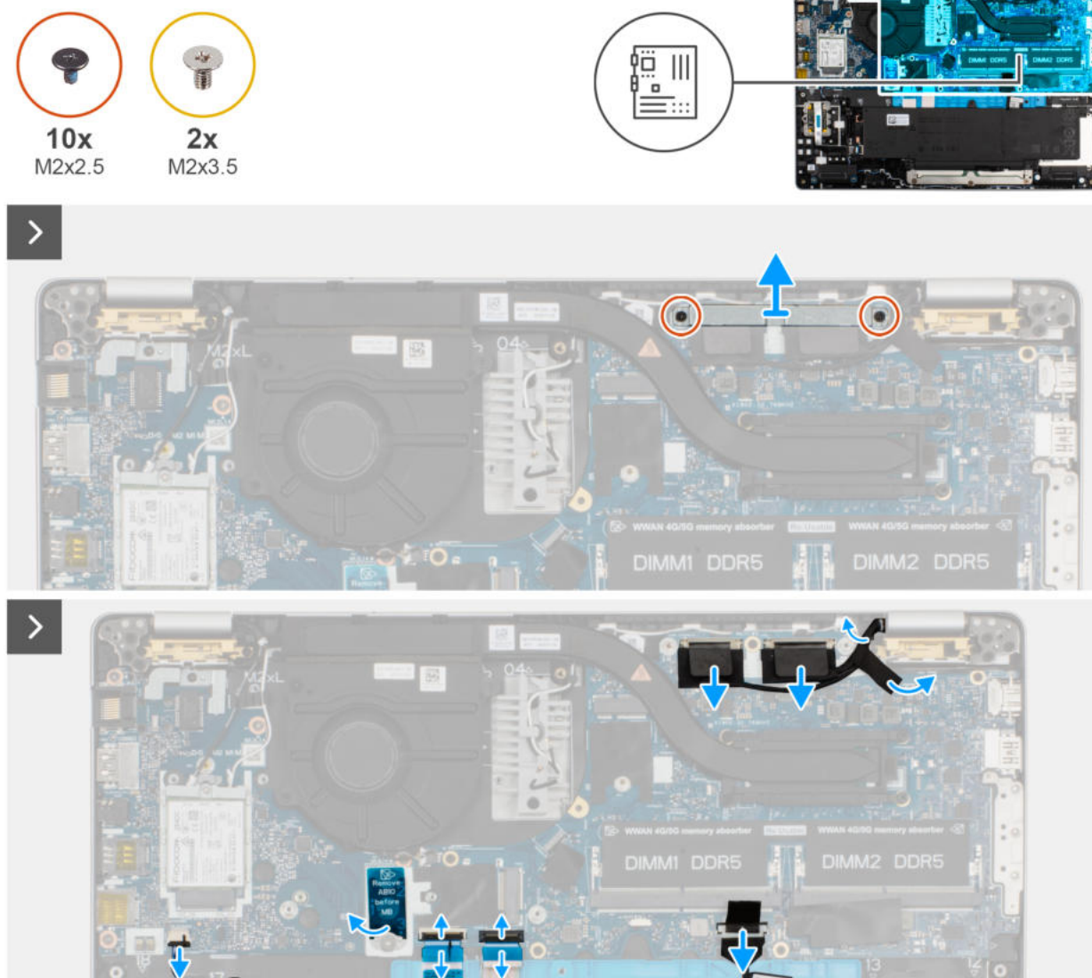
Rysunek 52. Wymontowywanie płyty głównej
