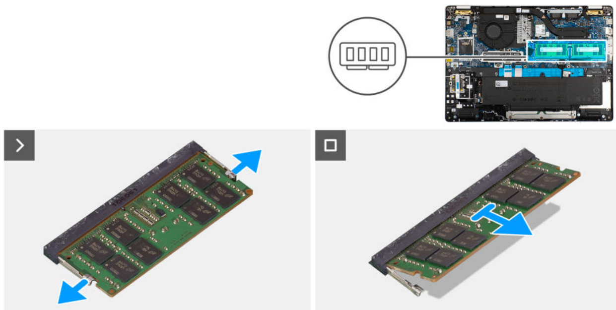
Rysunek 22. Wymontowywanie modułu pamięci
