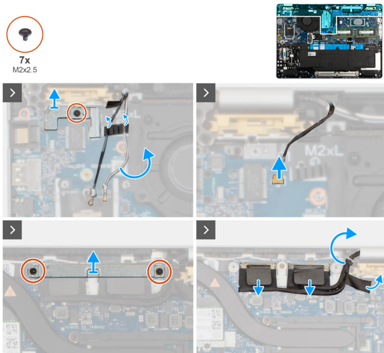
Rysunek 43. Wymontowywanie anteny sieci WLAN
