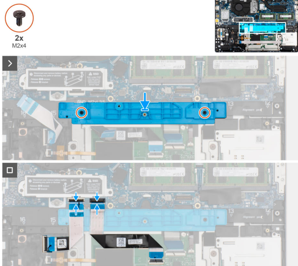
Rysunek 48. Instalowanie klamry wspornika baterii
