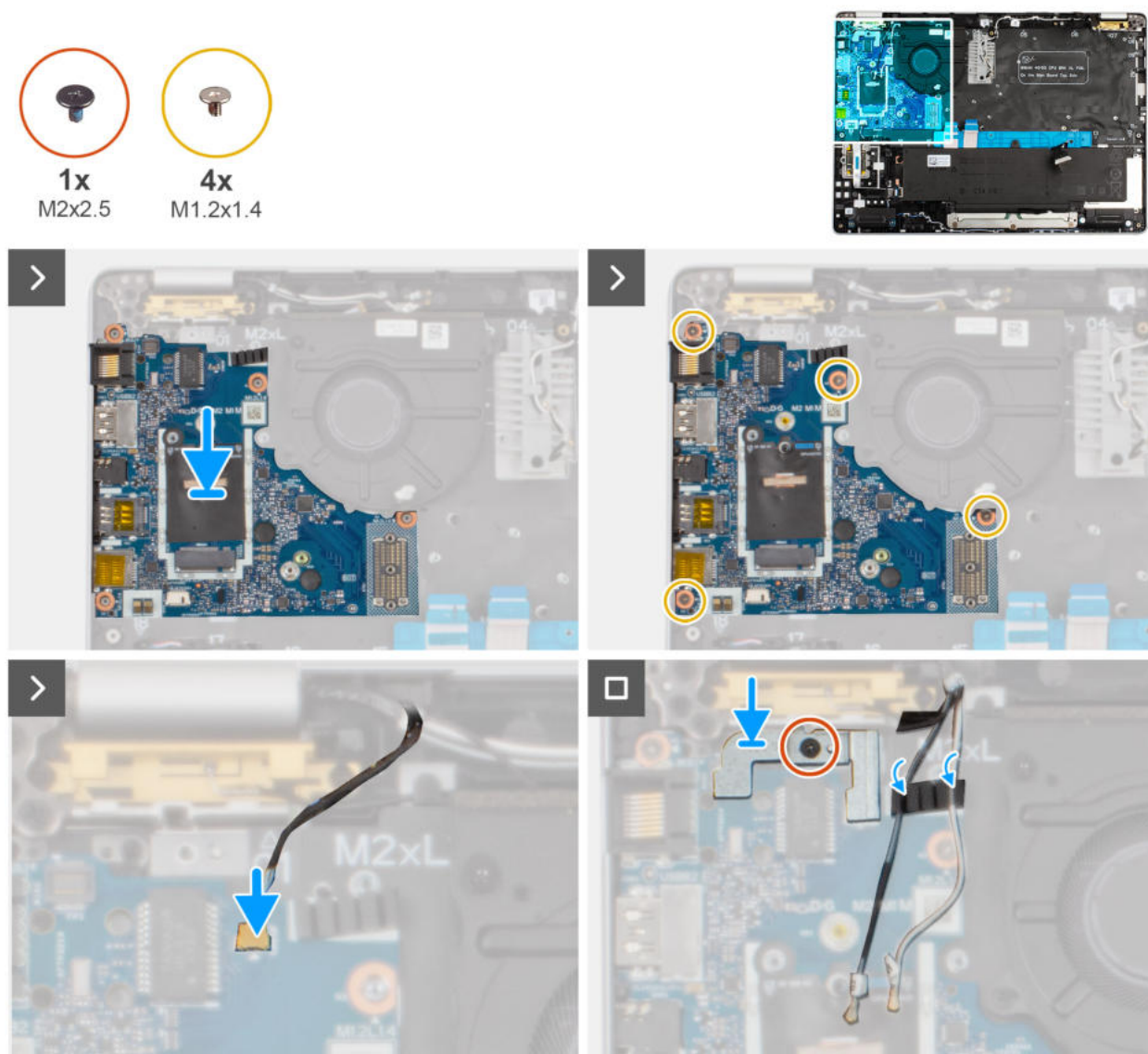
Rysunek 58. Wymontowywanie płyty we/wy
