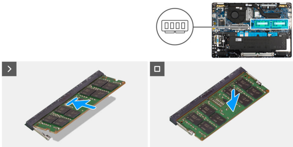
Rysunek 23. Instalowanie modułów pamięci
