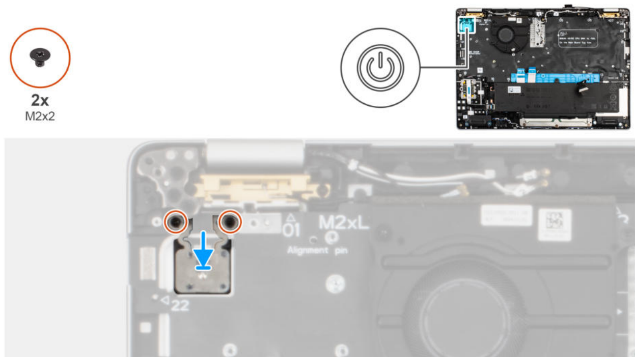
Rysunek 60. Instalowanie przycisku zasilania z opcjonalnym czytnikiem linii papilarnych
