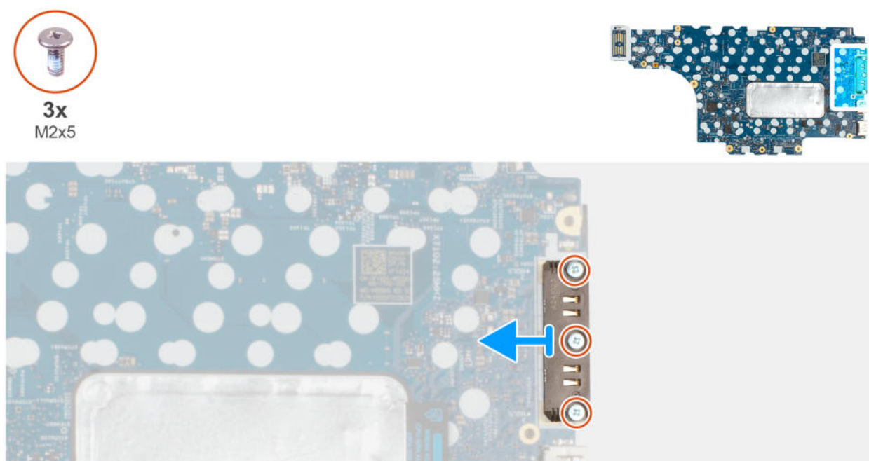
Rysunek 82. Wymontowywanie modułu łącznika USB Type-C
