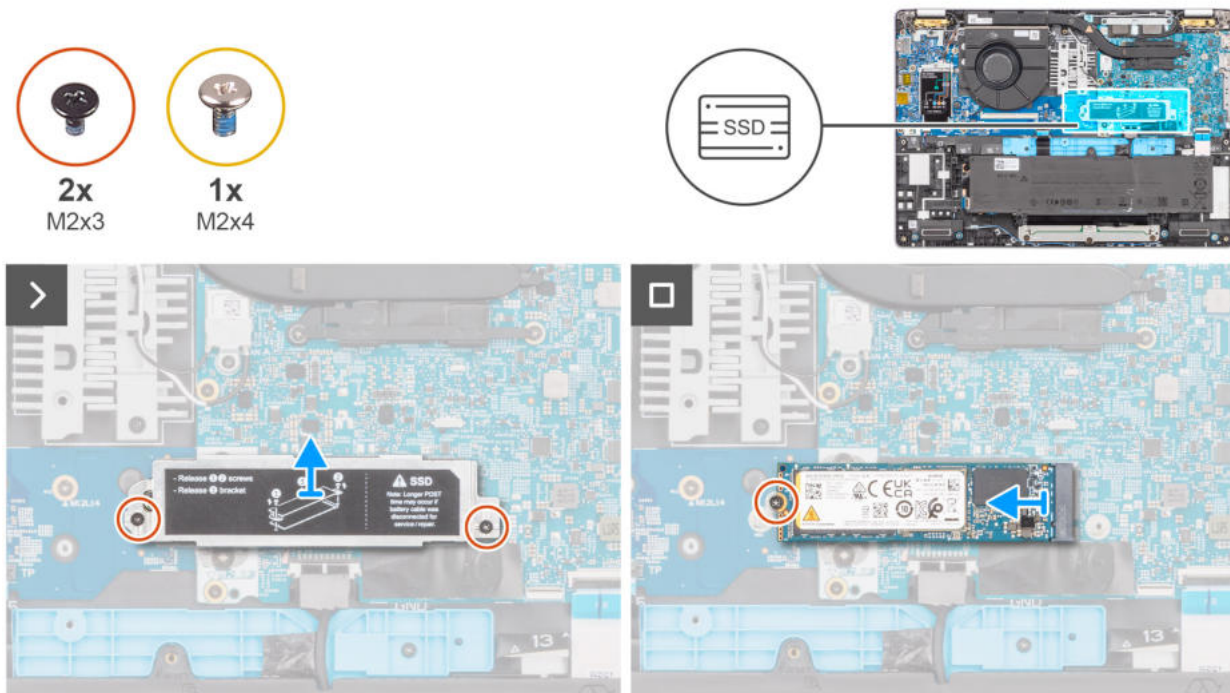
Rysunek 24. Wymontowywanie dysku SSD M.2 2280
