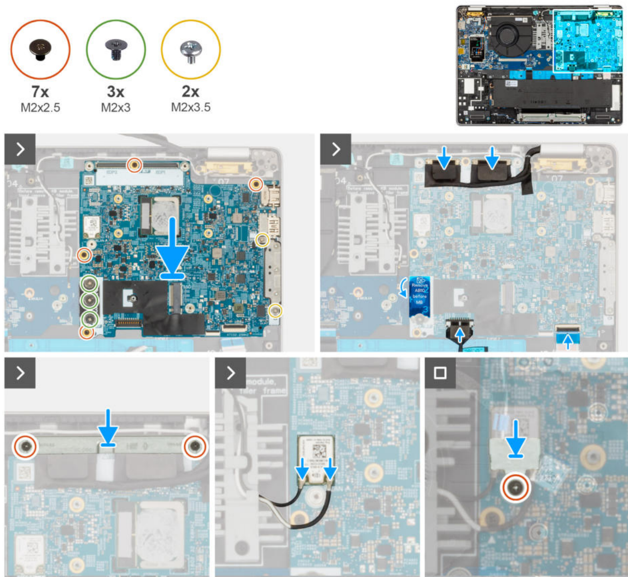
Rysunek 50. Instalowanie płyty głównej
