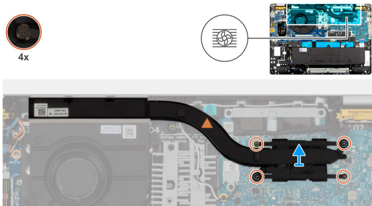
Rysunek 45. Wymontowywanie radiatora
