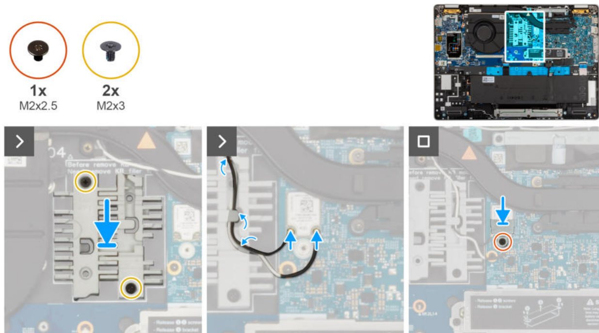
Rysunek 85. Instalowanie zaślepki klawiatury
