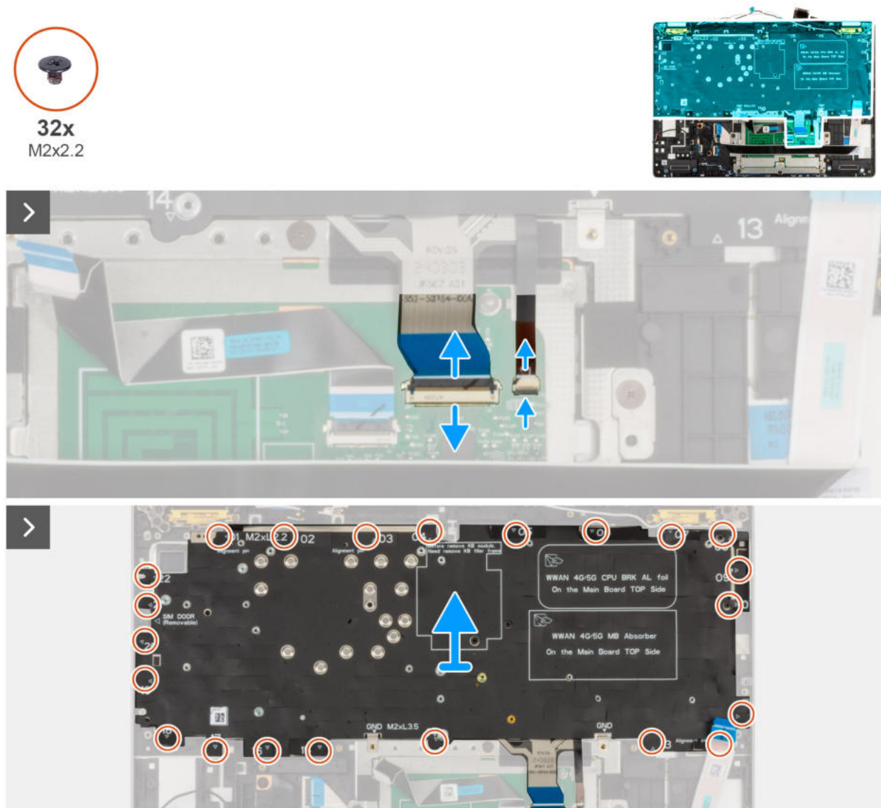
Rysunek 79. Wymontowywanie klawiatury
