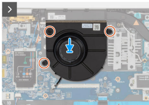
Rysunek 29. Instalowanie wentylatora
