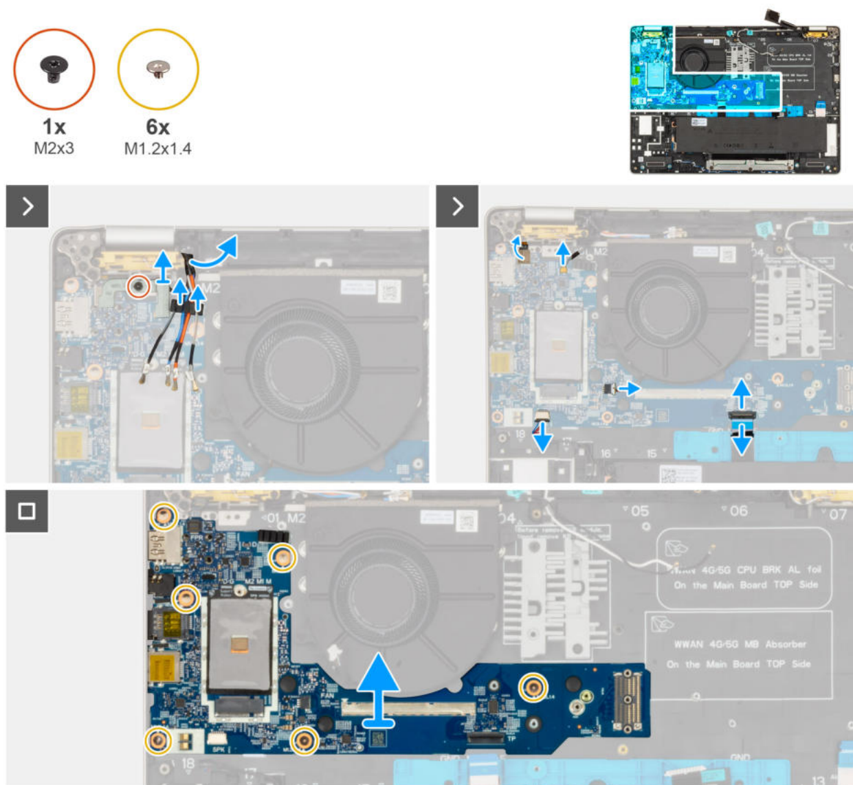
Rysunek 51. Wymontowywanie panelu we/wy
