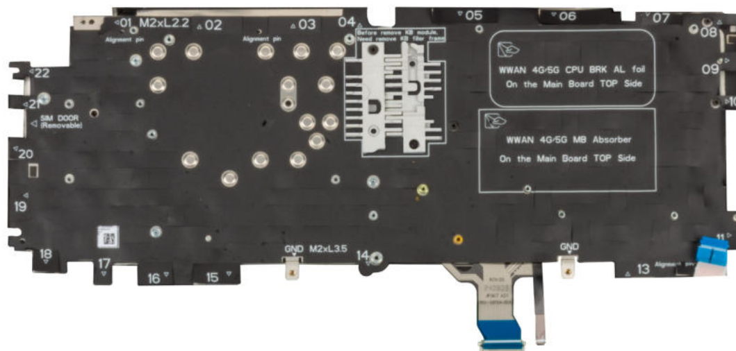
Rysunek 84. Instalowanie zaślepki klawiatury
