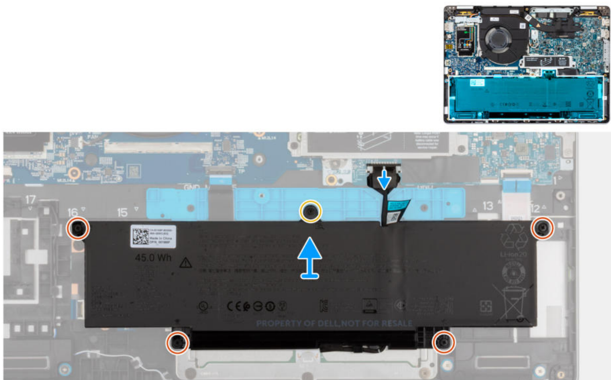
Rysunek 15. Odłączanie kabla baterii
