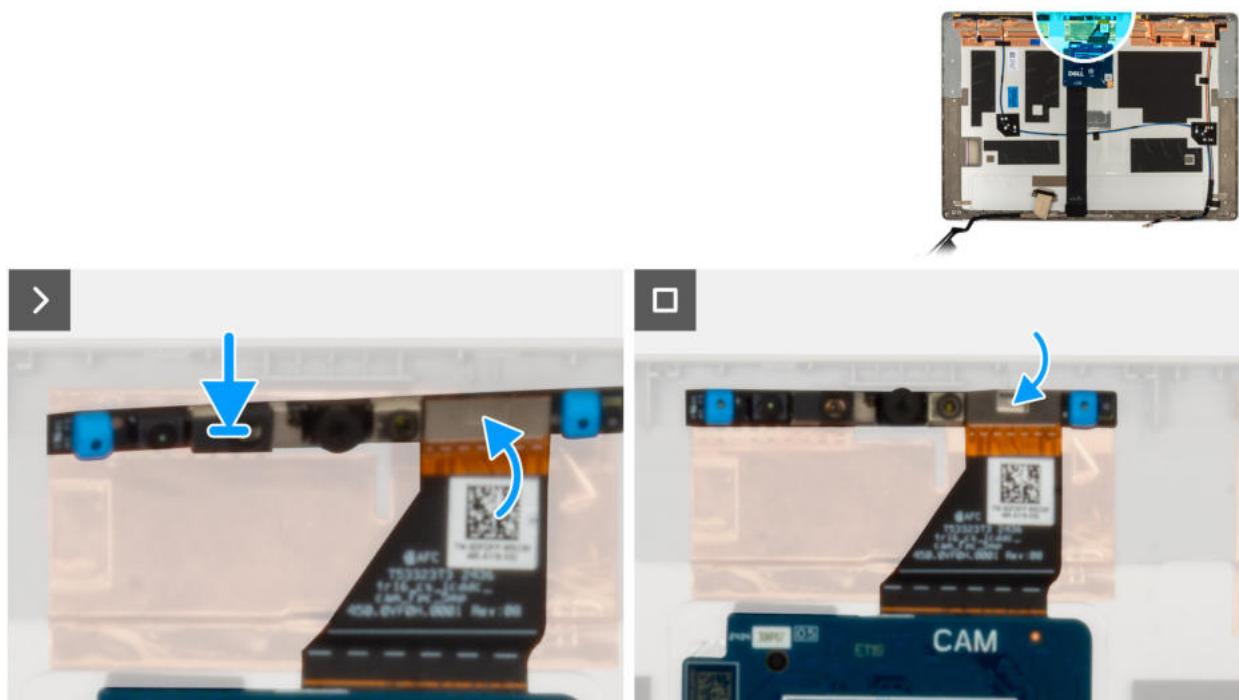
Rysunek 74. Instalowanie modułu kamery
