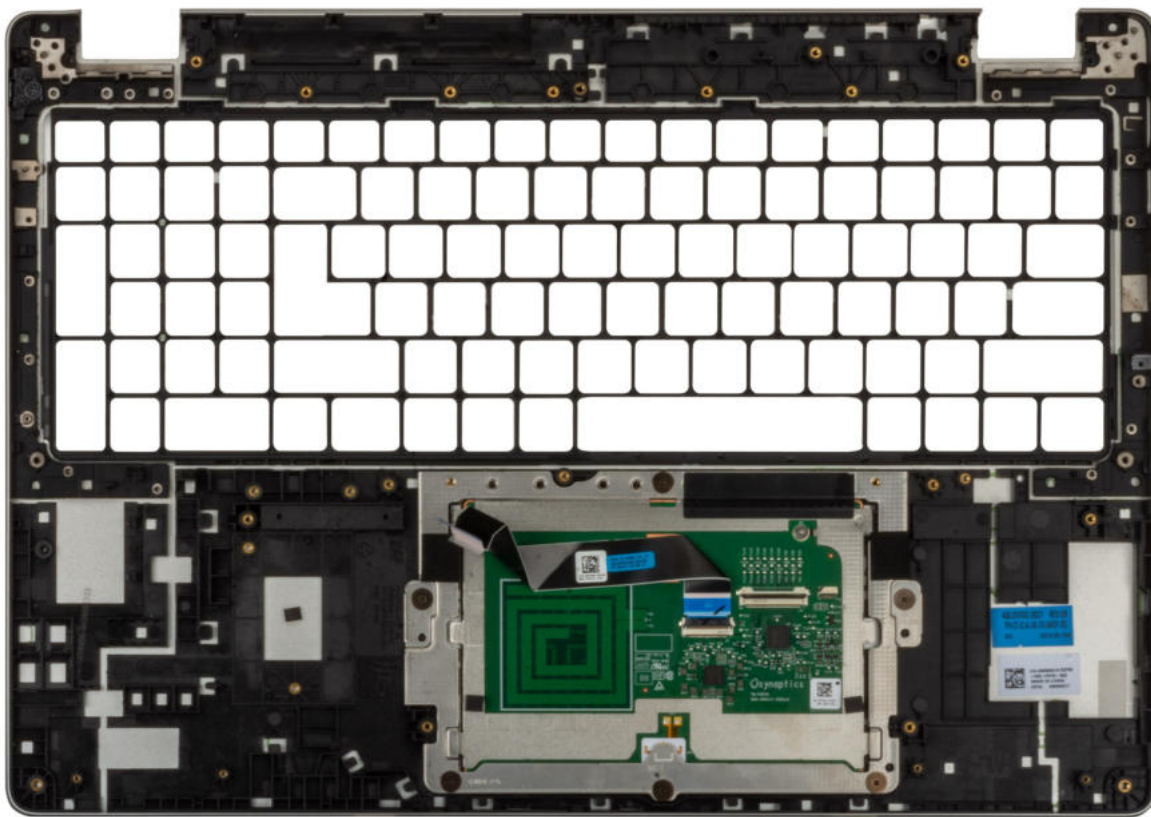
Rysunek 87. Wymontowywanie zestawu podpórki na nadgarstek
