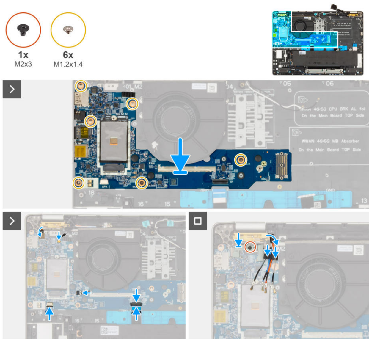
Rysunek 52. Instalowanie płyty we/wy
