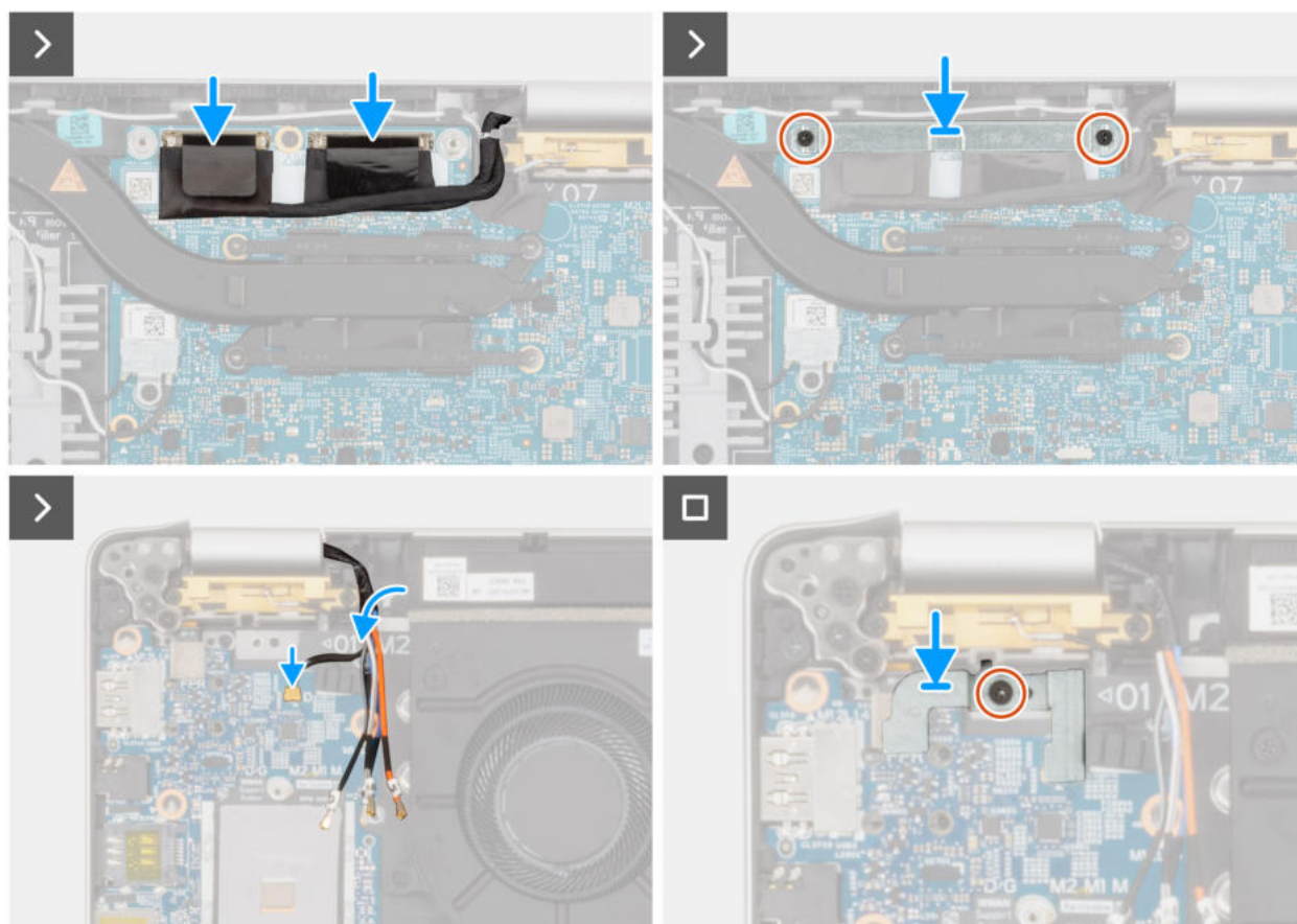
Rysunek 58. Instalowanie zestawu wyświetlacza
