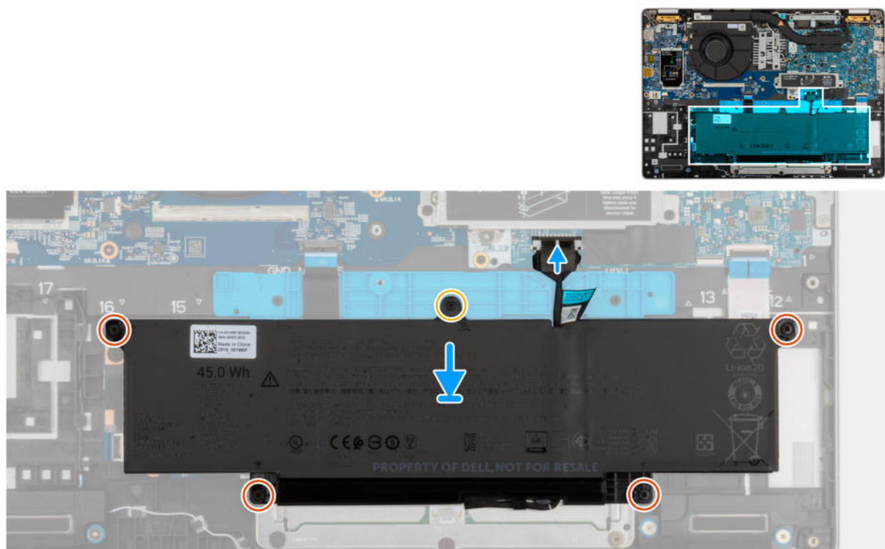
Rysunek 16. Podłączanie kabla baterii
