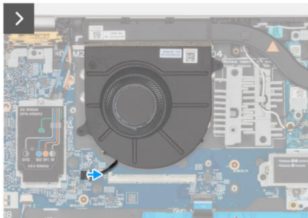
Rysunek 28. Wymontowywanie wentylatora
