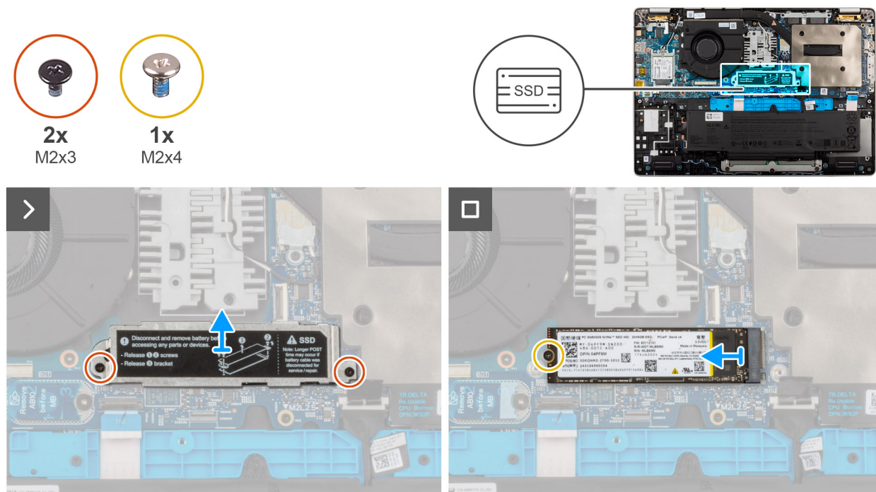
Rysunek 26. Wymontowywanie dysku SSD M.2 2280
