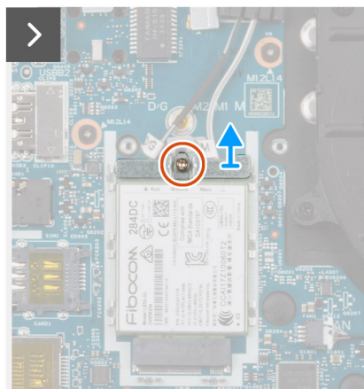
Rysunek 28. Wymontowywanie karty sieci WWAN 4G
