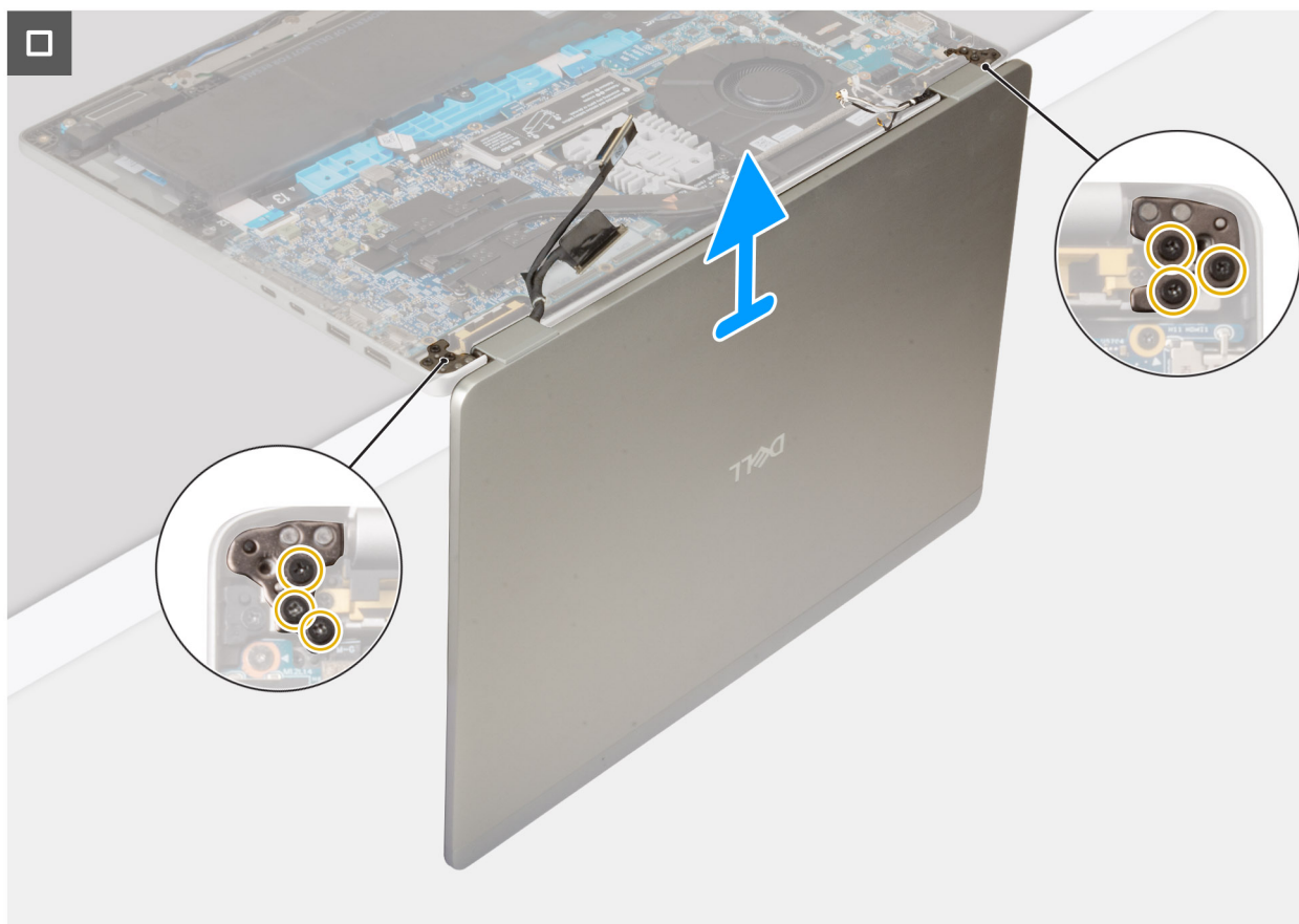
Rysunek 53. Wymontowywanie zestawu wyświetlacza
