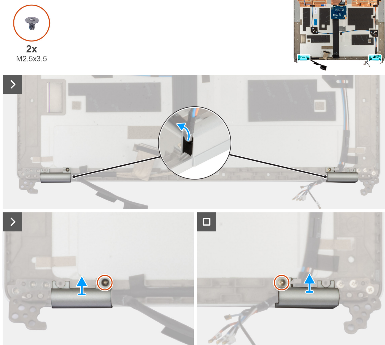
Rysunek 68. Zdejmowanie osłon zawiasów wyświetlacza
