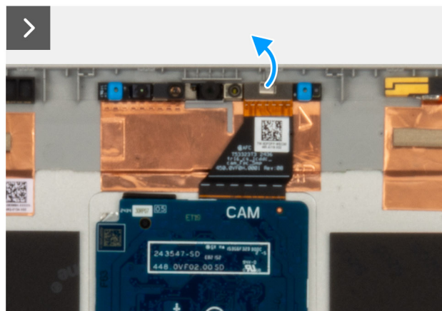
Rysunek 72. Wymontowywanie modułu kamery
