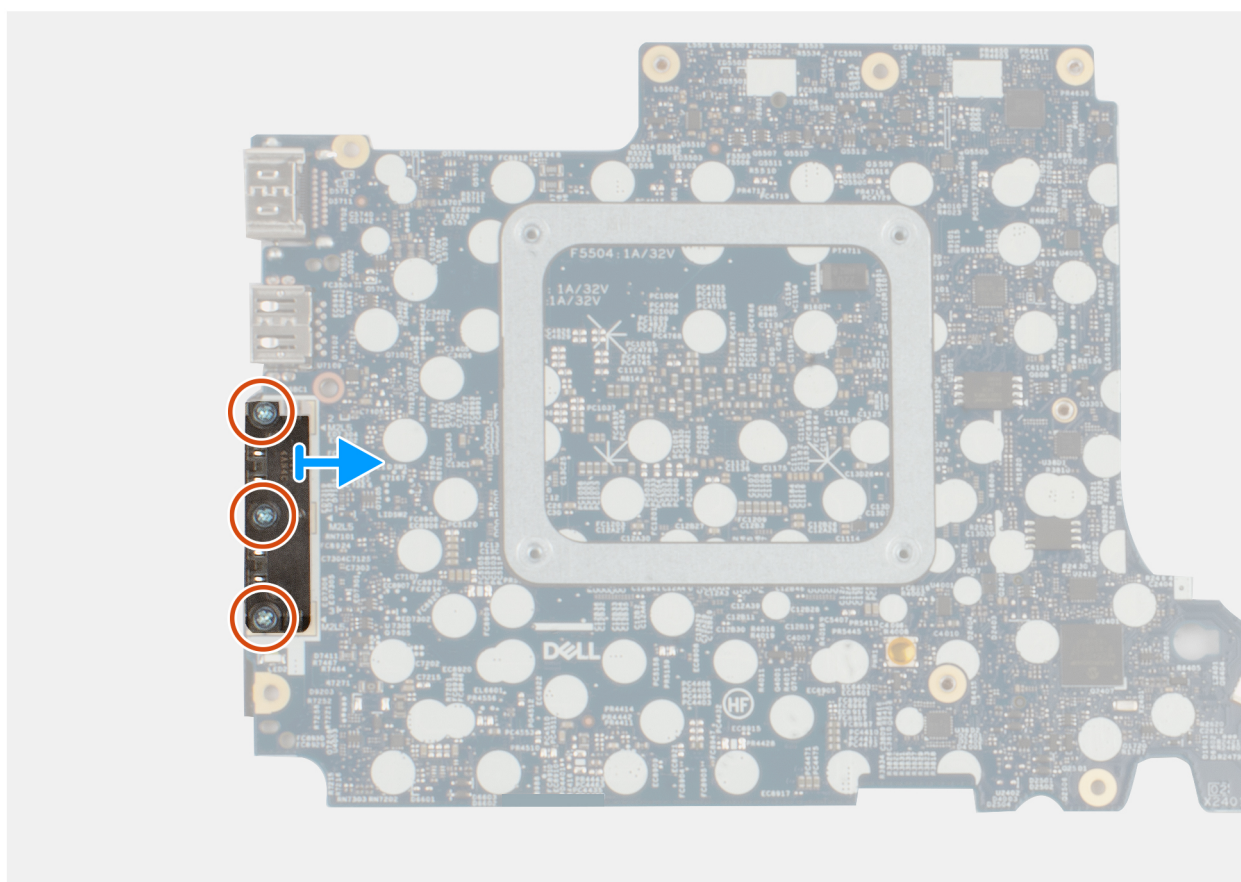
Rysunek 48. Wymontowywanie modułu łącznika USB Type-C
