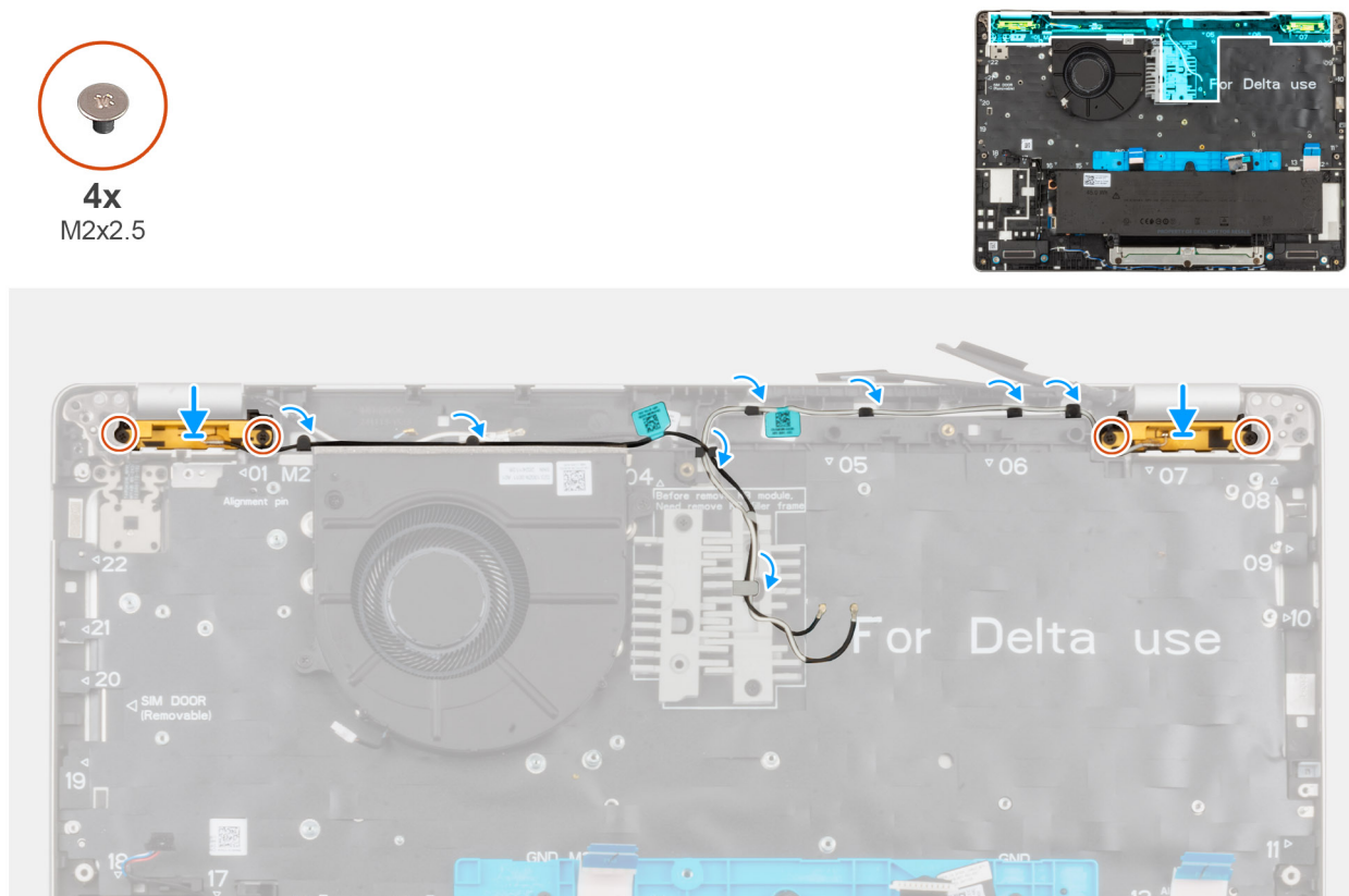
Rysunek 77. Instalowanie anteny sieci bezprzewodowej
