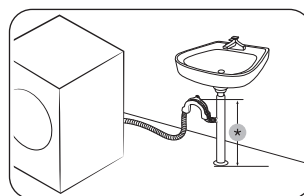
W odgałęzieniu rury odprowadzającej wodę z umywalki
