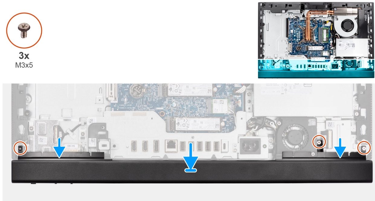
Rysunek 36. Instalowanie pokrywki dolnej
