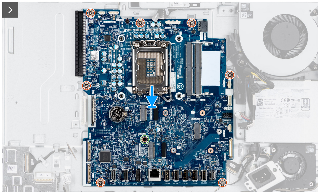
Rysunek 69. Instalowanie płyty głównej
