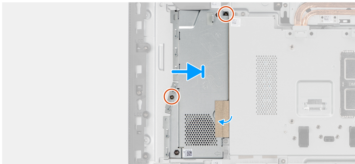
Rysunek 28. Instalowanie zestawu karty graficznej (model bez obsługi dotykowej)
