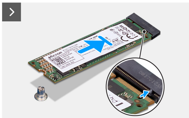
Rysunek 41. Instalowanie dysku SSD M.2 2280 w gnieździe M.2 nr 1
