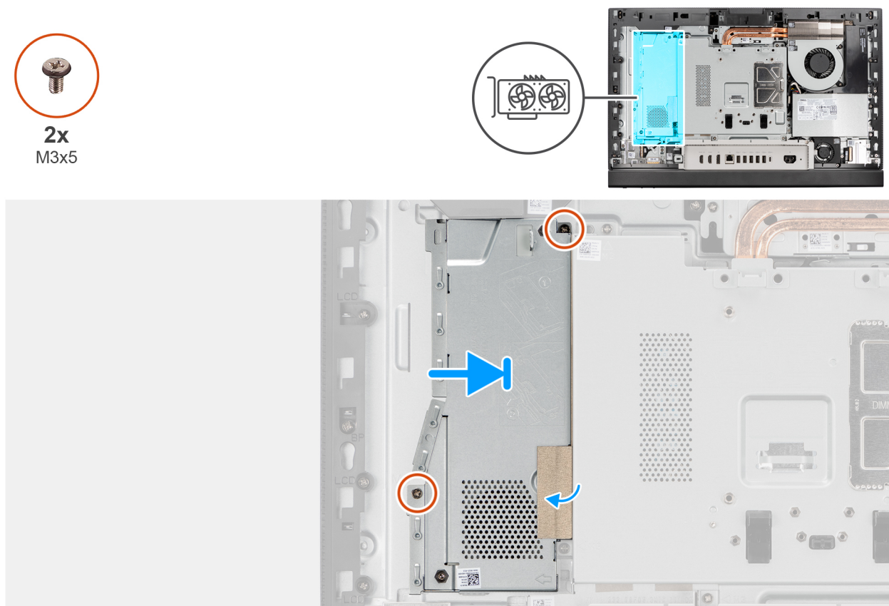
Rysunek 27. Instalowanie zestawu karty graficznej (model z ekranem dotykowym)
