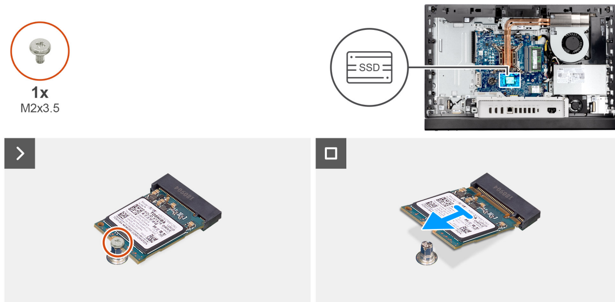
Rysunek 33. Wymontowywanie dysku SSD M.2 2230 z gniazda M.2 nr 0
