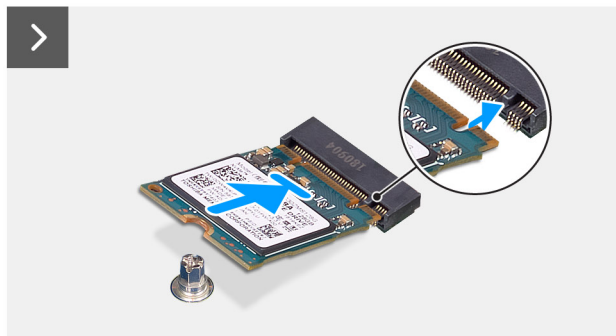
Rysunek 39. Instalowanie dysku SSD M.2 2230 w gnieździe M.2 nr 1
