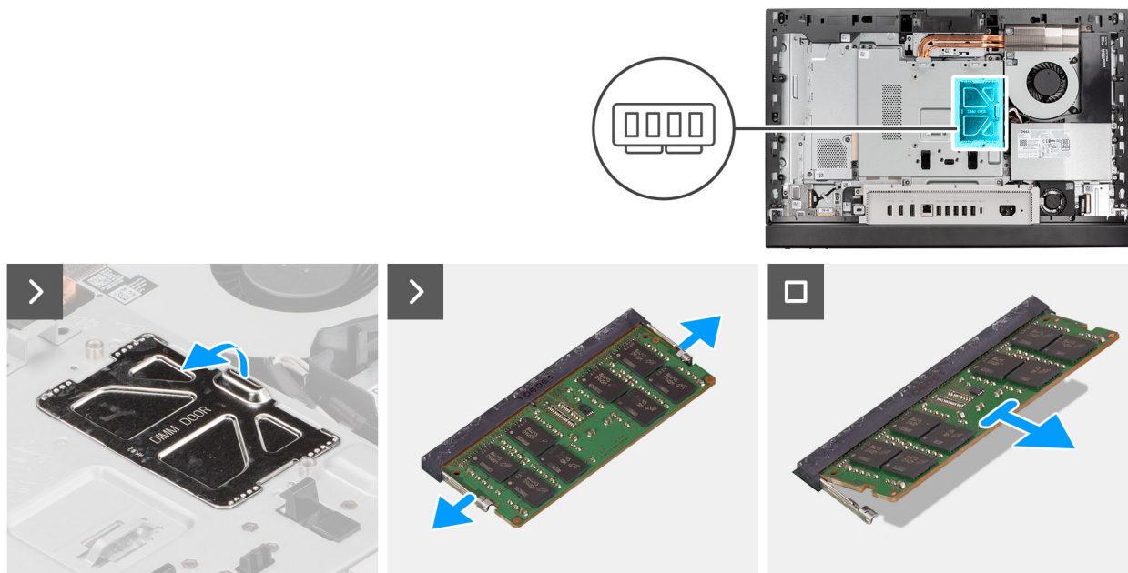
Rysunek 23. Wymontowywanie modułów pamięci
