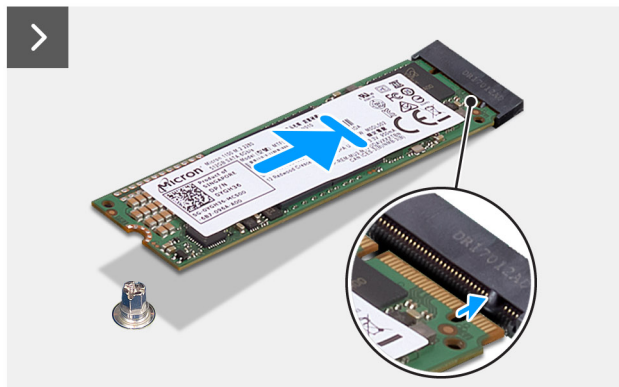
Rysunek 36. Instalowanie dysku SSD M.2 2280 w gnieździe M.2 nr 0
