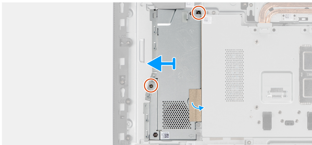
Rysunek 26. Wymontowywanie zestawu karty graficznej (model bez obsługi dotykowej)
