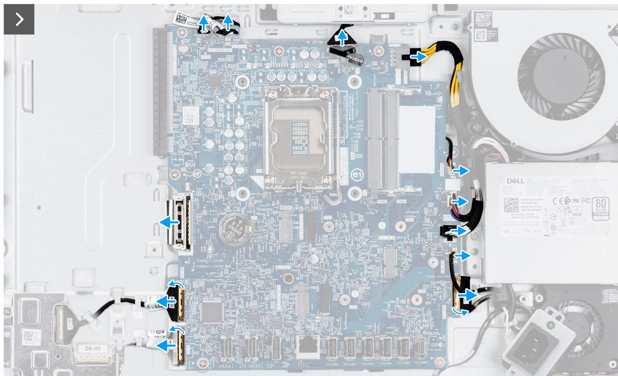
Rysunek 66. Wymontowywanie płyty głównej
