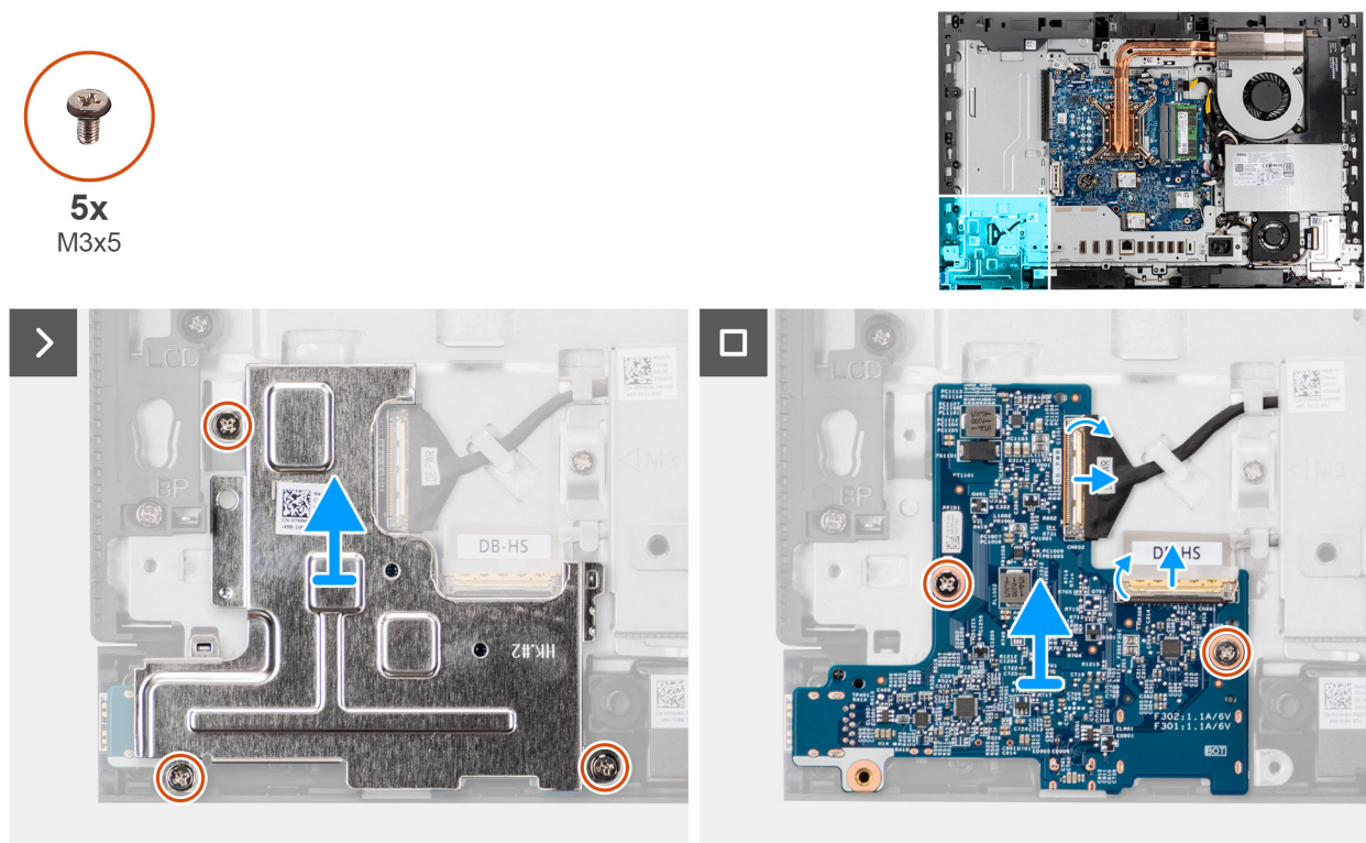
Rysunek 71. Wymontowywanie płyty przycisku zasilania i złączy we/wy
