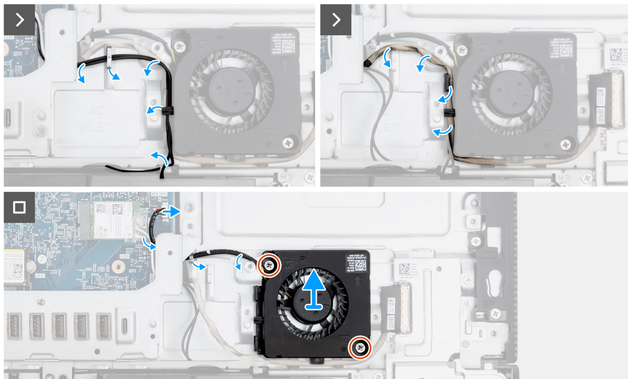
Rysunek 55. Wymontowywanie wentylatora zasilacza
