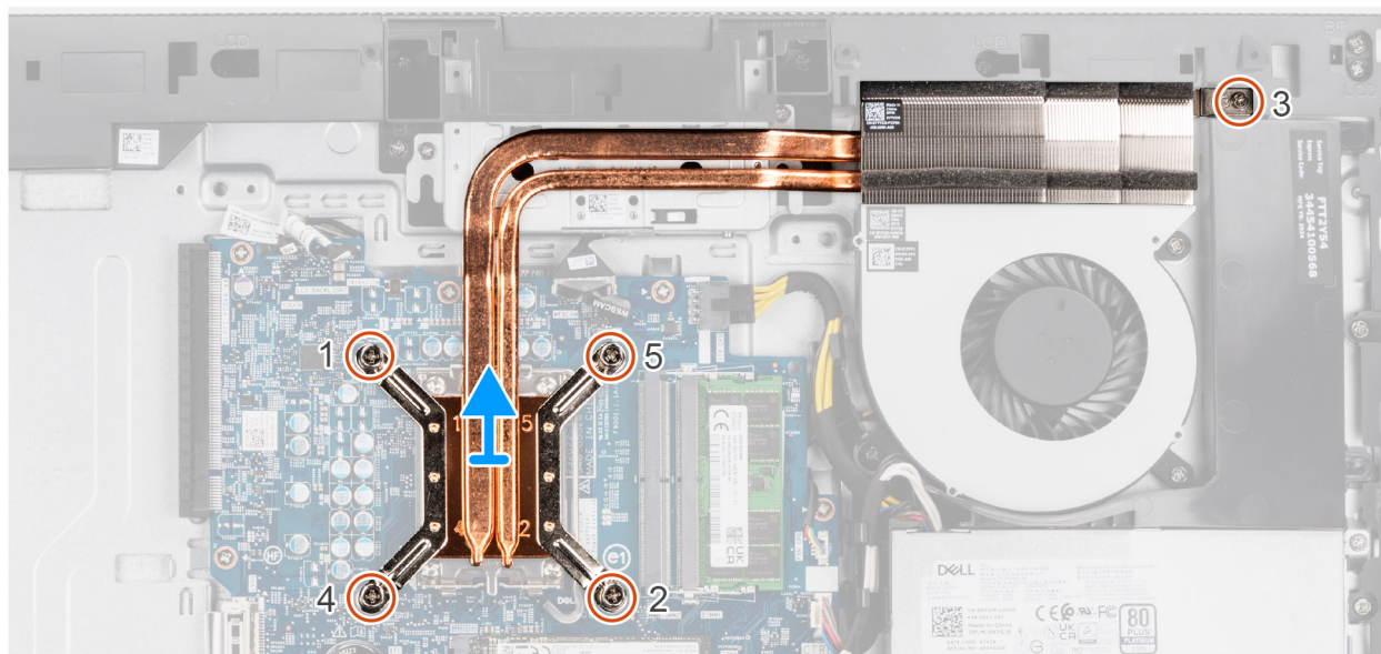
Rysunek 61. Wymontowywanie radiatora
