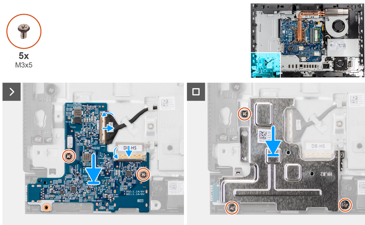
Rysunek 72. Instalowanie płyty przycisku zasilania i złączy we/wy
