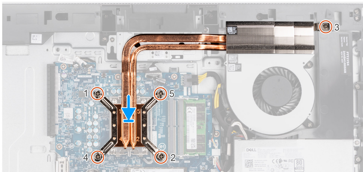
Rysunek 62. Instalowanie radiatora
