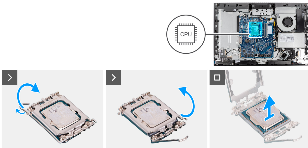
Rysunek 63. Wymontowywanie procesora
