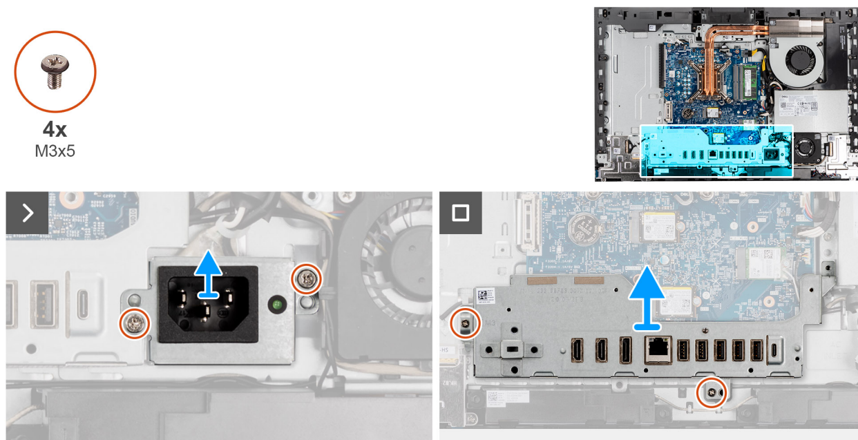
Rysunek 57. Wymontowywanie panelu we/wy
