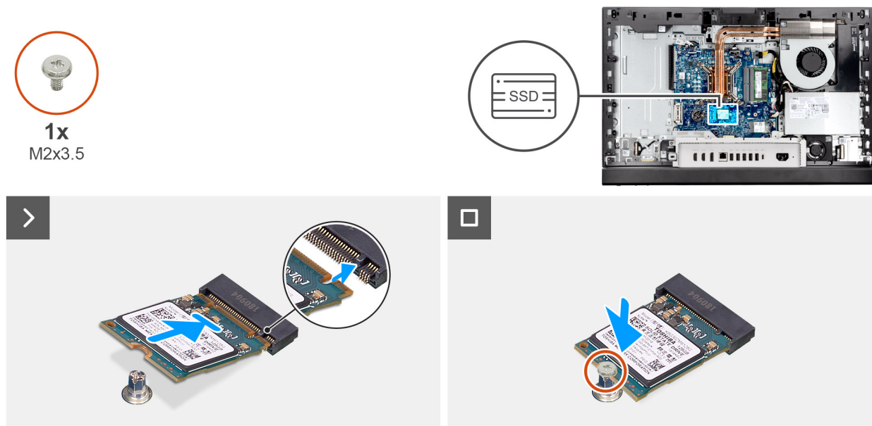
Rysunek 34. Instalowanie dysku SSD M.2 2230 w gnieździe M.2 nr 0
