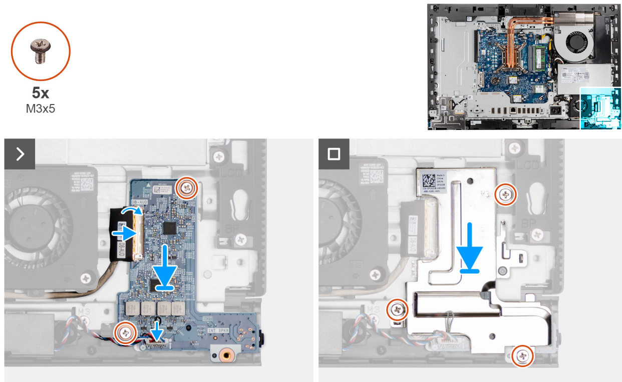
Rysunek 74. Instalowanie karty dźwiękowej
