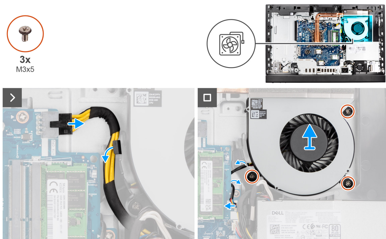
Rysunek 51. Wymontowywanie wentylatora
