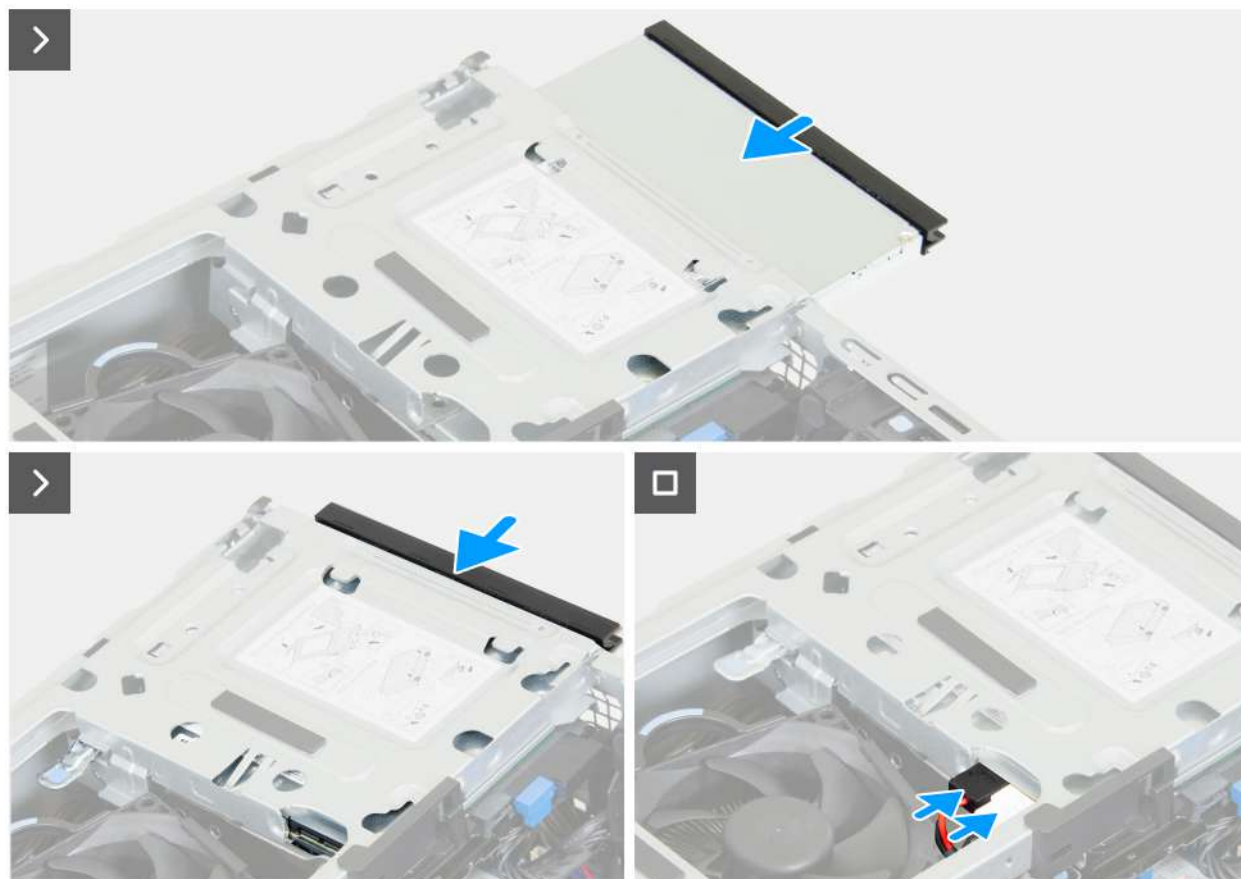
Rysunek 48. Instalowanie napędu optycznego
