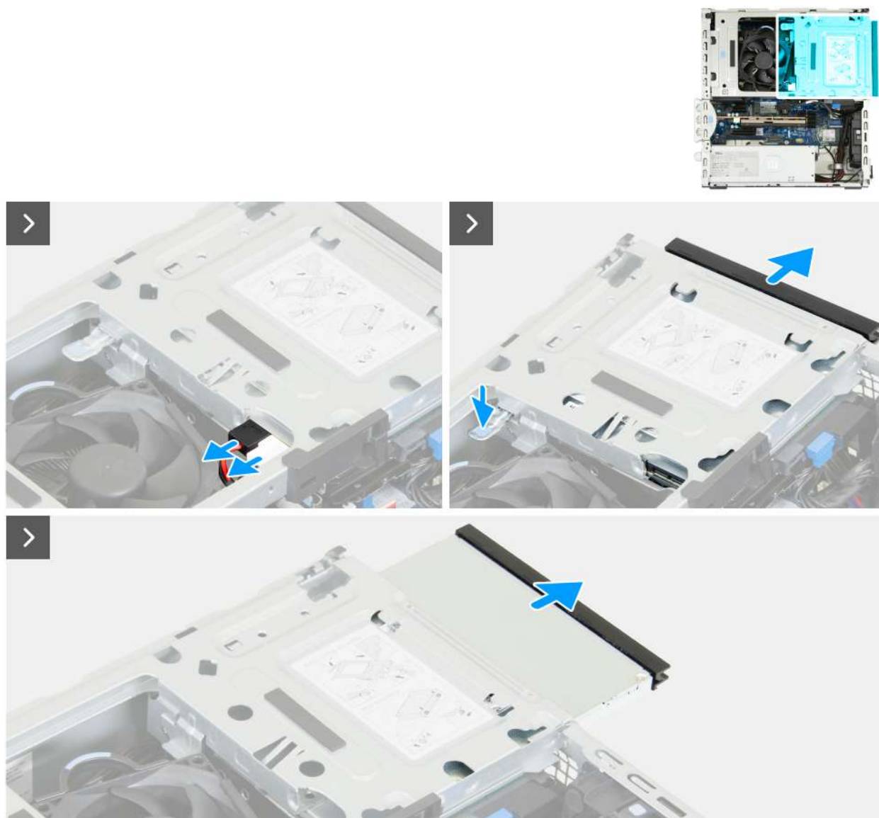
Rysunek 45. Wymontowywanie napędu optycznego
