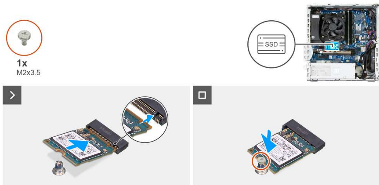
Rysunek 28. Instalowanie dysku SSD M.2 2230 w gnieździe 1
