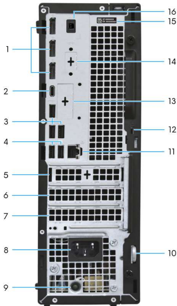
Rysunek 2. Widok z tyłu komputera Dell Pro Slim Plus QBS1250
