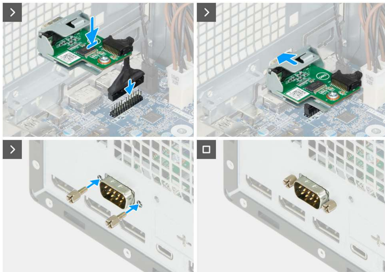
Rysunek 65. Instalowanie modułu portu szeregowego
