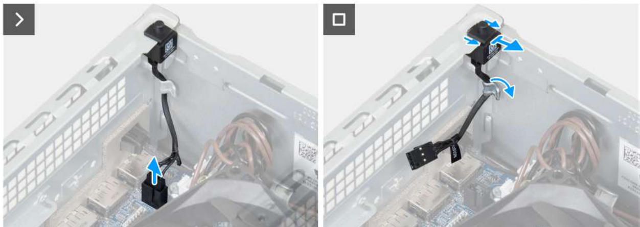
Rysunek 55. Wymontowywanie czujnika otwarcia obudowy
