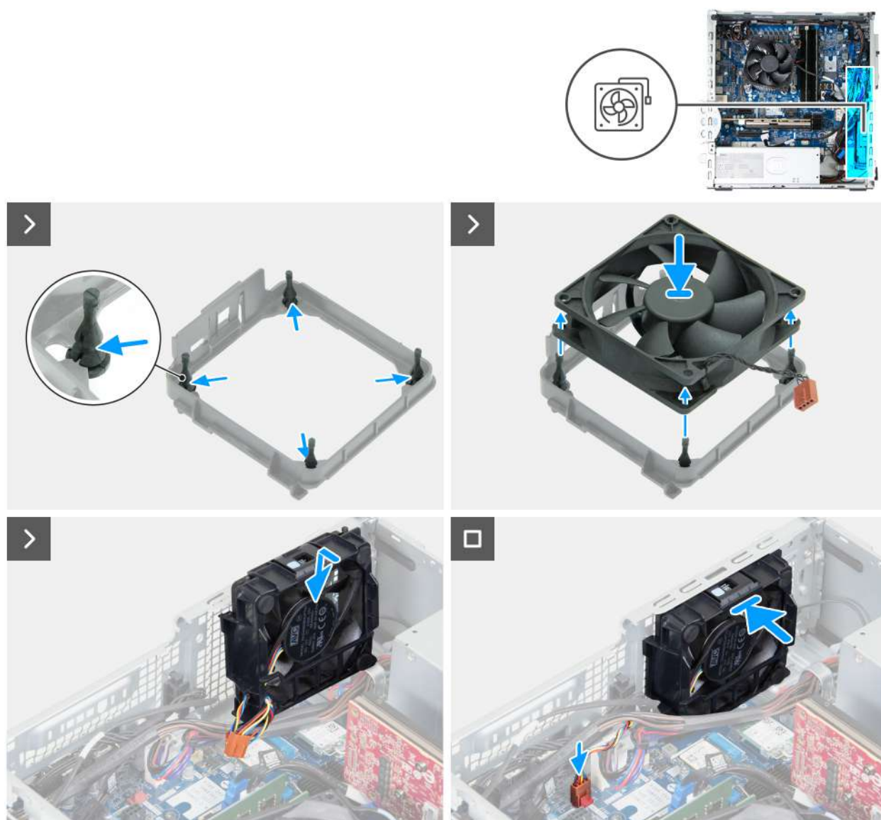
Rysunek 58. Instalowanie wentylatora
