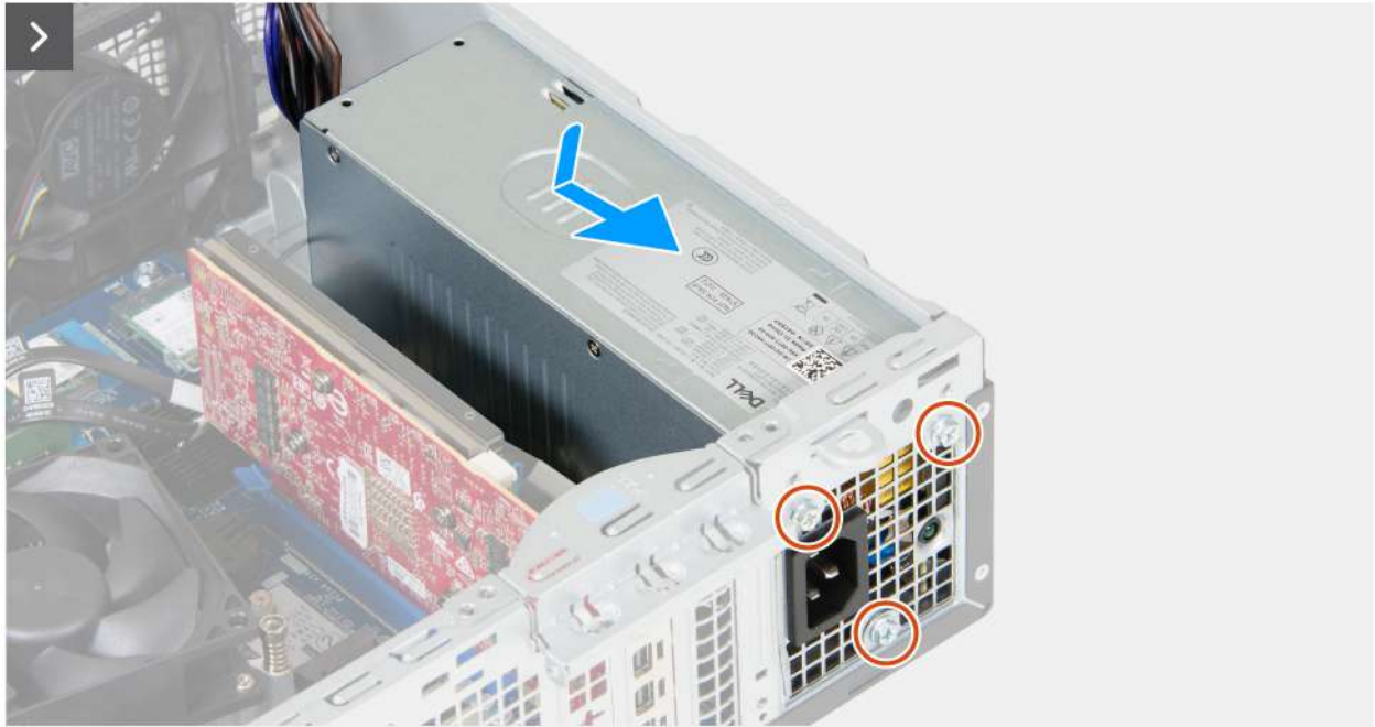
Rysunek 72. Instalowanie zasilacza
