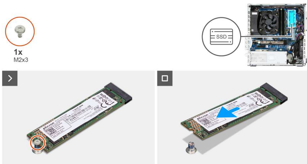
Rysunek 31. Wymontowywanie dysku SSD M.2 2280 z gniazda 2
