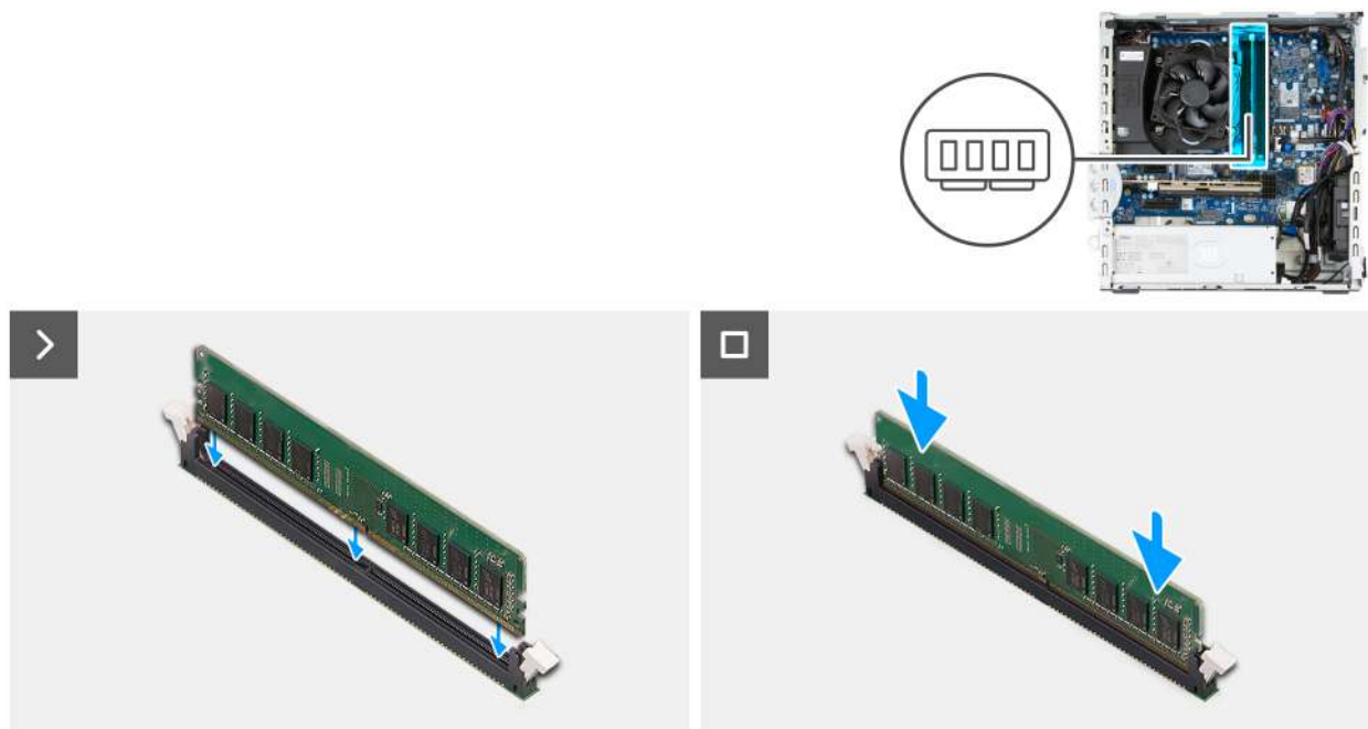
Rysunek 21. Instalowanie modułów pamięci
