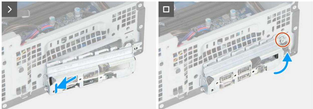
Rysunek 95. Instalowanie płyty głównej
