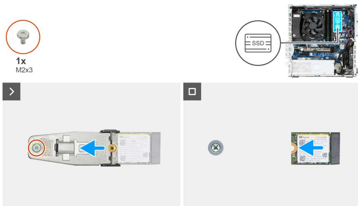
Rysunek 29. Wymontowywanie dysku SSD M.2 2230 z gniazda 2
