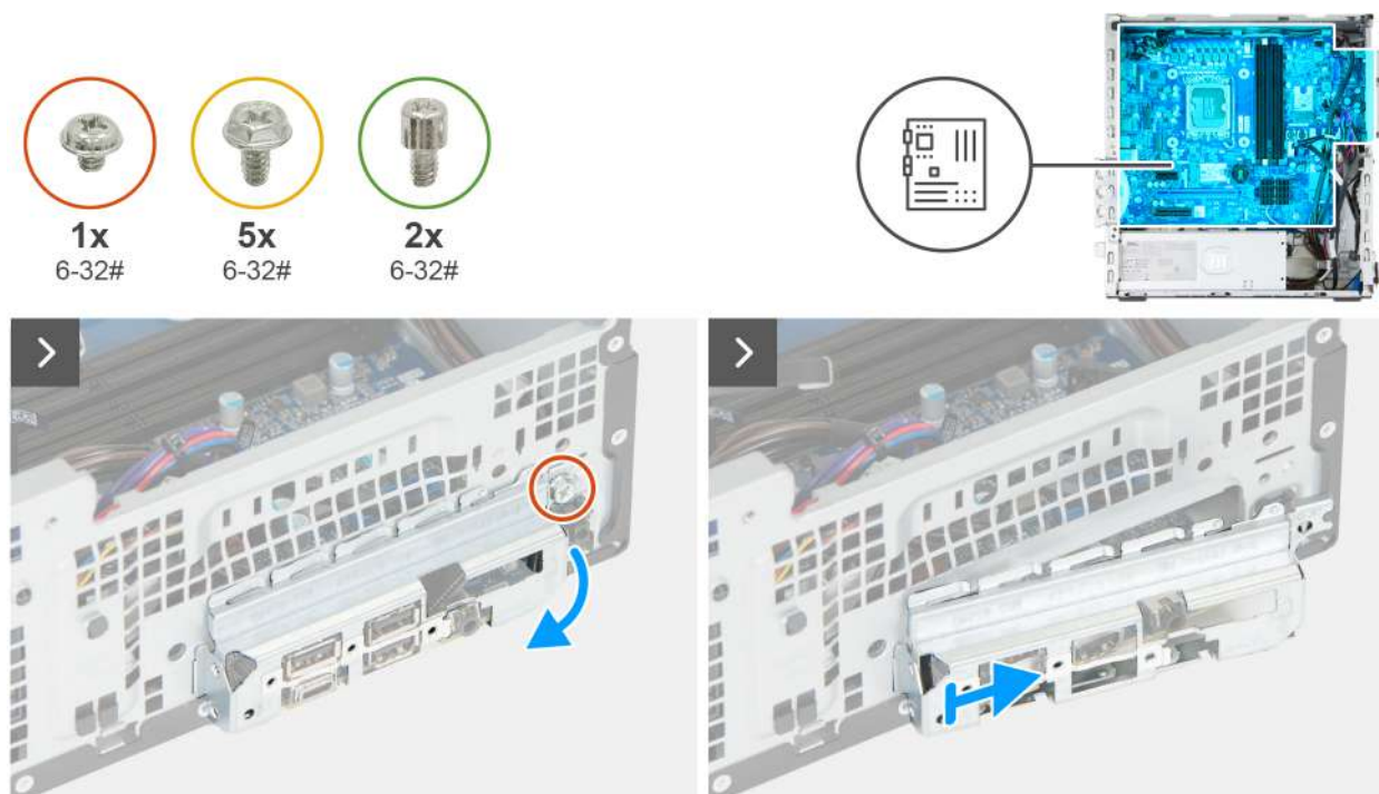
Rysunek 87. Wymontowywanie płyty systemowej
