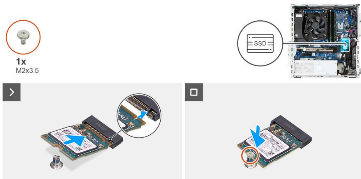
Rysunek 23. Instalowanie dysku SSD M.2 2230 w gnieździe 0
