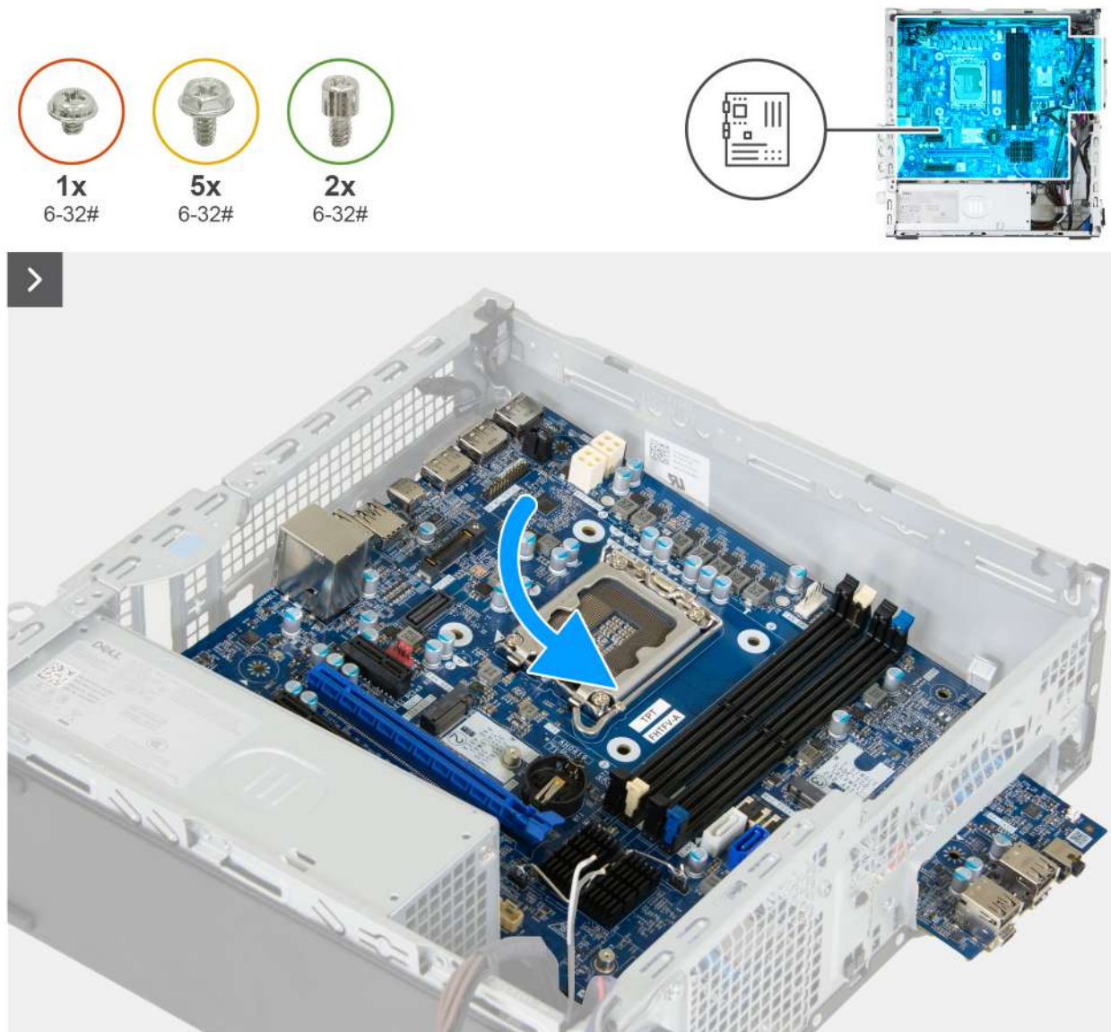
Rysunek 92. Instalowanie płyty głównej
