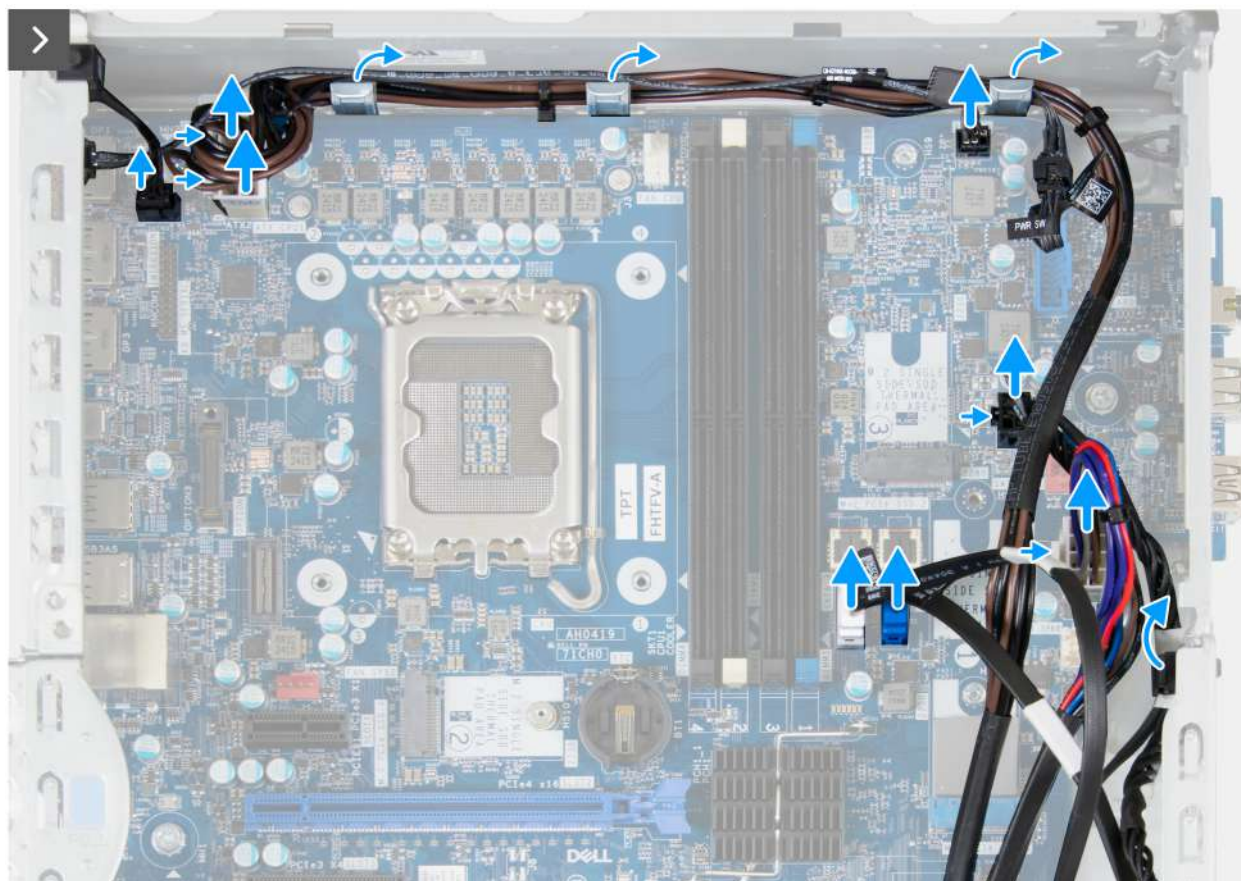
Rysunek 89. Wymontowywanie płyty systemowej
