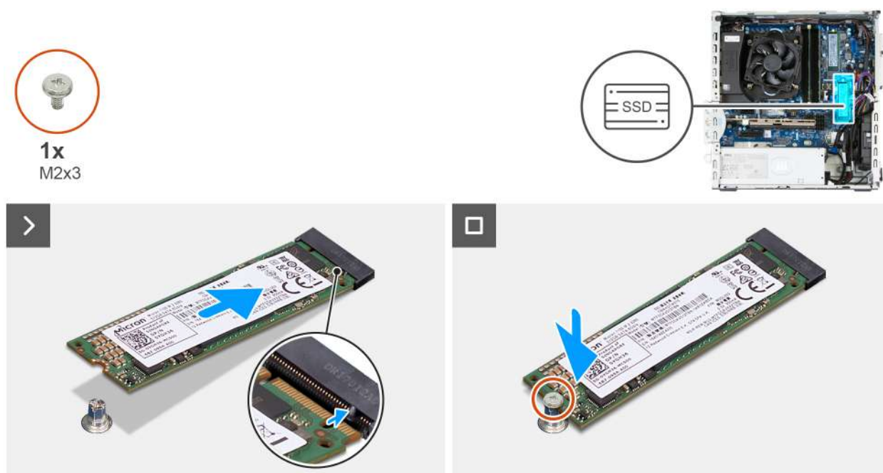
Rysunek 25. Instalowanie dysku SSD M.2 2280 w gnieździe 0
