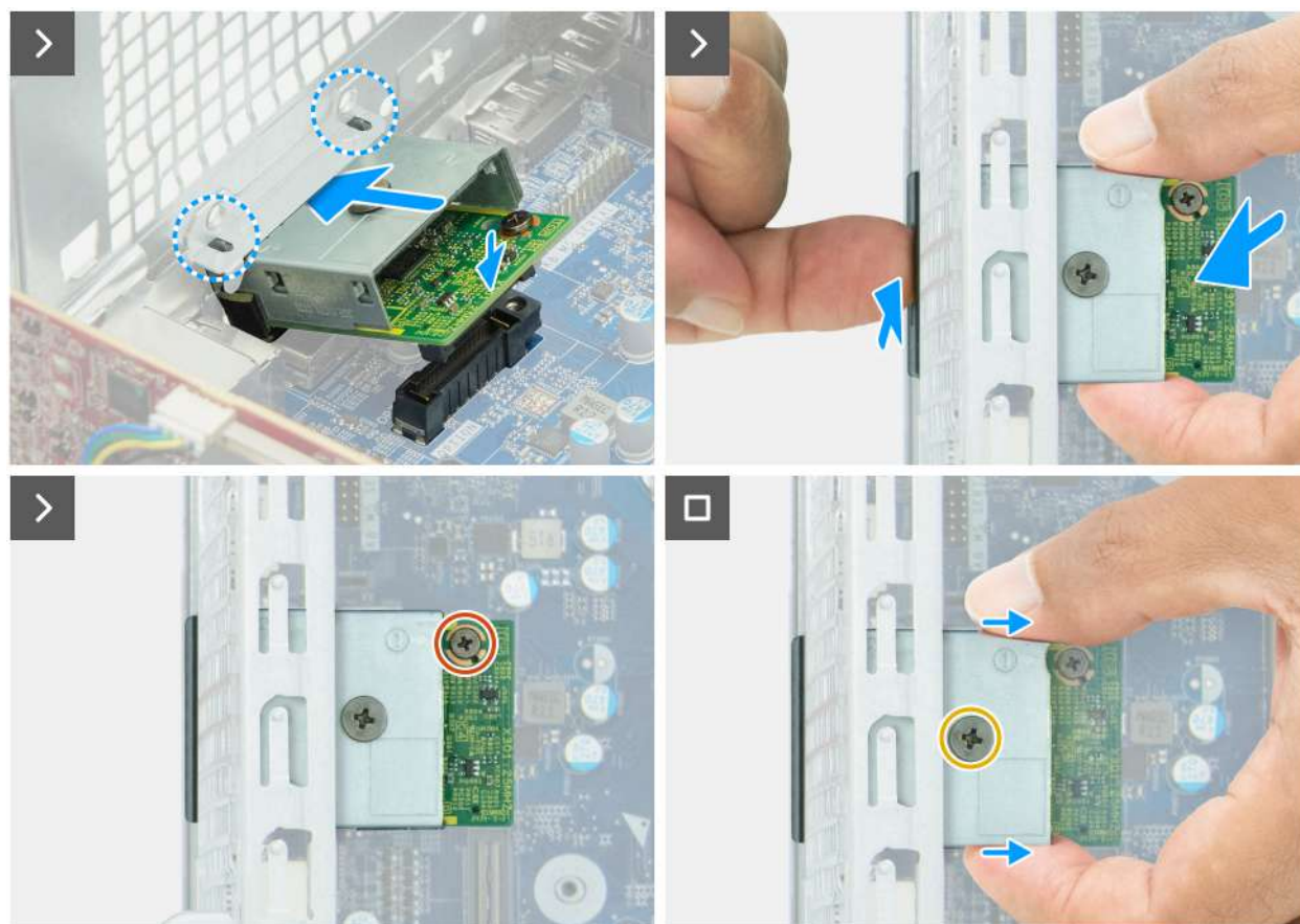
Rysunek 80. Instalowanie modułu opcjonalnego portu
