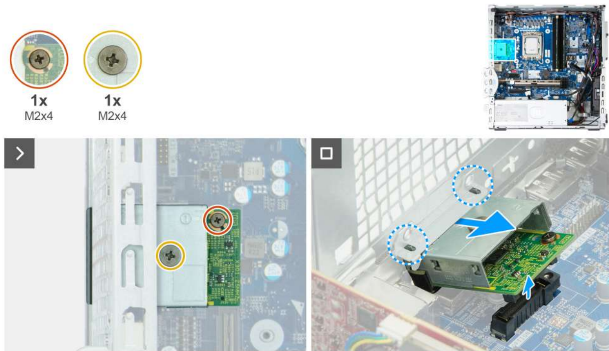
Rysunek 78. Wymontowywanie modułu z opcjonalnym portem
