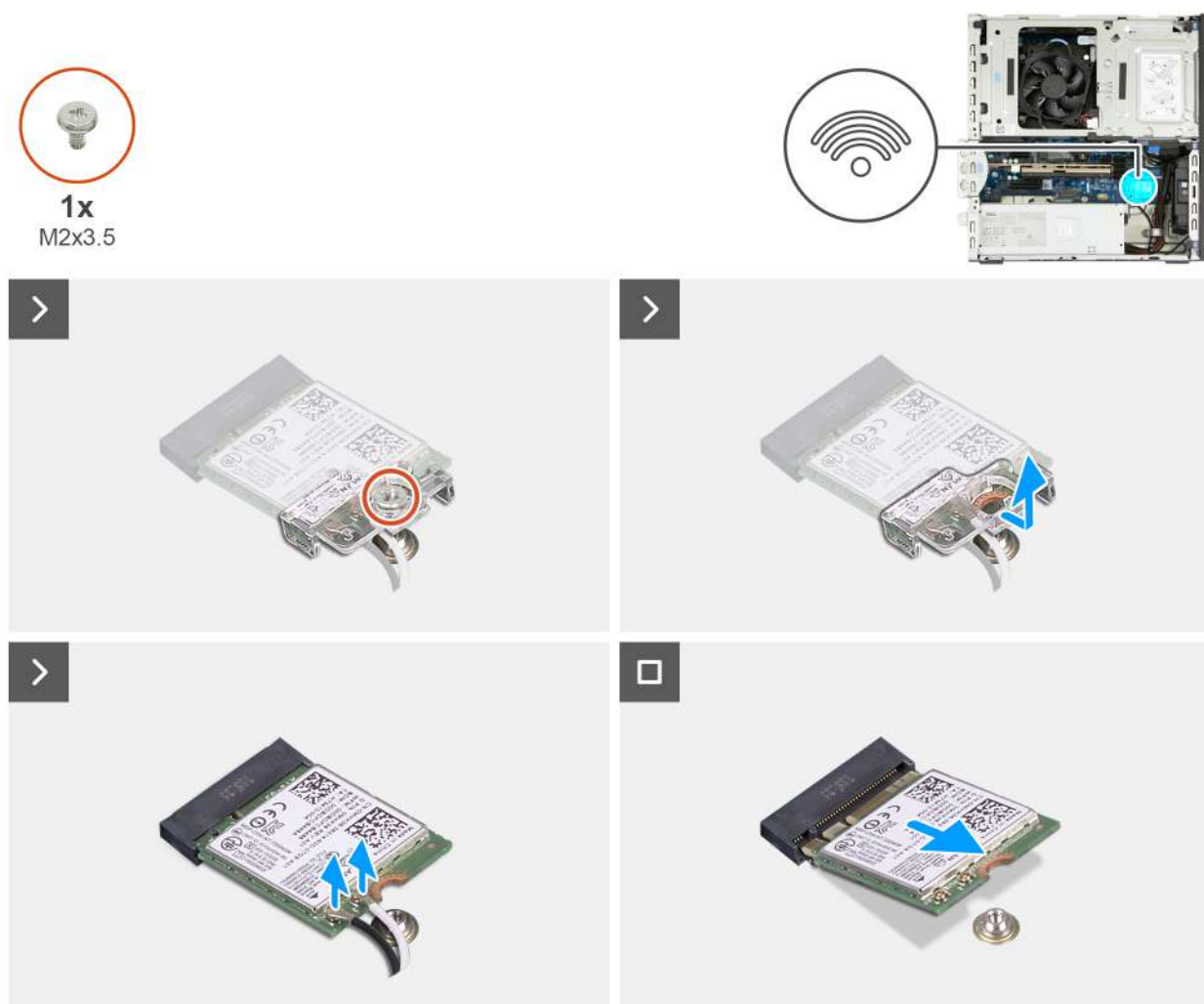
Rysunek 35. Wymontowywanie karty sieci bezprzewodowej
