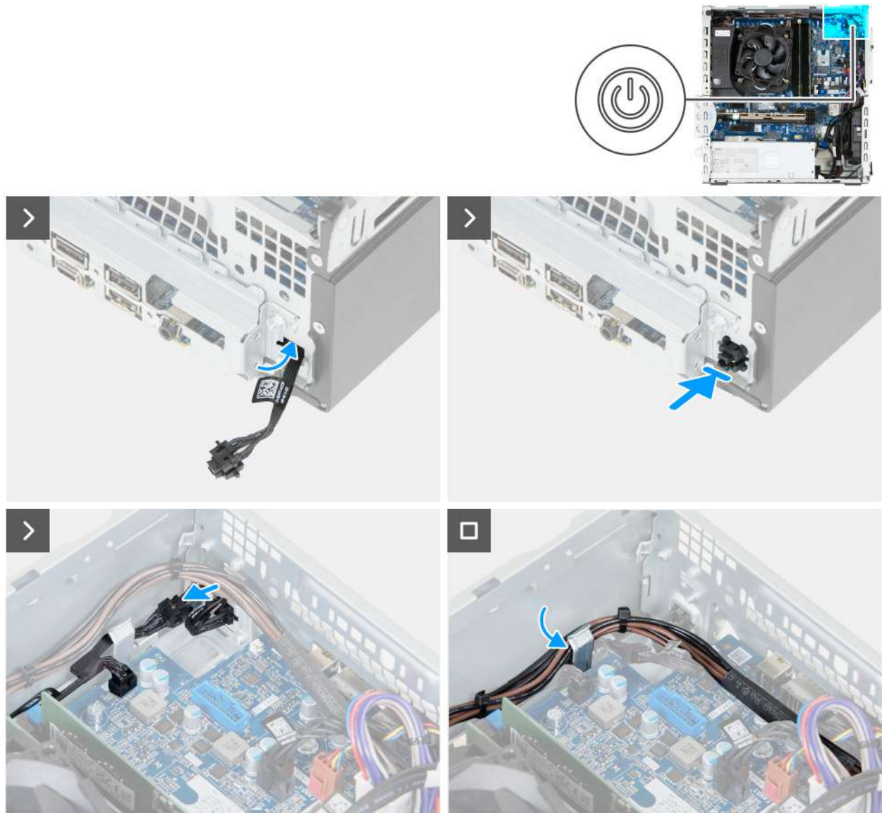
Rysunek 63. Instalowanie przycisku zasilania
