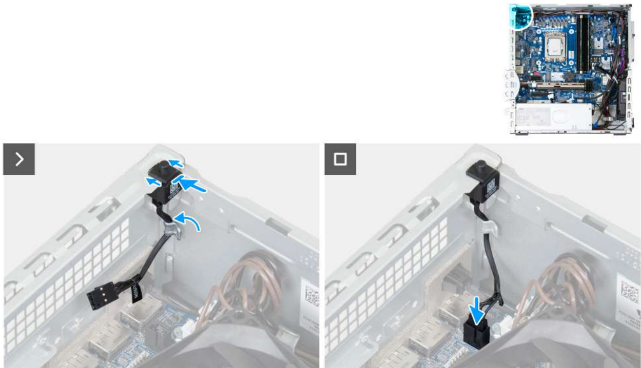
Rysunek 56. Instalowanie czujnika naruszenia obudowy
