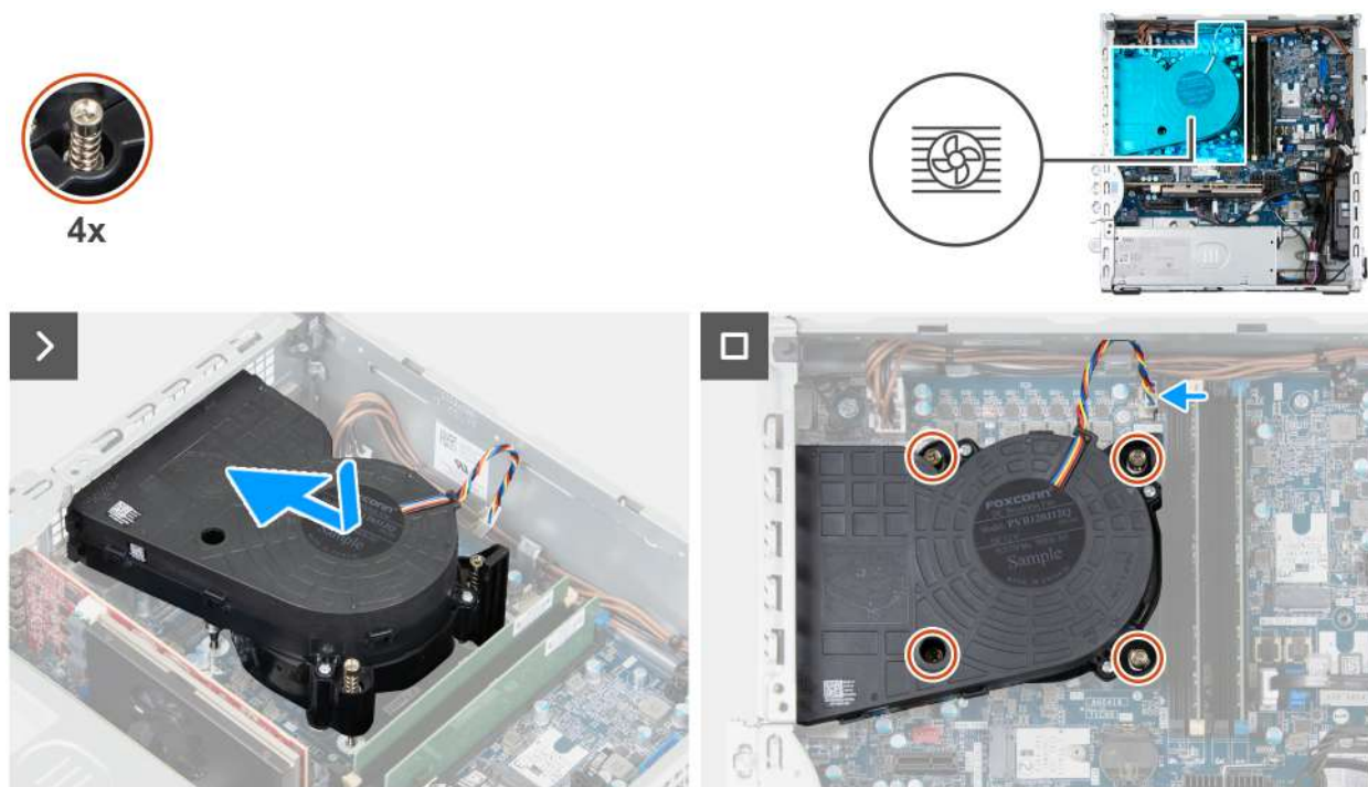
Rysunek 76. Instalowanie zestawu wentylatora i radiatora procesora (Dell Pro Slim Plus QBS1250)
