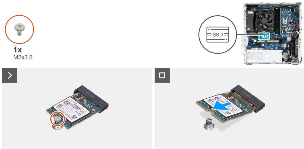
Rysunek 27. Wymontowywanie dysku SSD M.2 2230 z gniazda 1
