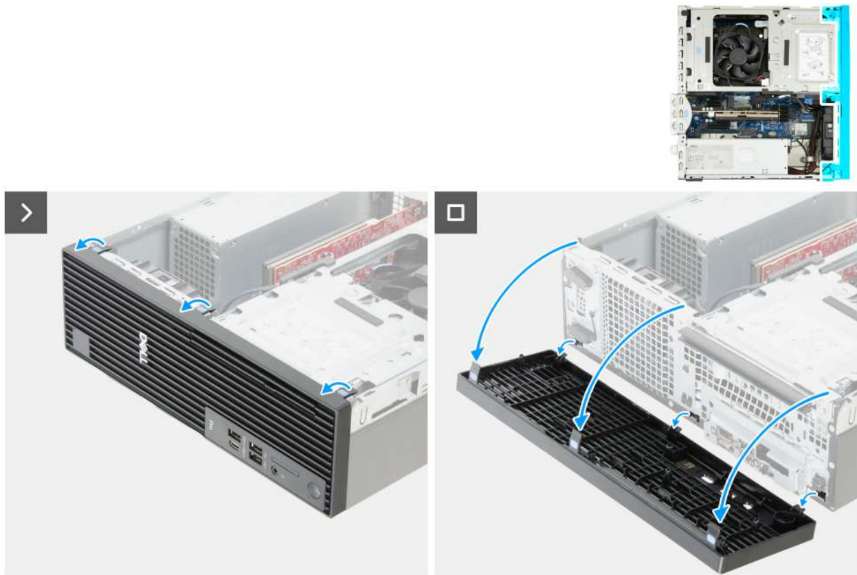
Rysunek 16. Wymontowywanie pokrywki przedniej
