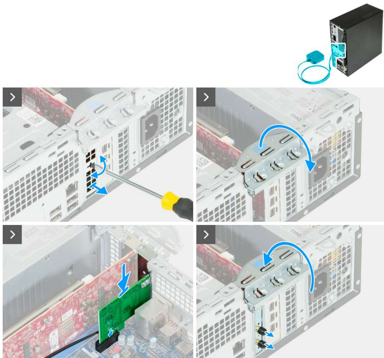
Rysunek 43. Instalowanie karty rozszerzenia anteny krążkowej
