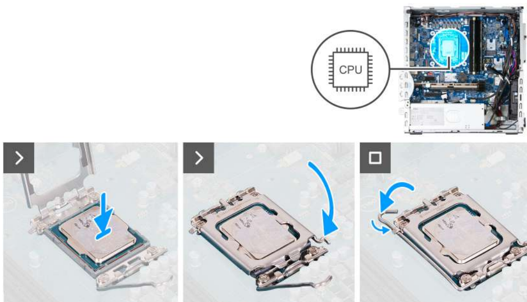
Rysunek 85. Instalowanie procesora
