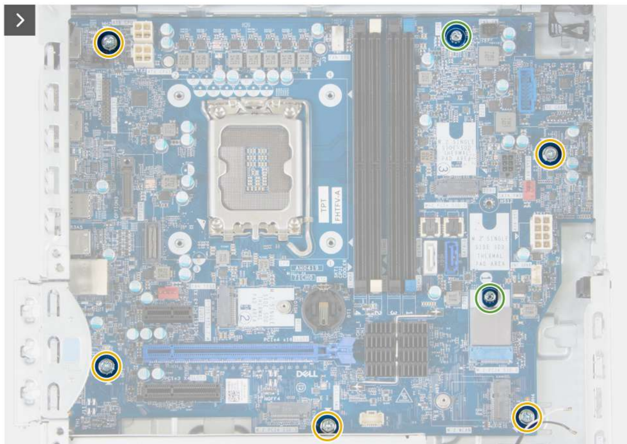
Rysunek 88. Wymontowywanie płyty systemowej
