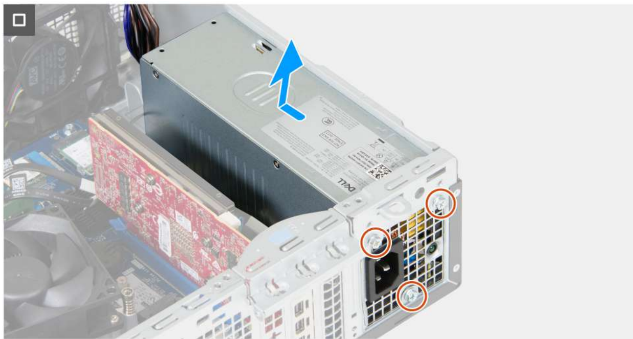
Rysunek 71. Instalowanie zasilacza
