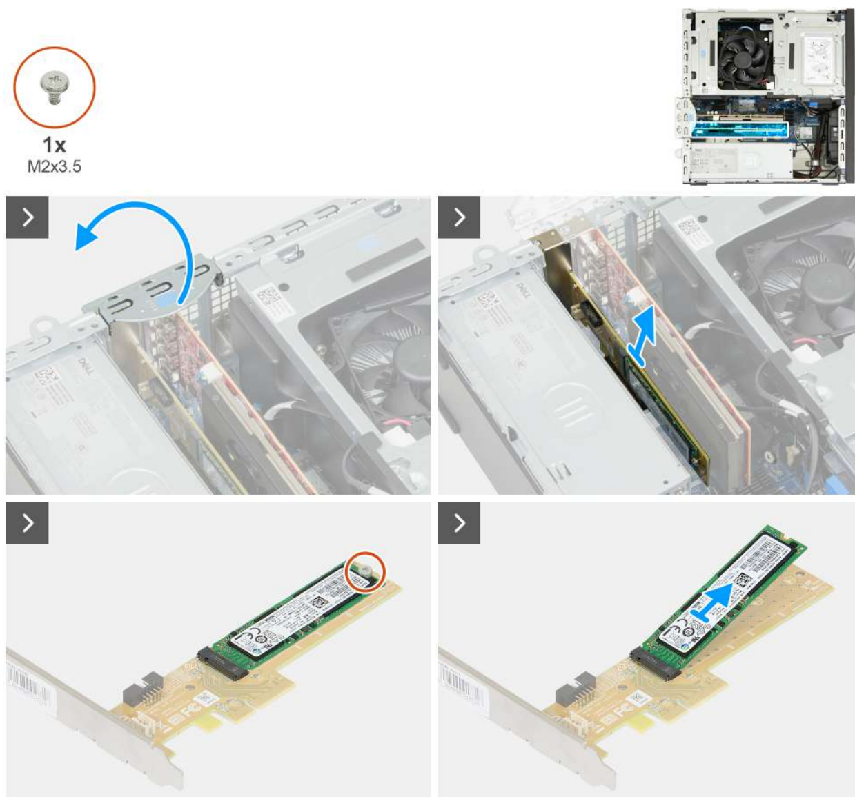
Rysunek 37. Wymontowywanie karty rozszerzeń SSD
