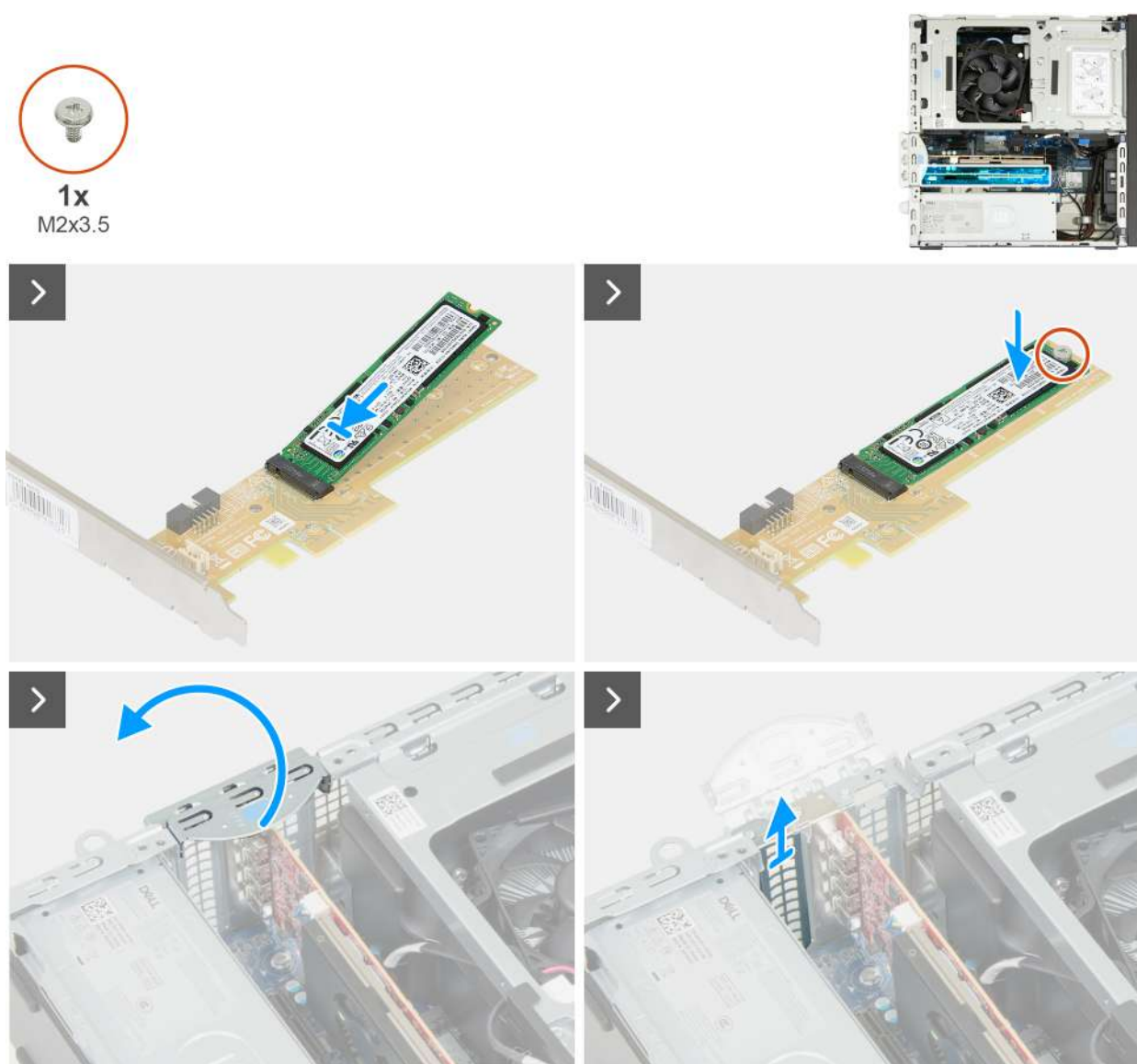
Rysunek 39. Instalowanie karty rozszerzeń SSD
