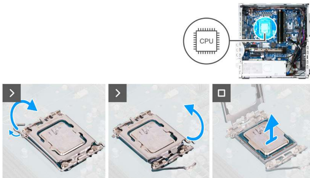
Rysunek 84. Wymontowywanie procesora
