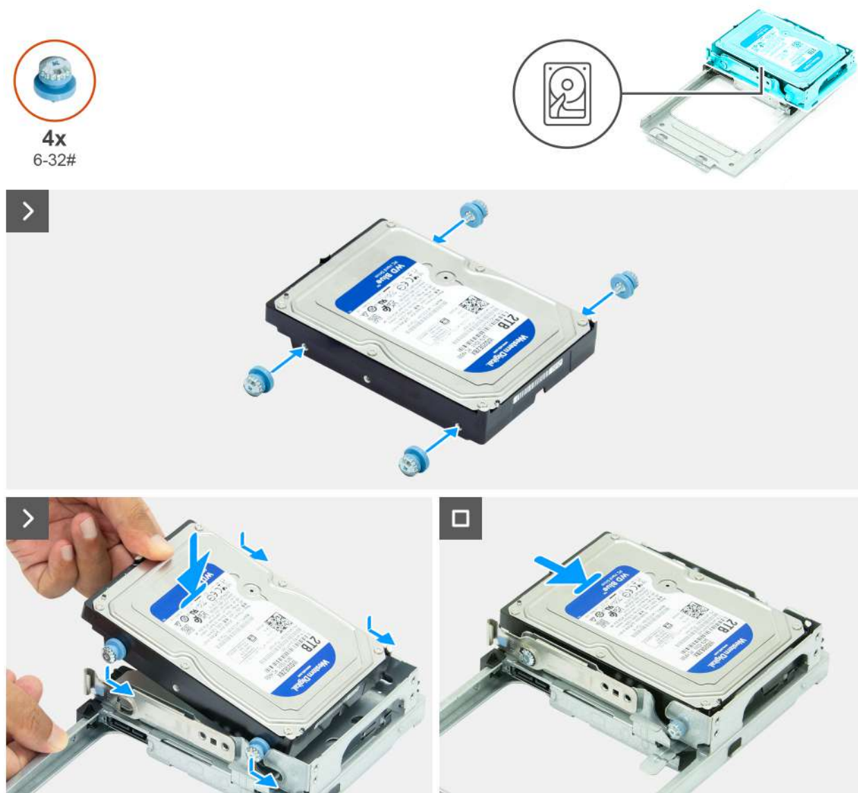
Rysunek 54. Instalowanie dysku twardego
