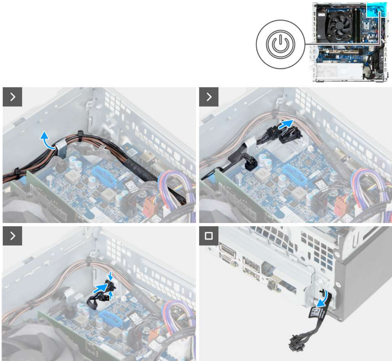
Rysunek 62. Wymontowywanie przycisku zasilania
