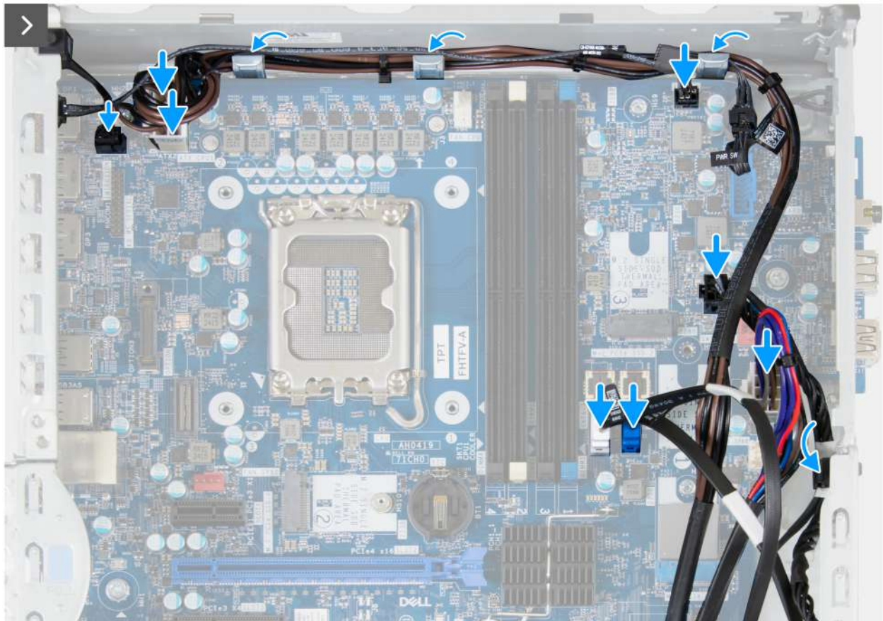
Rysunek 94. Instalowanie płyty głównej
