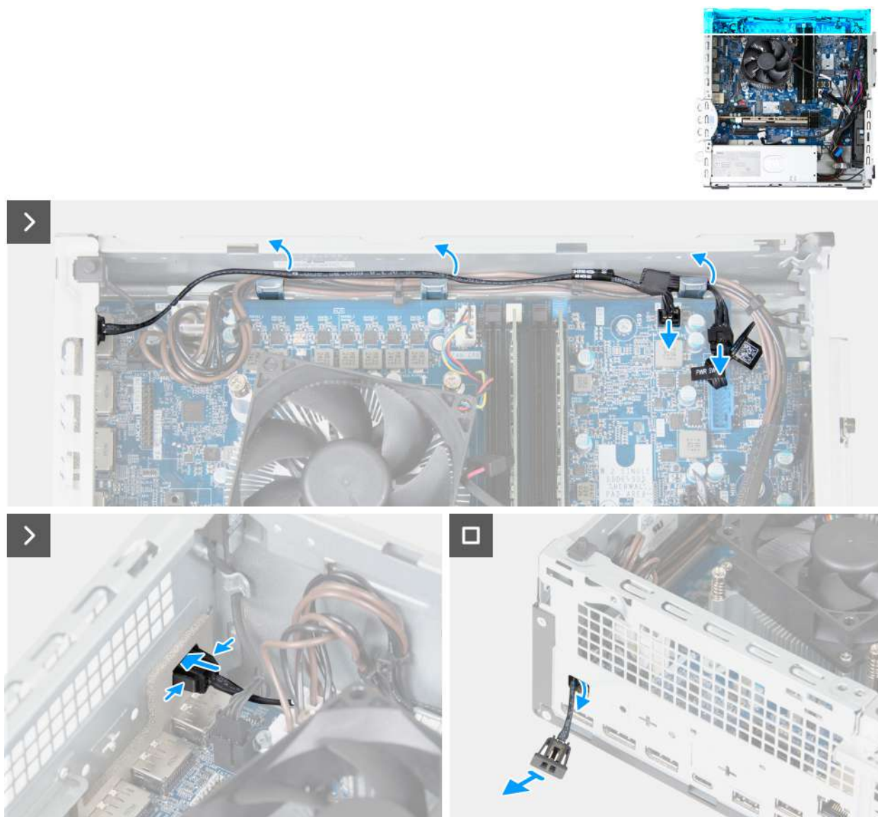
Rysunek 59. Wymontowywanie zdalnego przełącznika zasilania
