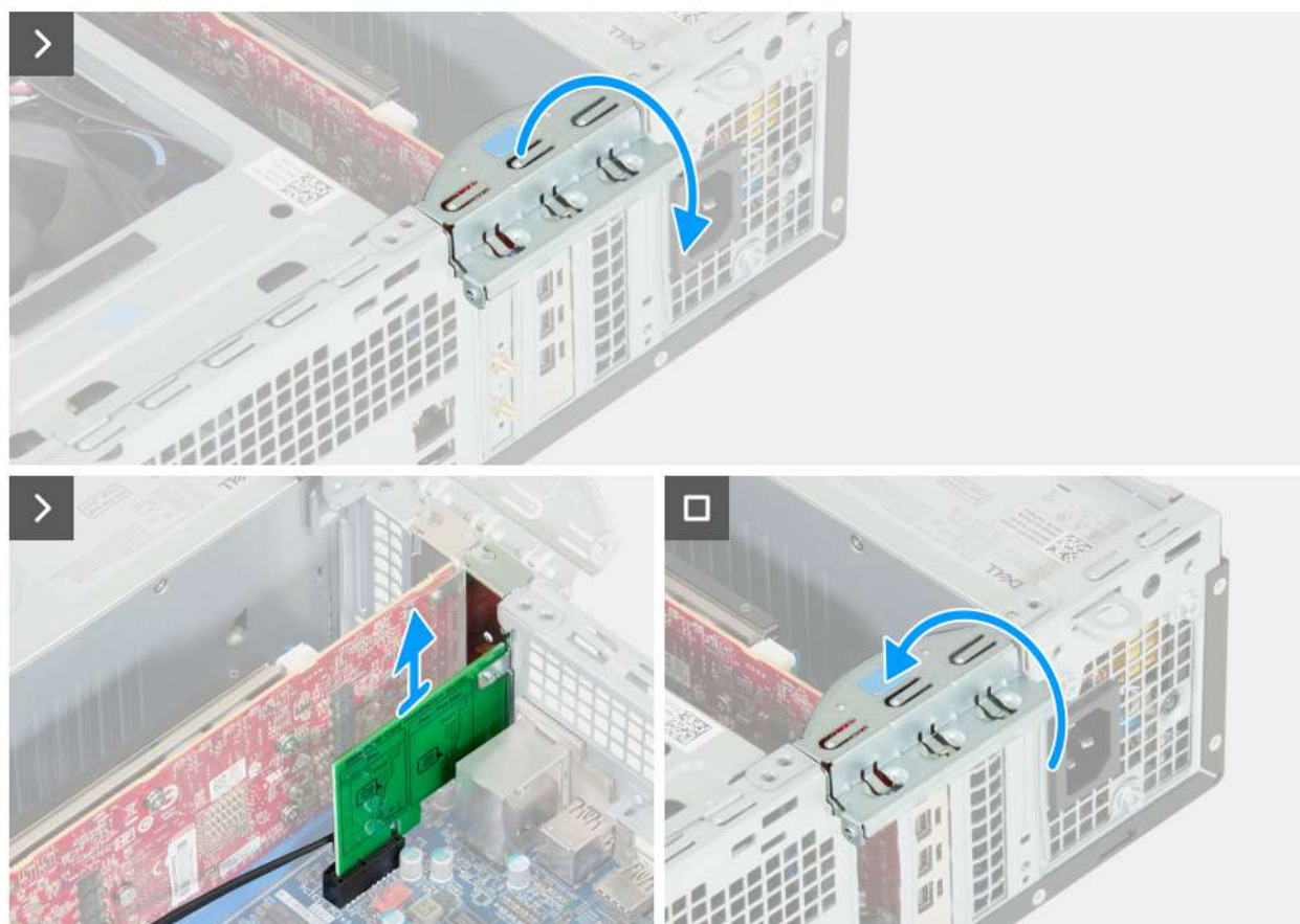
Rysunek 42. Wymontowywanie karty rozszerzenia anteny krążkowej
