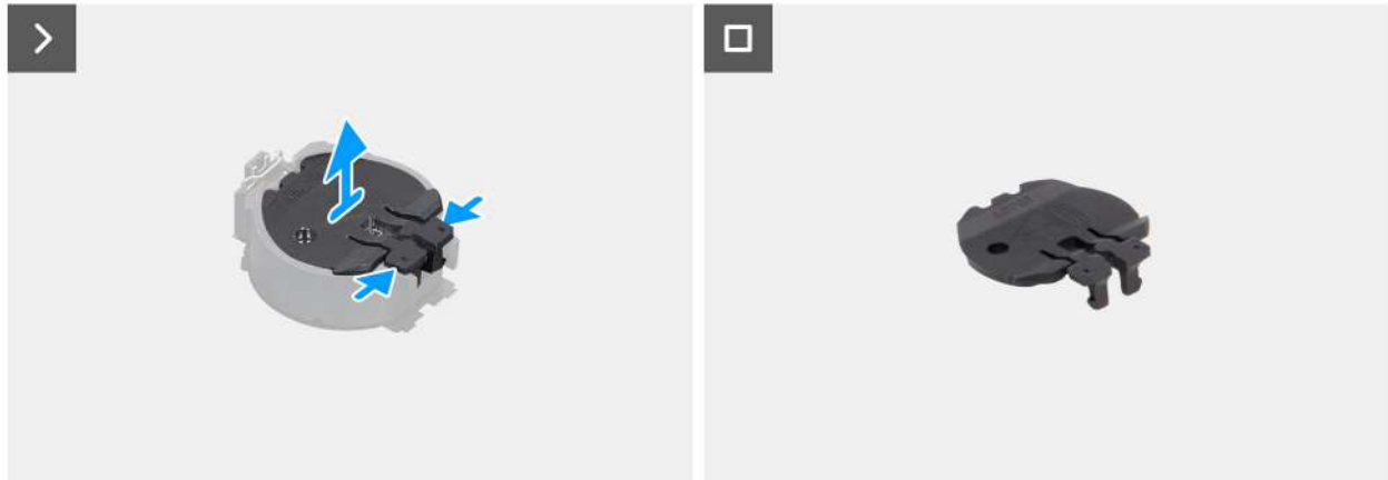
Rysunek 10. Wymontowywanie pokrywy baterii pastylkowej
