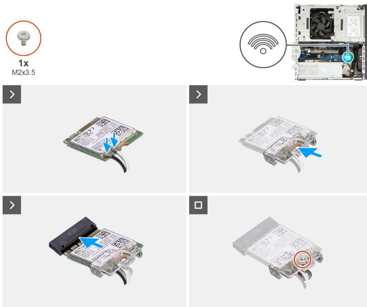
Rysunek 36. Instalowanie karty sieci bezprzewodowej
