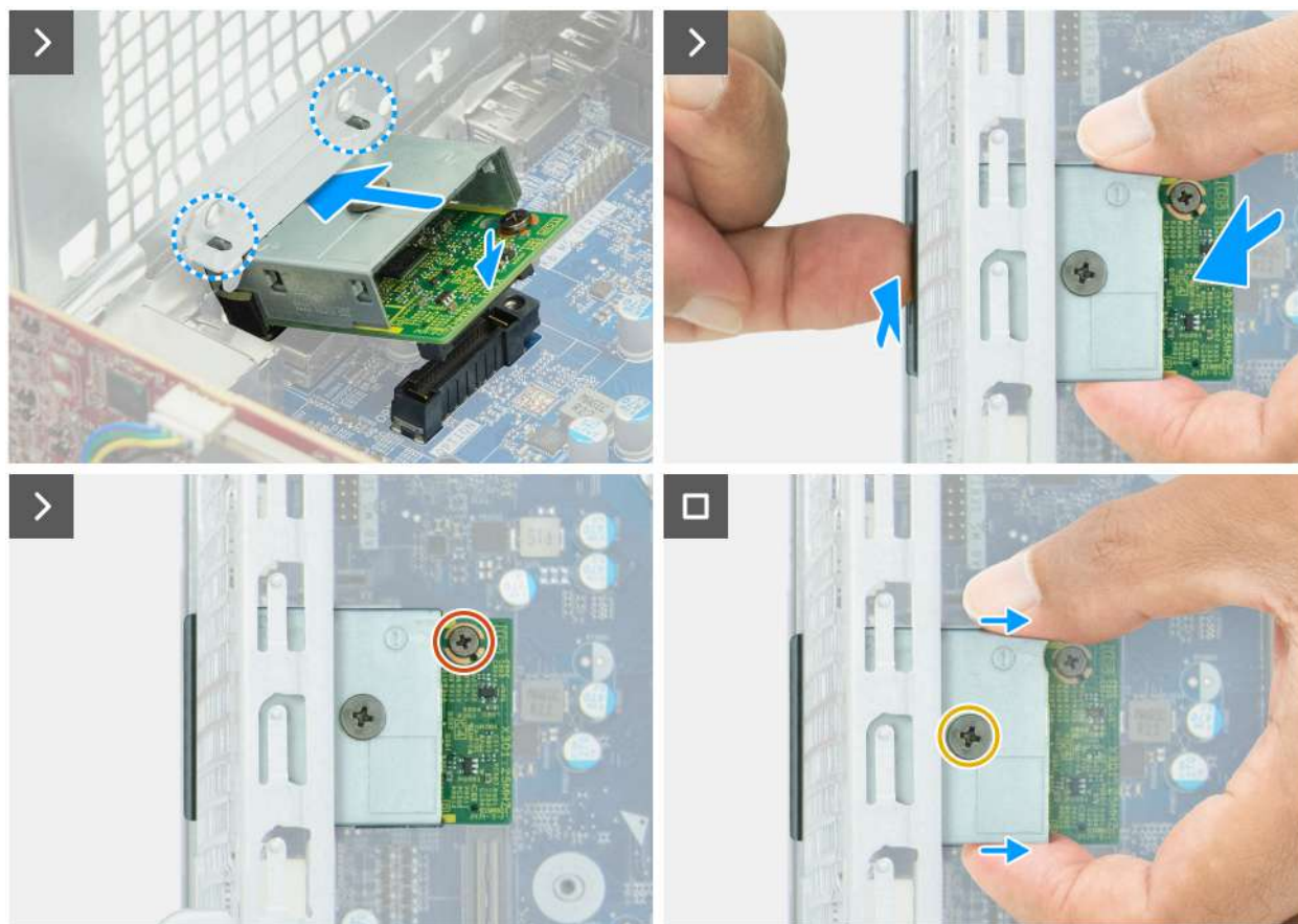
Rysunek 50. Instalowanie modułu portu opcjonalnego
