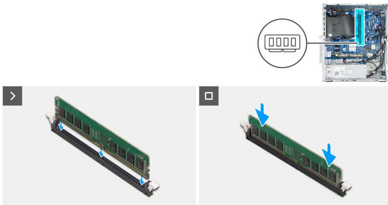
Rysunek 24. Instalowanie modułów pamięci
