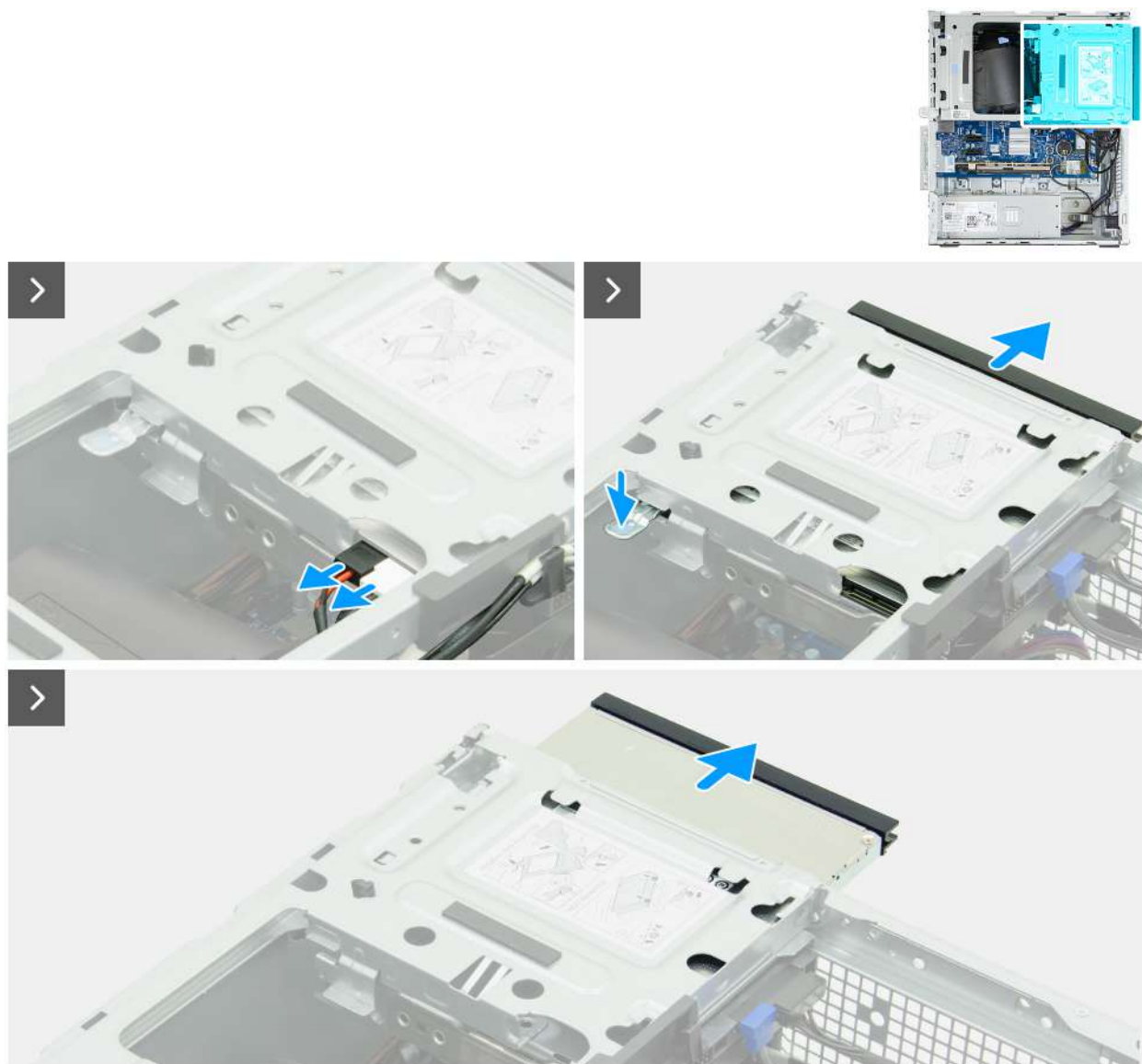
Rysunek 34. Wymontowywanie napędu optycznego
