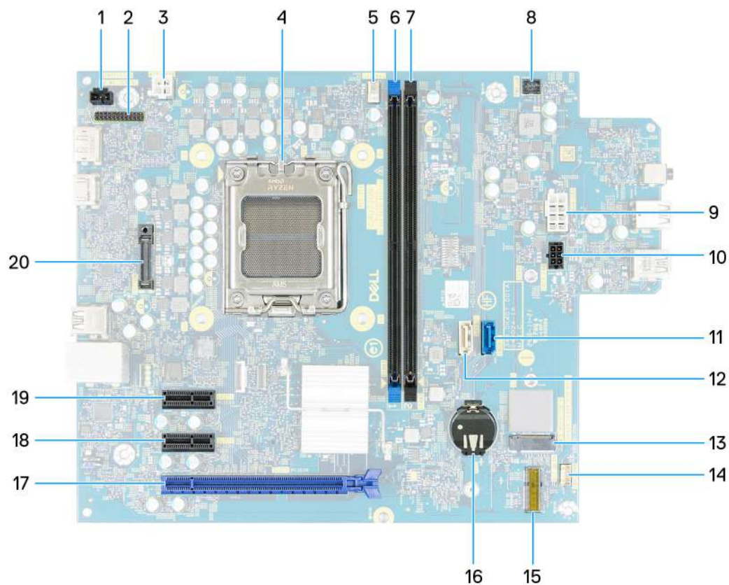
Rysunek 71. Elementy płyty głównej
