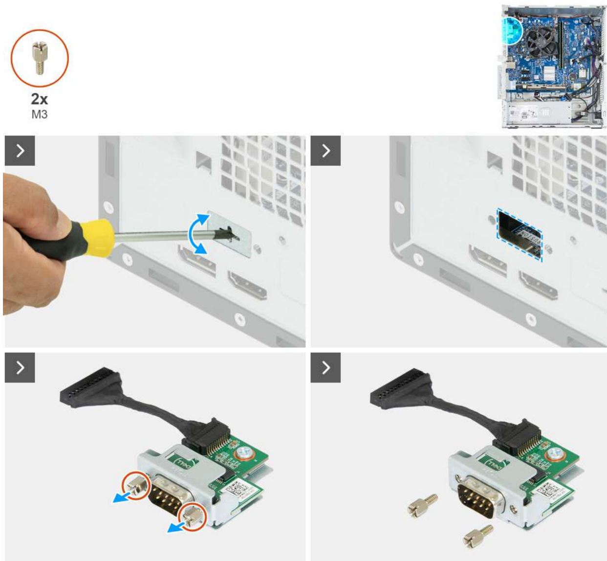
Rysunek 52. Instalowanie modułu portu szeregowego
