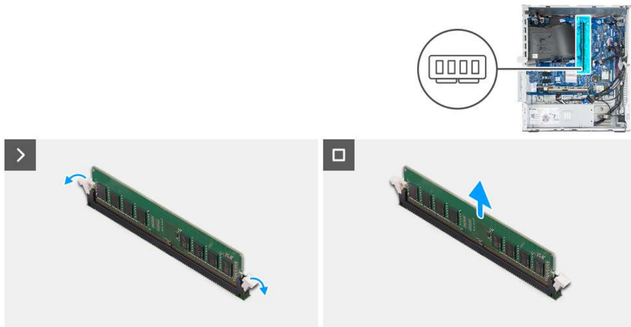
Rysunek 23. Wymontowywanie modułów pamięci
