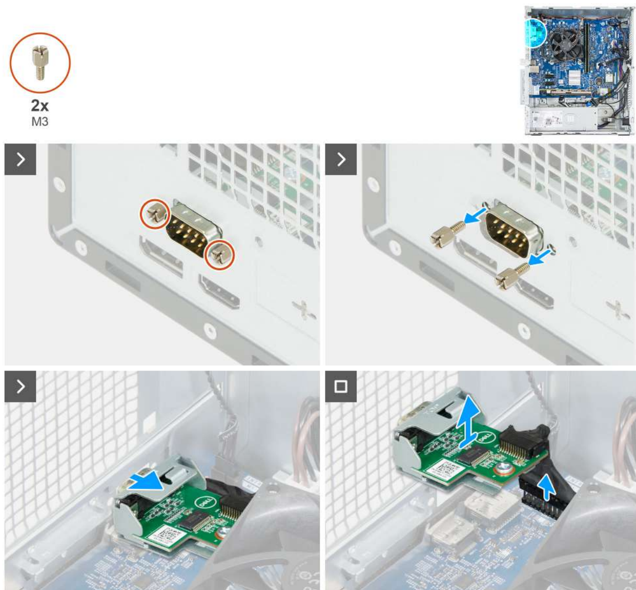
Rysunek 51. Wymontowywanie modułu portu szeregowego
