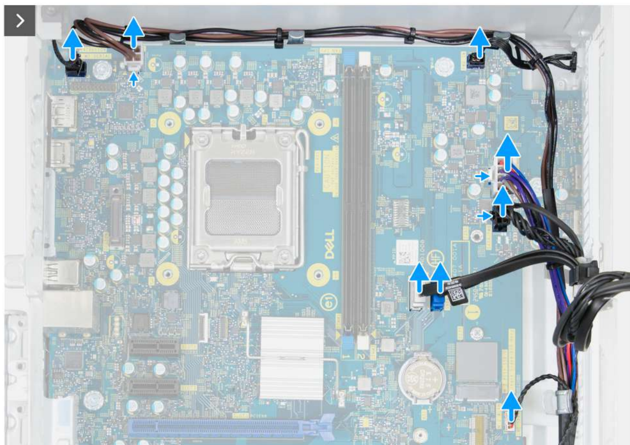
Rysunek 68. Wymontowywanie płyty głównej
