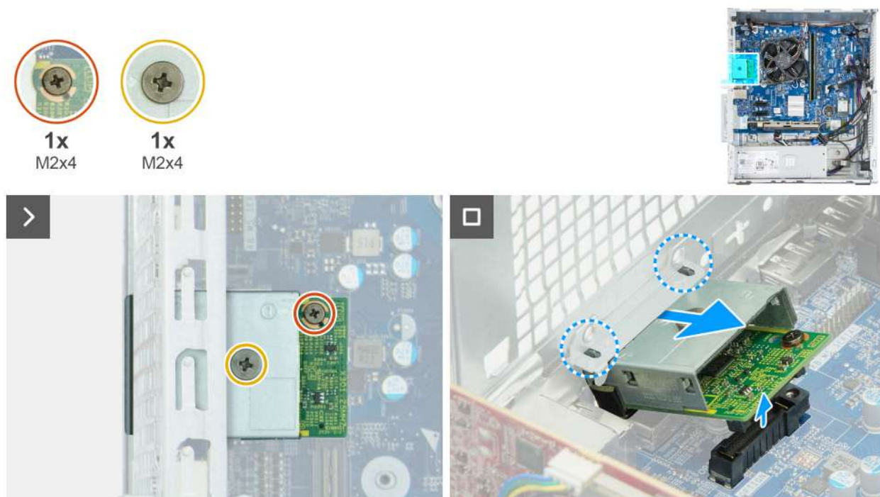
Rysunek 48. Wymontowywanie modułu portu opcjonalnego
