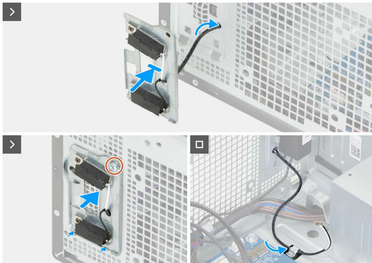
Rysunek 57. Instalowanie modułów anten
