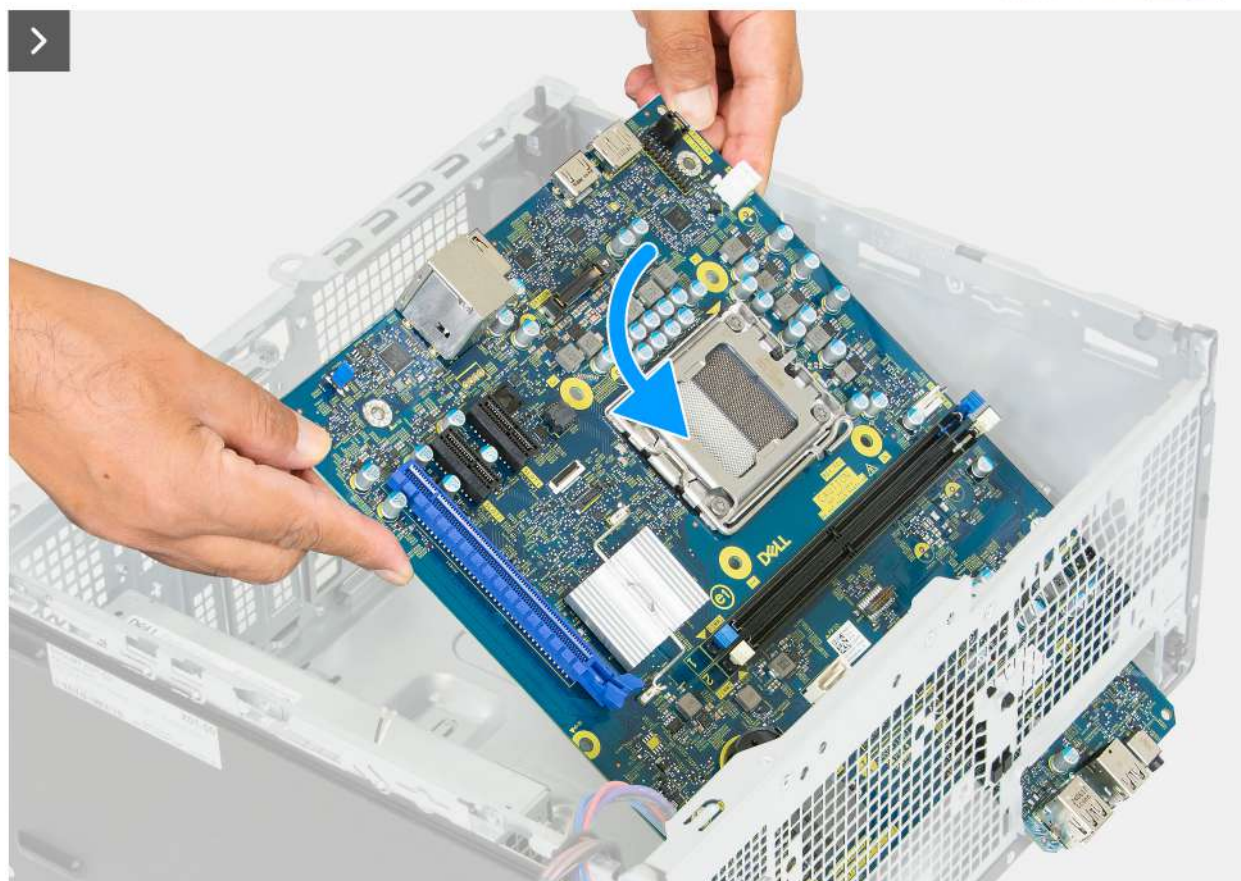
Rysunek 72. Instalowanie płyty głównej
