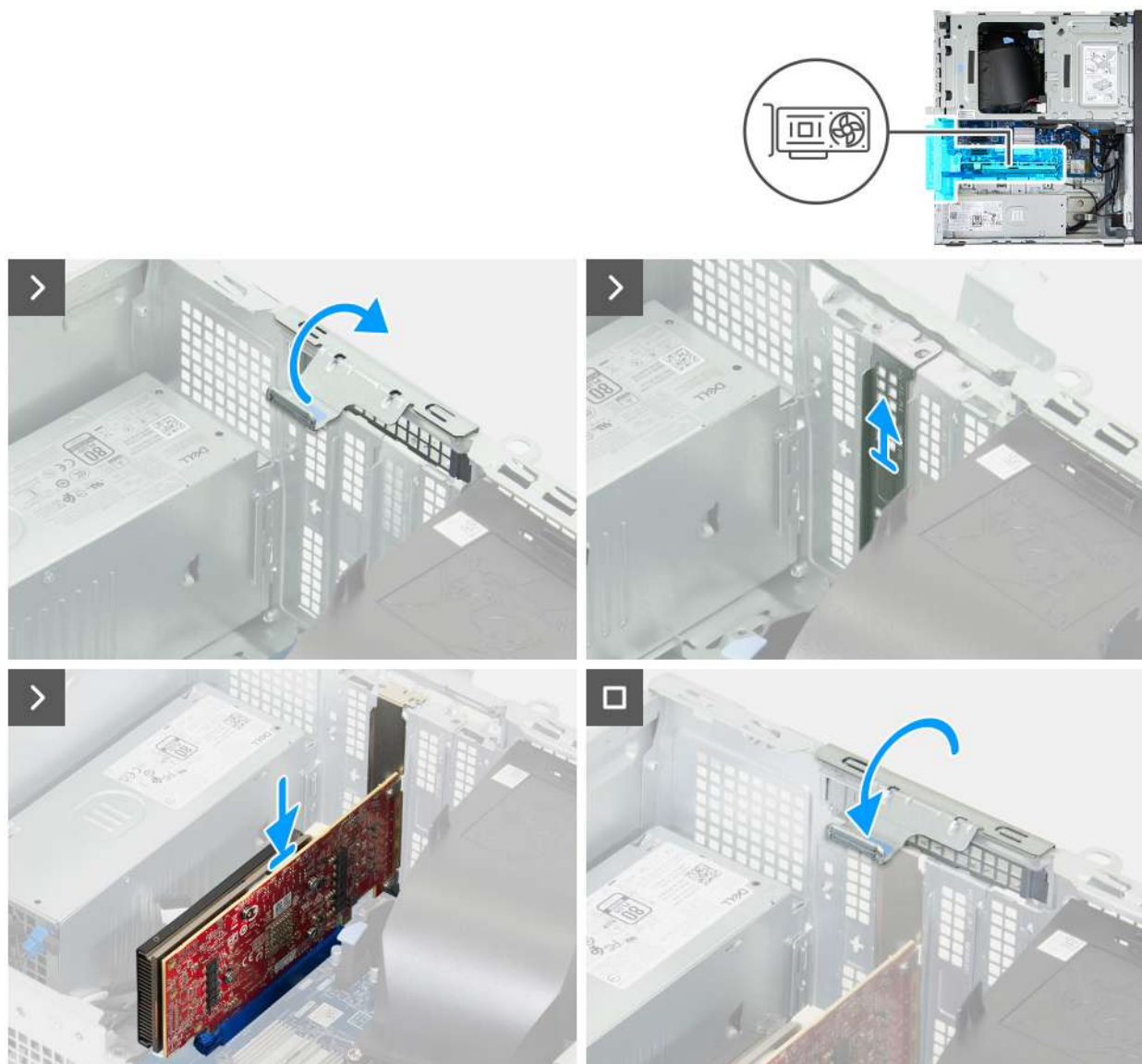
Rysunek 31. Instalowanie karty graficznej
