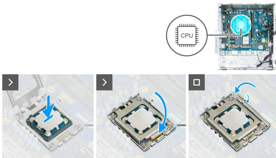
Rysunek 65. Instalowanie procesora
