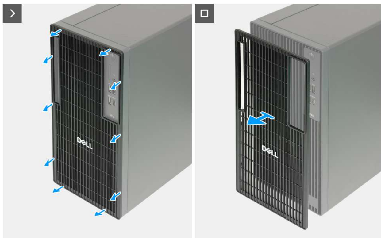
Rysunek 17. Wymontowywanie filtra przeciwpylowego
