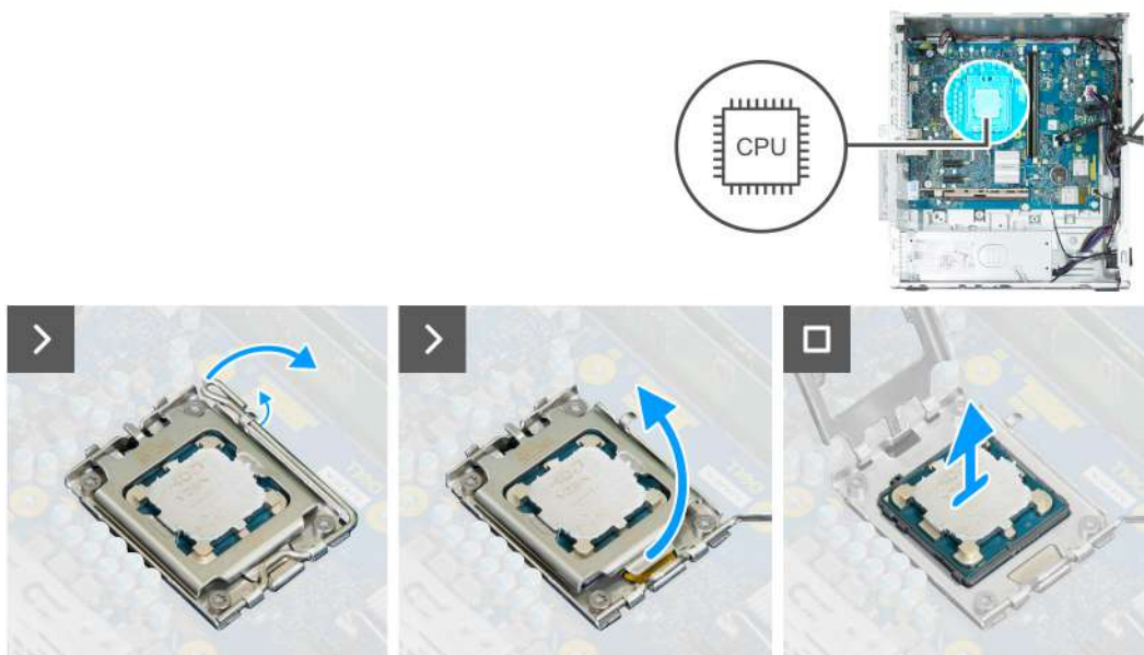
Rysunek 64. Wymontowywanie procesora
