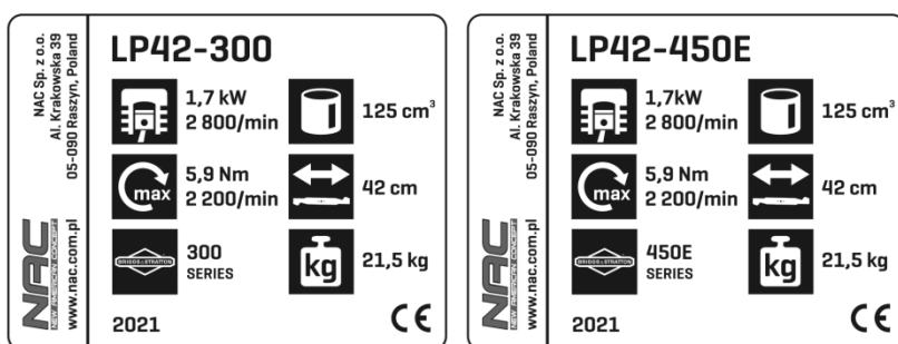
Tabliczka znamionowa
