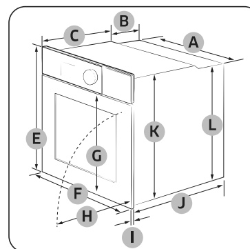
Piekarnik (mm)
