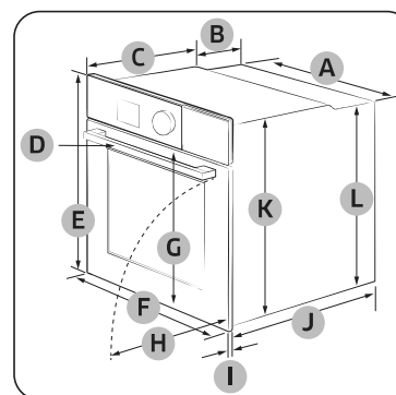
Piekarnik (mm)
