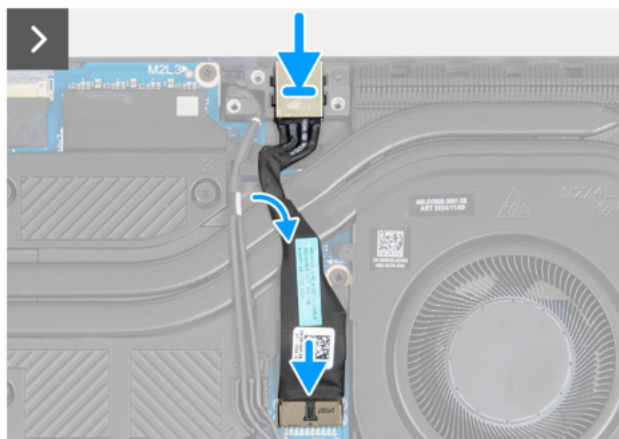
Rysunek 39. Instalowanie gniazda zasilacza
