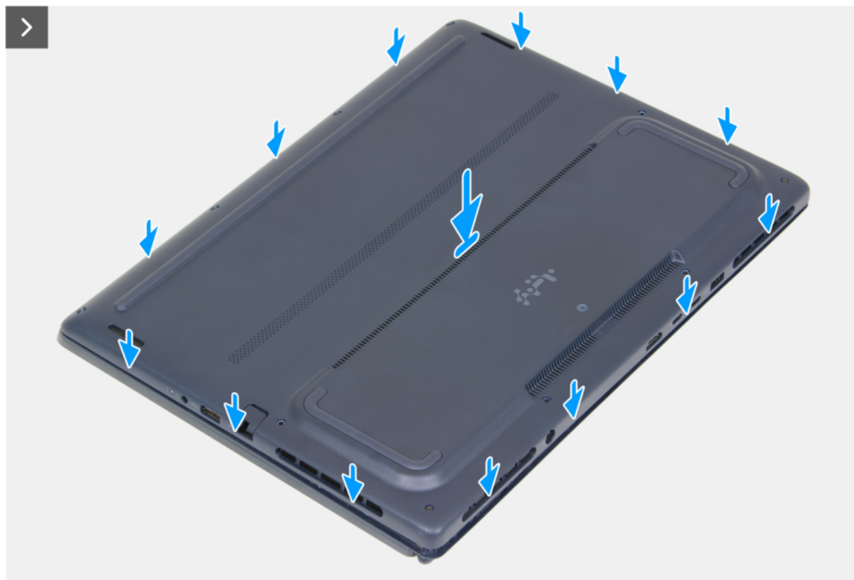
Rysunek 18. Instalowanie pokrywy dolnej
