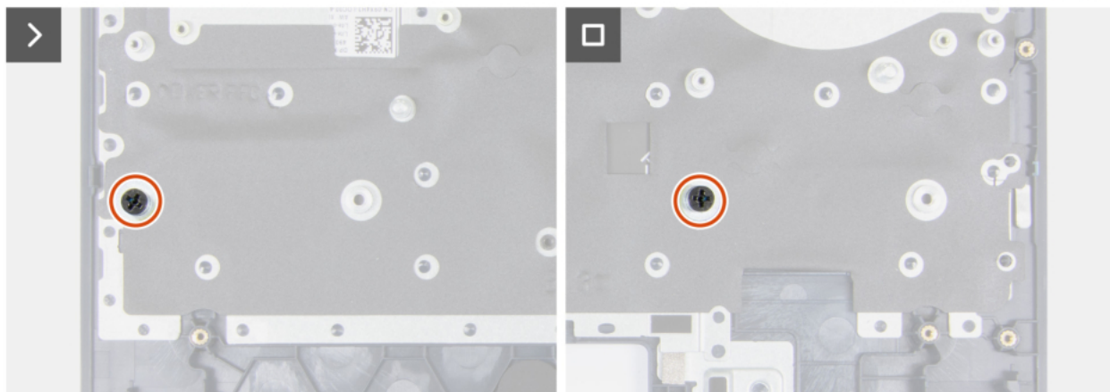
Rysunek 74. Wkręcanie uchwytów na śruby dysku SSD
