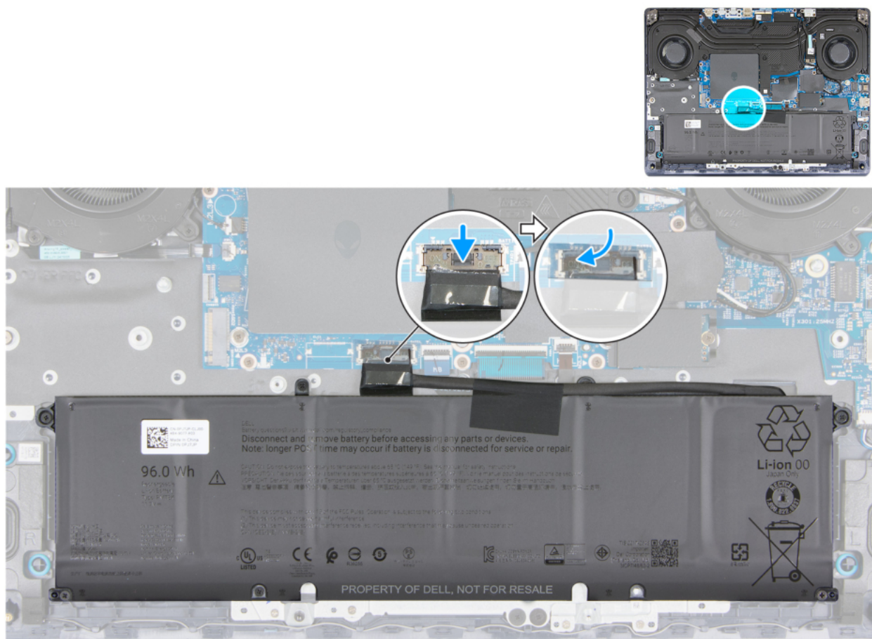
Rysunek 17. Podłączanie kabla baterii
