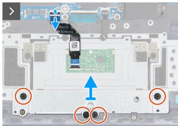
Rysunek 48. Wymontowywanie touchpada
