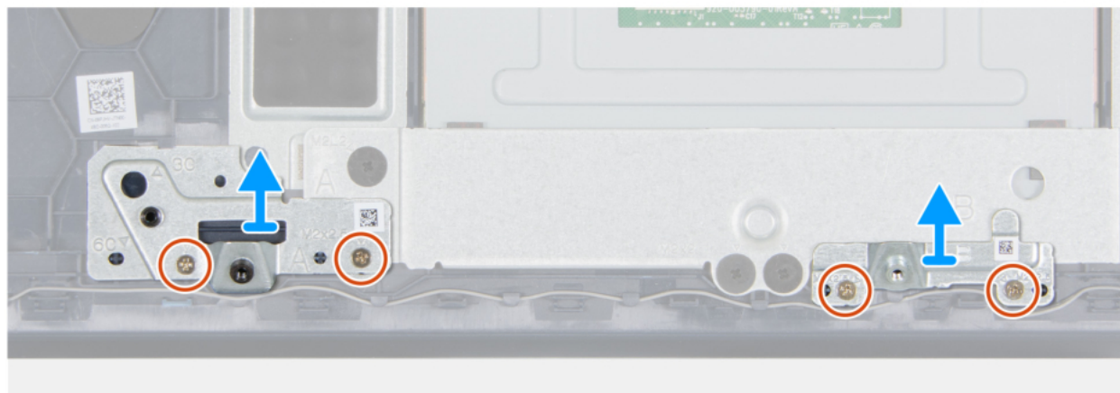
Rysunek 46. Wymontowywanie klamer baterii 6-ogniowej
