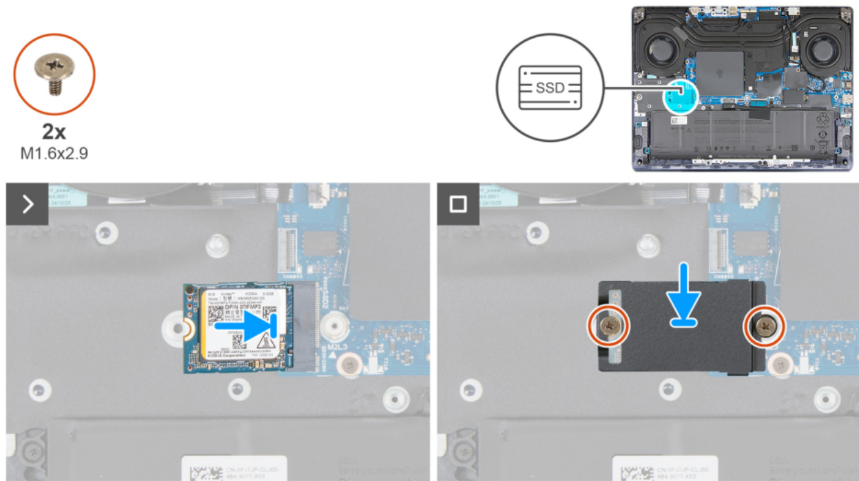
Rysunek 32. Wymontowywanie dysku SSD M.2 2230 z gniazda SSD2
