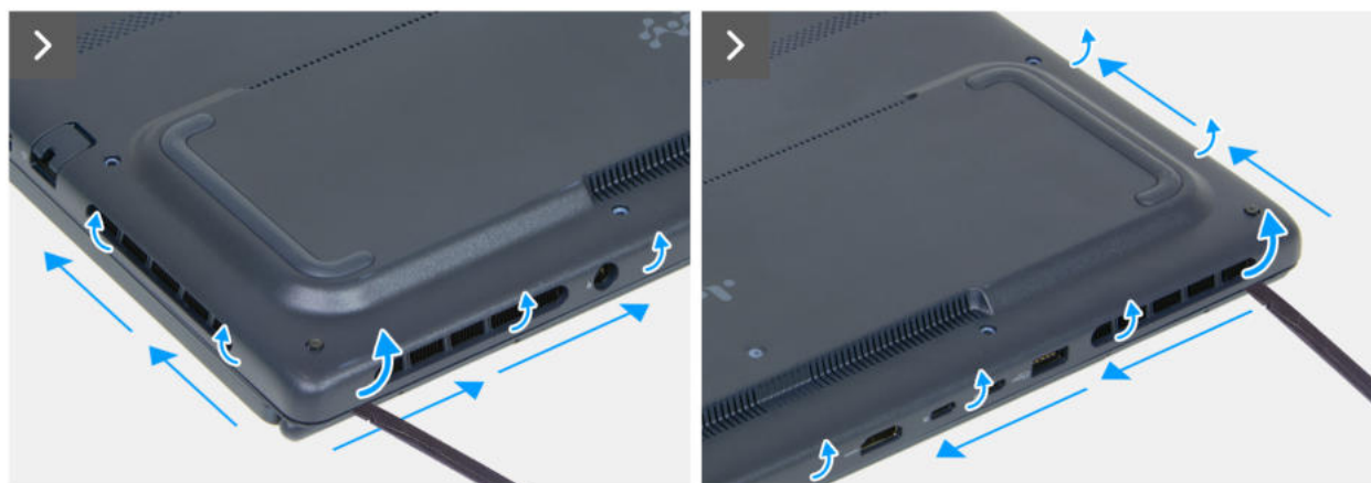
Rysunek 13. Wsuwanie rysika między szczelinę
