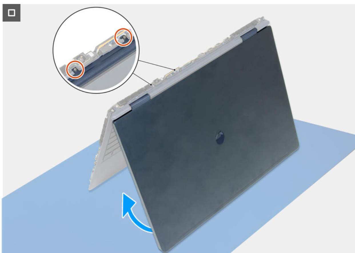
Rysunek 66. Instalacja listwy środkowej
