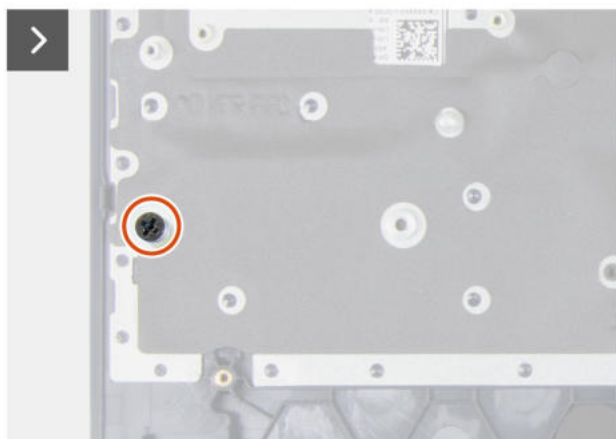
Rysunek 73. Wymontowywanie uchwytych na śruby dysku SSD
