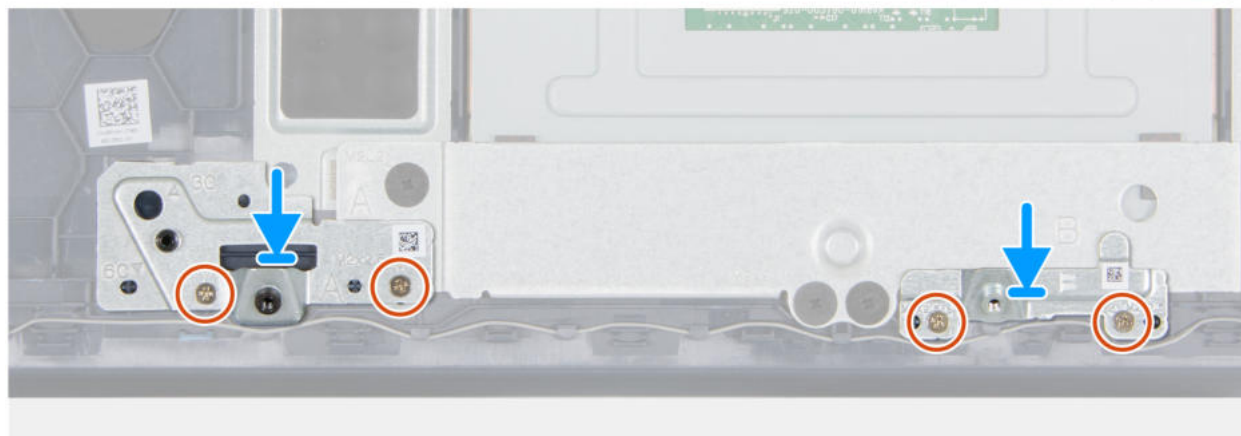
Rysunek 47. Instalacja klamer baterii 6-ogniowej
