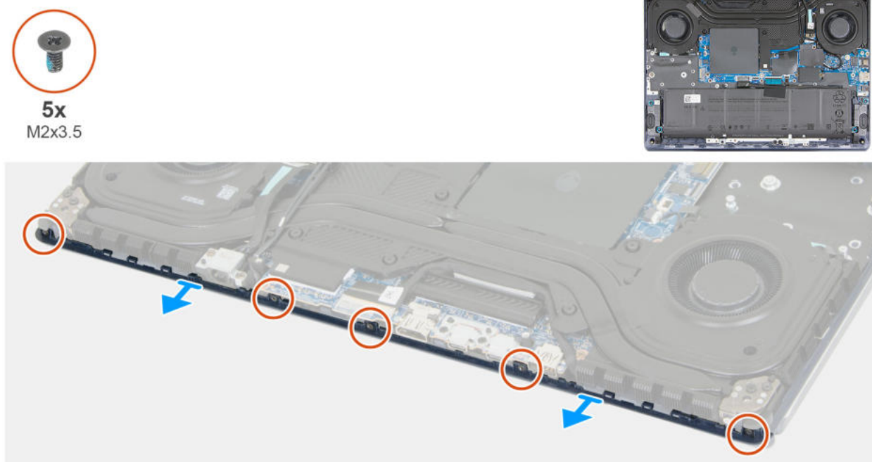
Rysunek 60. Wymontowywanie pokrywy tylnej
