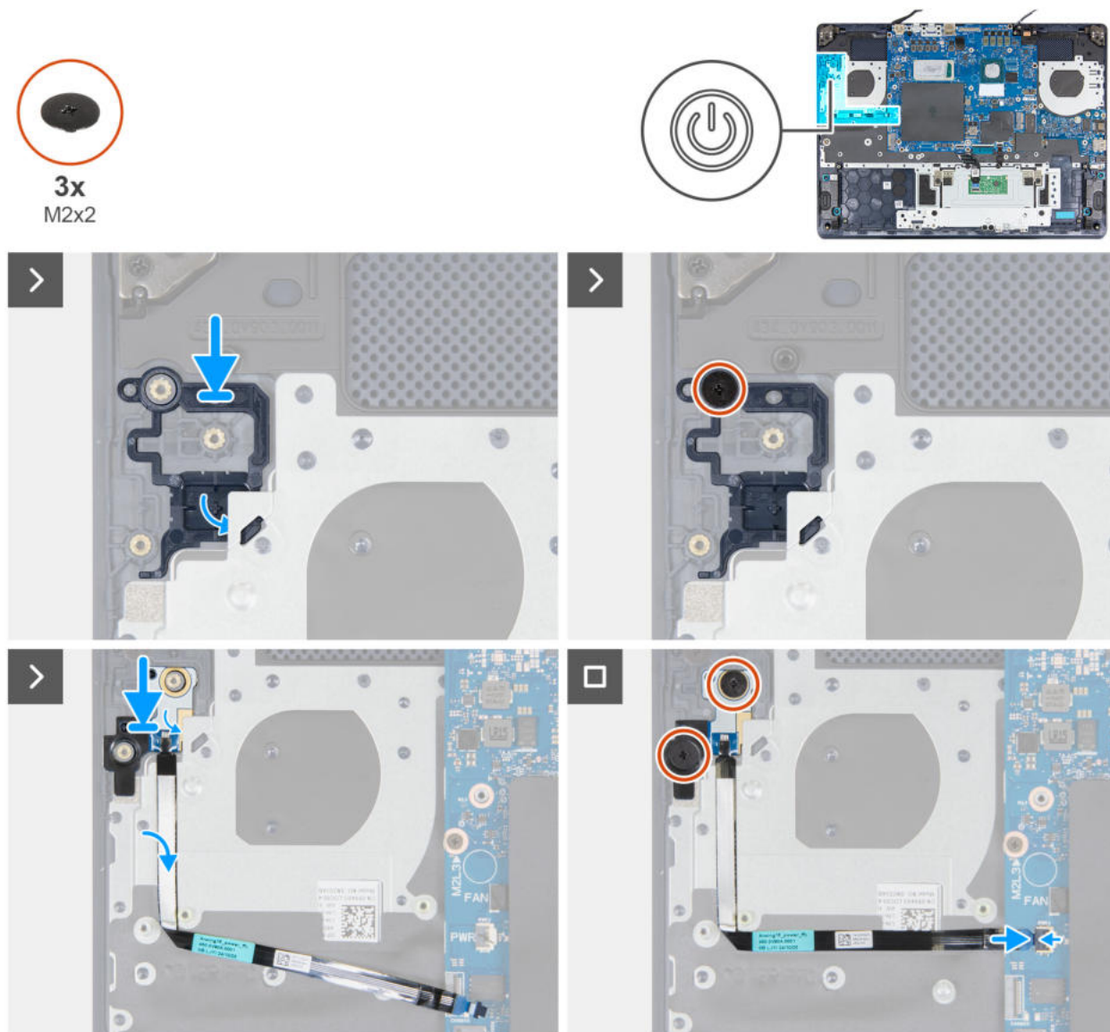
Rysunek 51. Instalacja przycisku zasilania i płyty przycisku zasilania
