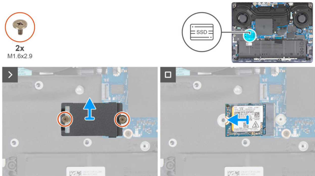
Rysunek 33. Instalacja dysku SSD M.2 2230 w gnieździe SSD2
