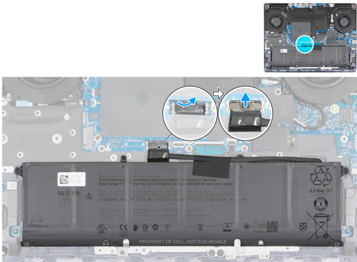
Rysunek 15. Odłączanie kabla baterii
