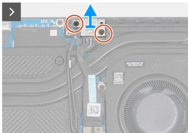
Rysunek 38. Wymontowywanie gniazda zasilacza
