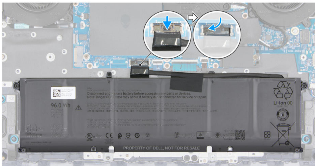
Rysunek 17. Podłączanie kabla baterii
