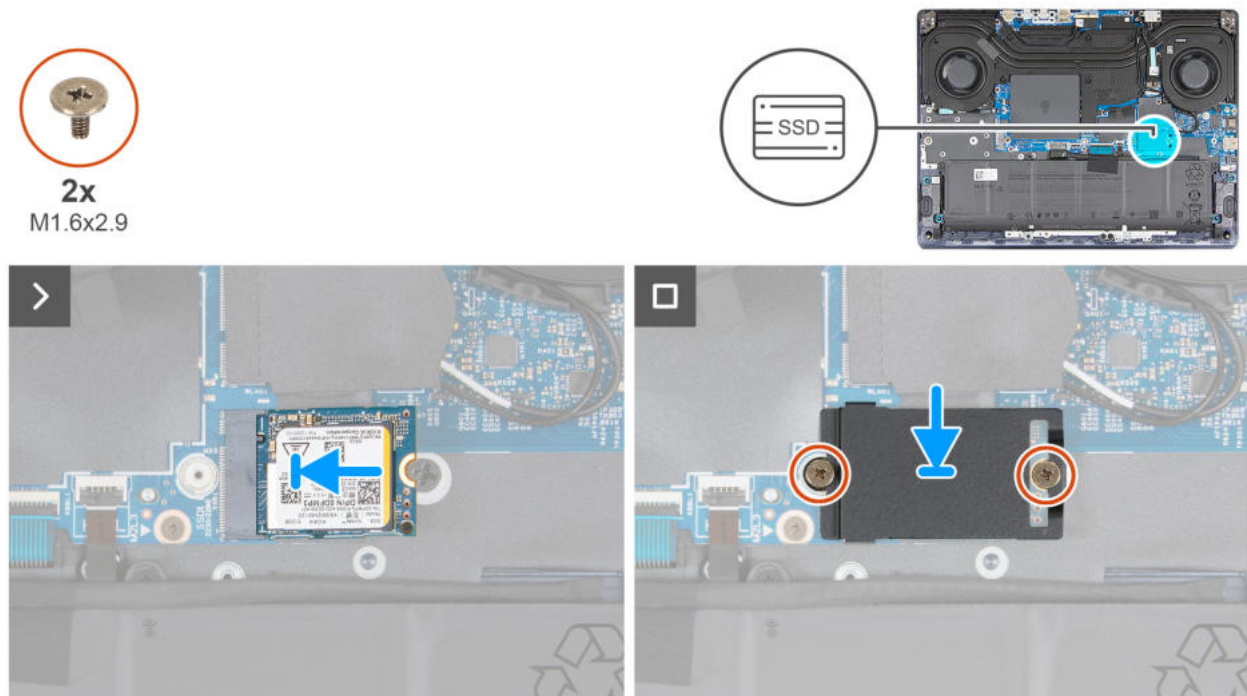
Rysunek 31. Instalacja dysku SSD M.2 2230 w gnieździe SSD1
