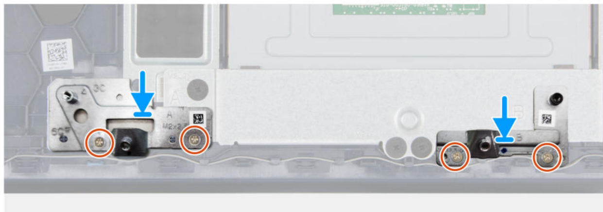
Rysunek 45. Instalacja klamer baterii 3-ogniowej
