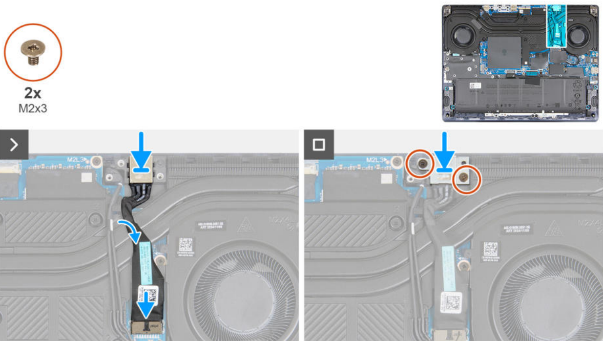
Rysunek 39. Instalowanie gniazda zasilacza
