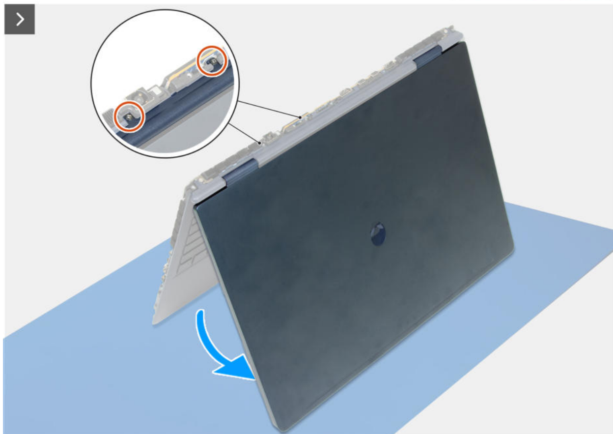
Rysunek 63. Wymontowywanie listwy środkowej
