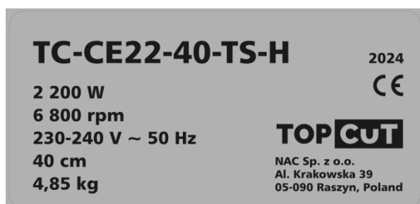
Tabliczka znamionowa
