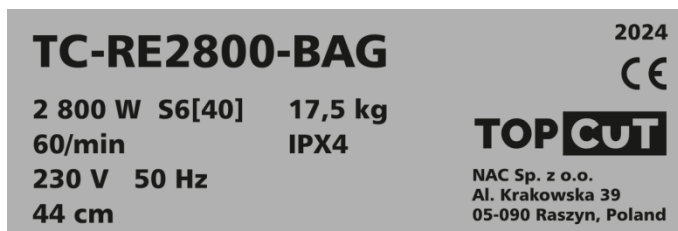
Tabliczka znamionowa
