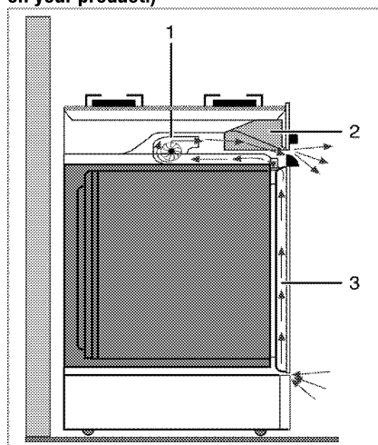
1 Cooling fan
