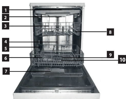
Přední pohled
