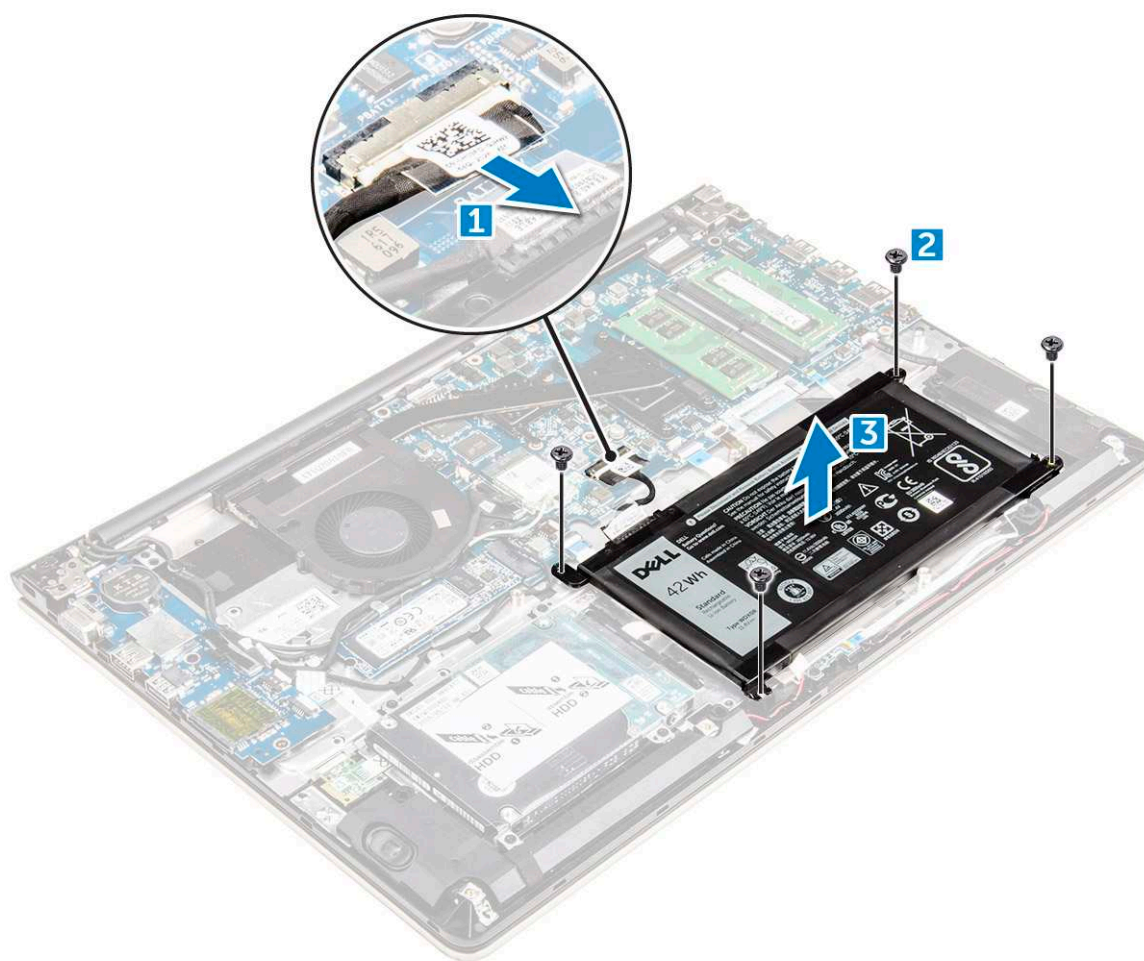
Rysunek 7. Wymontowywanie akumulatora
