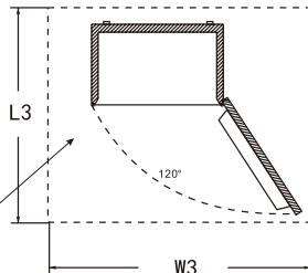
Całkowita przestrzeń potrzebna do eksploatacji produktu
