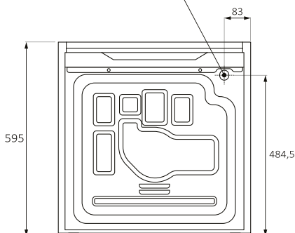
Widok tylny
