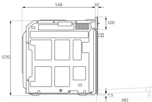
Widok boczny
