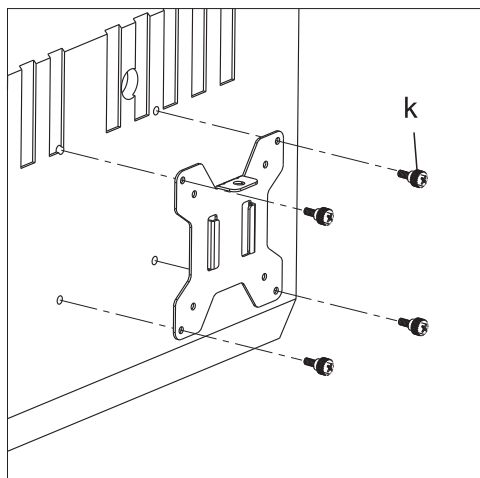
Dla monitora z płaską tylną obudową
