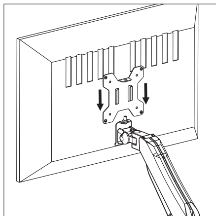
Nasun płytkę z przytwierdzonym monitorem na prowadnice w głowicy uchwytu.
