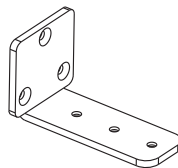
(c) Stopka do klamry typu „C”
