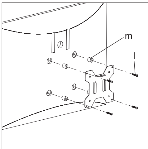
Dla monitora z zakrzywionym lub cofniętym tyłem
