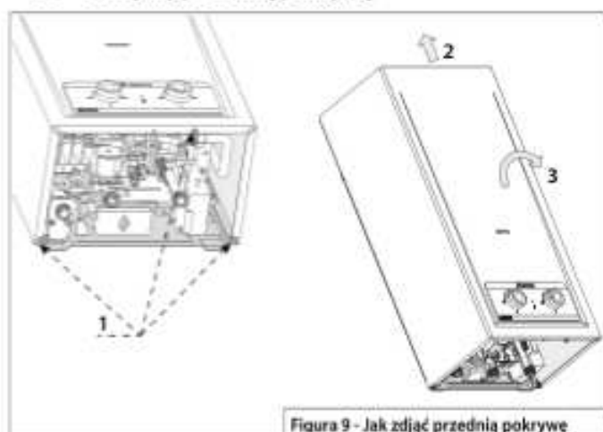
Figura 9 - Jak zdjąć przednią pokrywę
