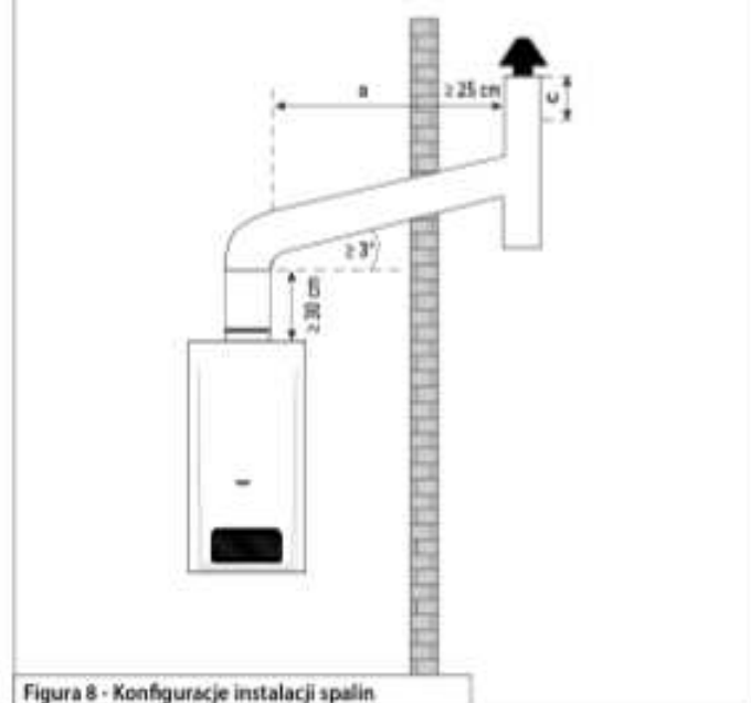
Figura 8 - Konfiguracje instalacji spalin
