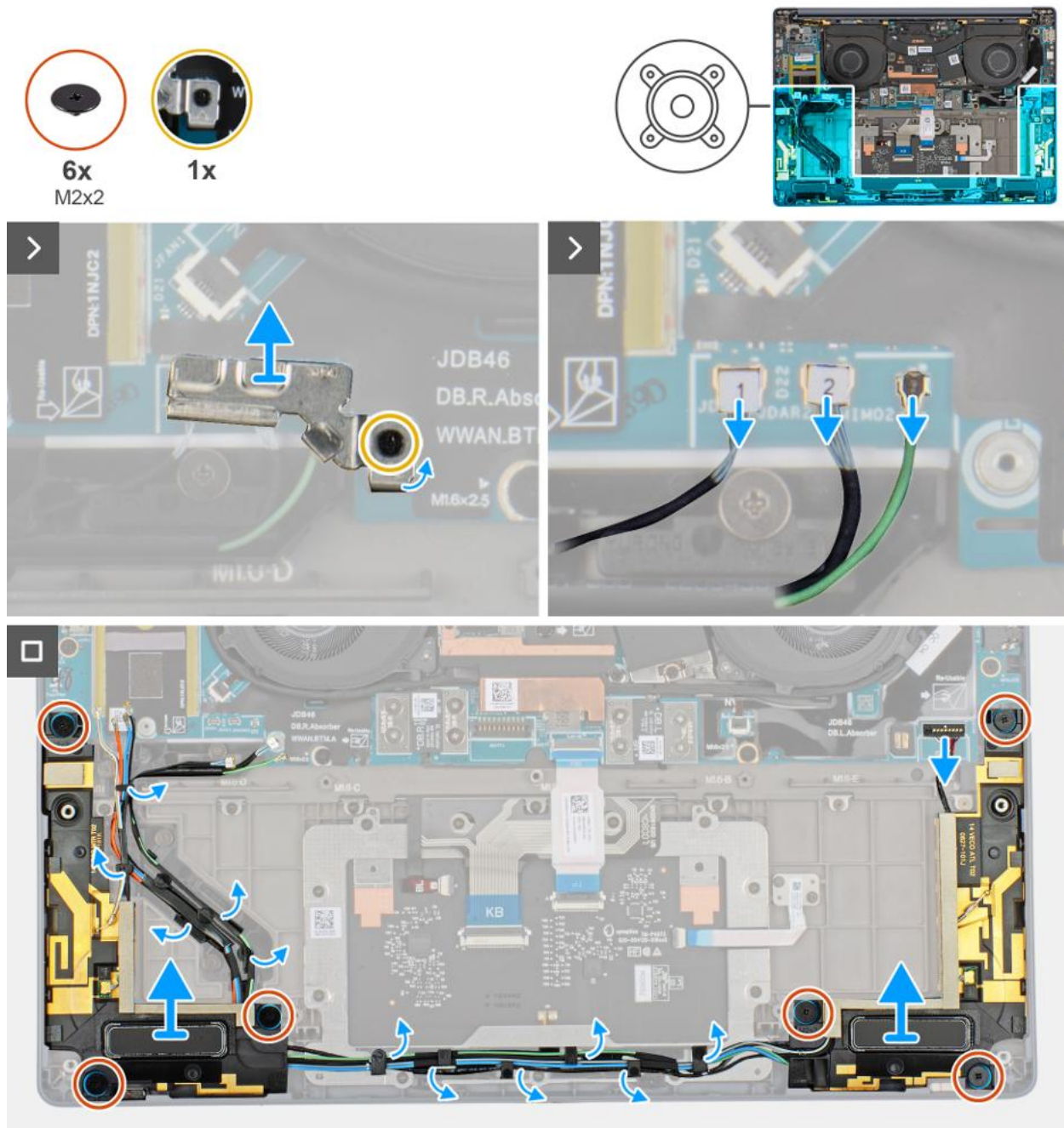
Rysunek 36. Wymywanie głośników z antenami (konfiguracja WWAN)
