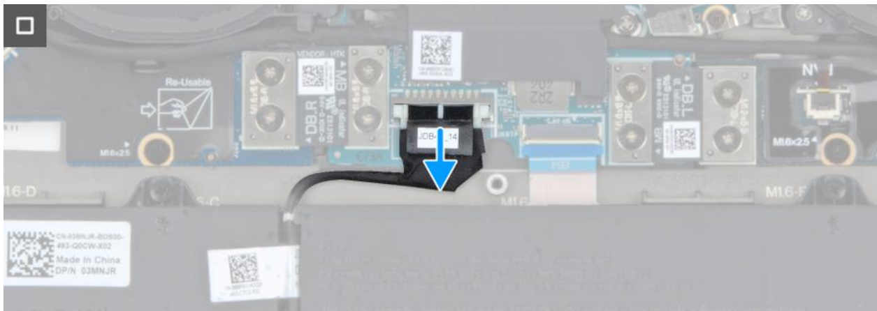
Rysunek 18. Odłączenie kabla baterii od płyty głównej
