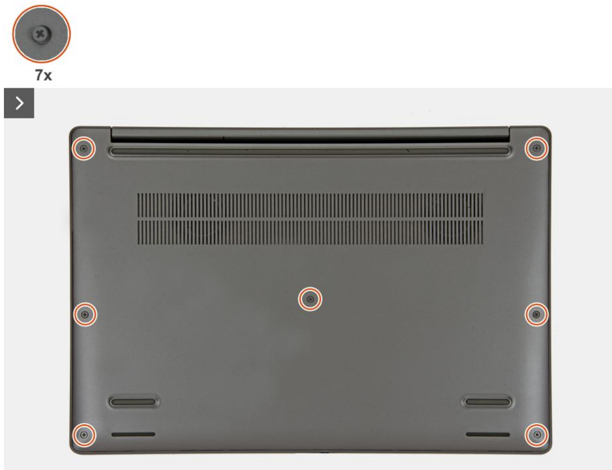
Rysunek 16. Luzowanie śrub mocujących
