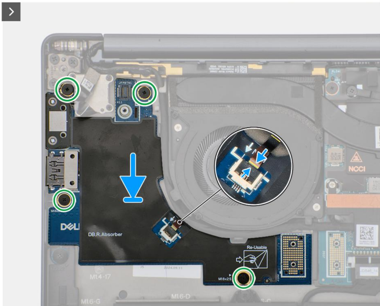
Rysunek 48. Instalowanie prawej płyty we/wy (bez anten WWAN)
