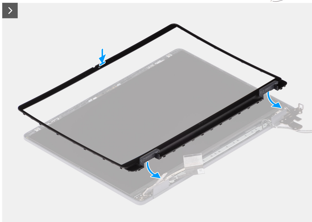
Rysunek 72. Instalowanie ramki wyświetlacza
