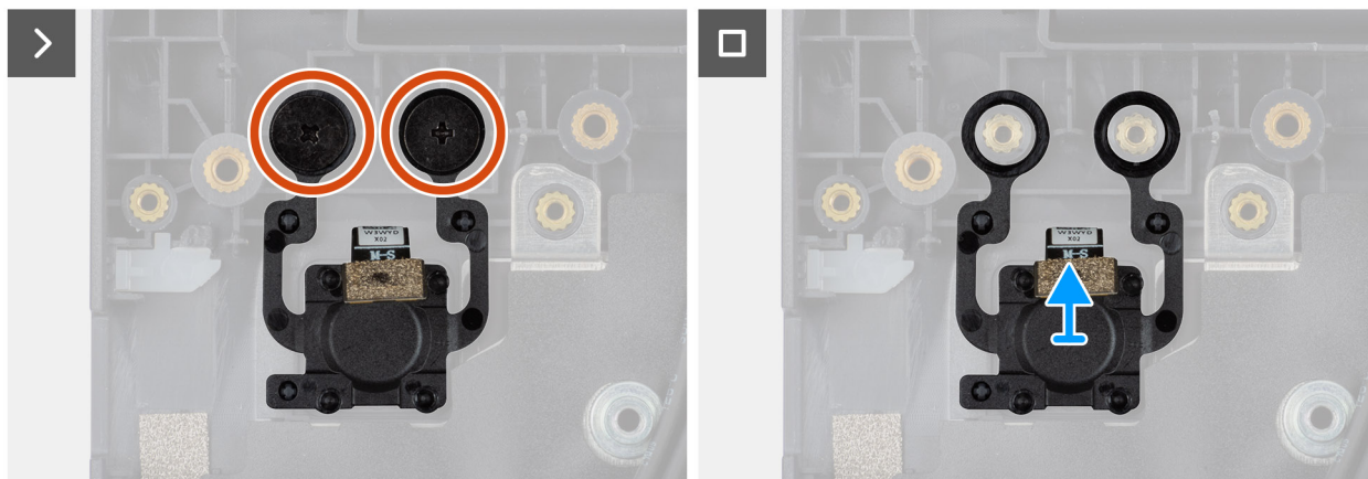
Rysunek 40. Wymontowywanie przycisku zasilania z czytnikiem linii papilarnych
