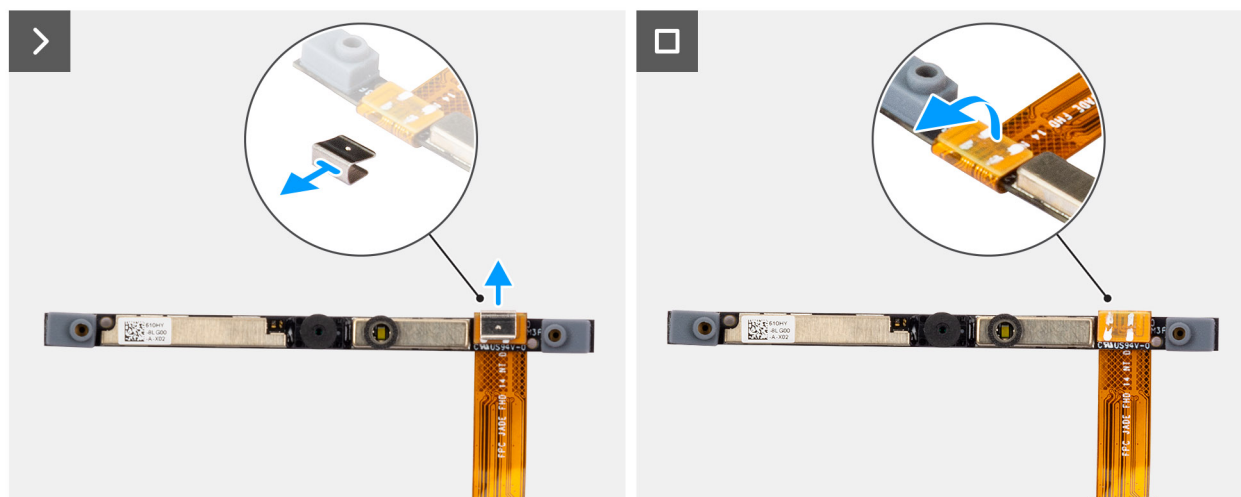
Rysunek 82. Wymontowywanie kamery
