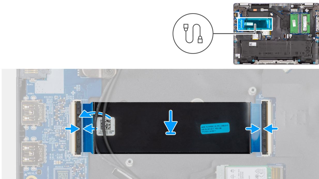
Rysunek 39. Instalowanie płyty we/wy
