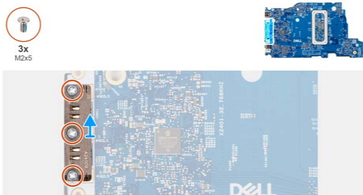
Rysunek 48. Wymontowywanie modułu USB-C
