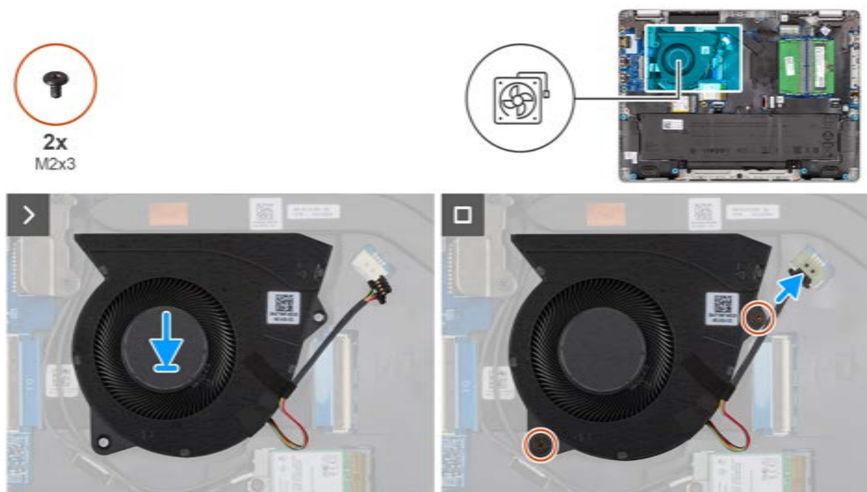
Rysunek 31. Instalowanie wentylatora
