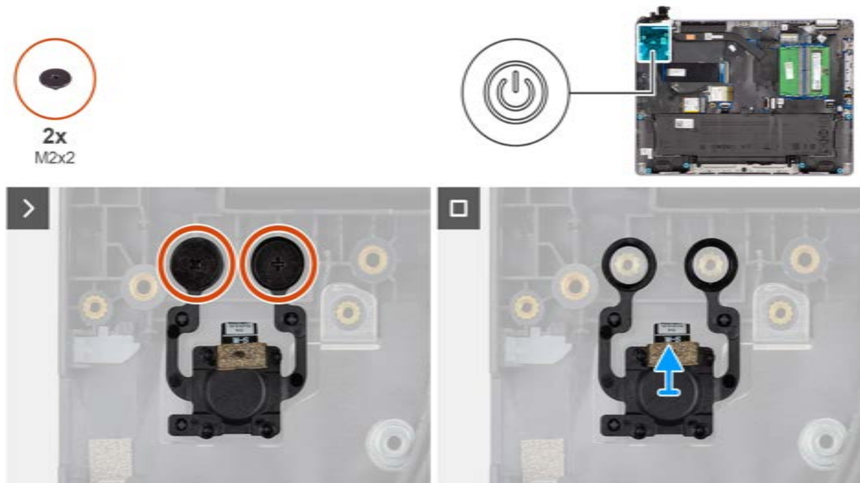
Rysunek 40. Wymontowywanie przycisku zasilania z czytnikiem linii papilarnych
