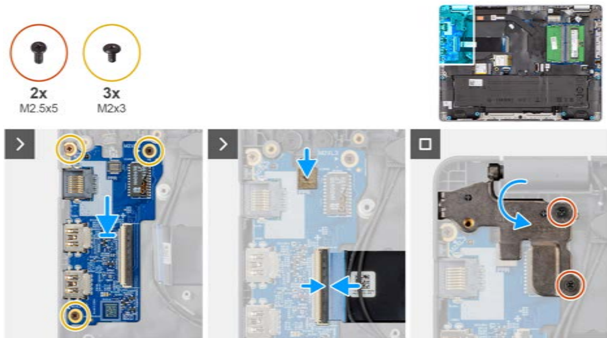
Rysunek 37. Instalowanie płyty we/wy
