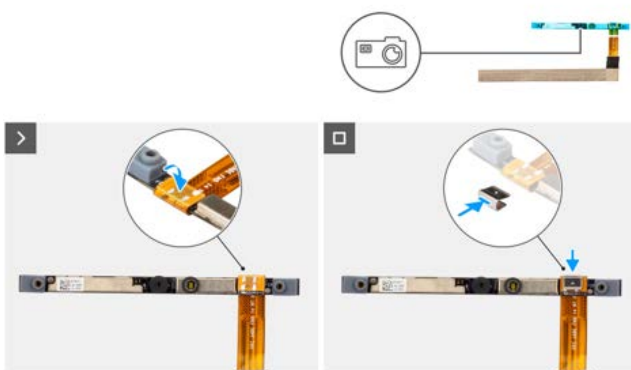
Rysunek 83. Instalowanie kamery
