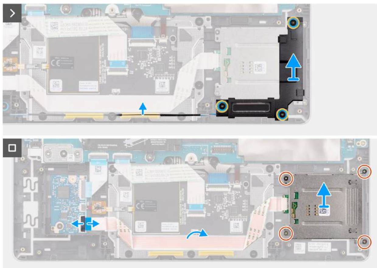
Rysunek 44. Wymontowywanie czytnika kart smart
