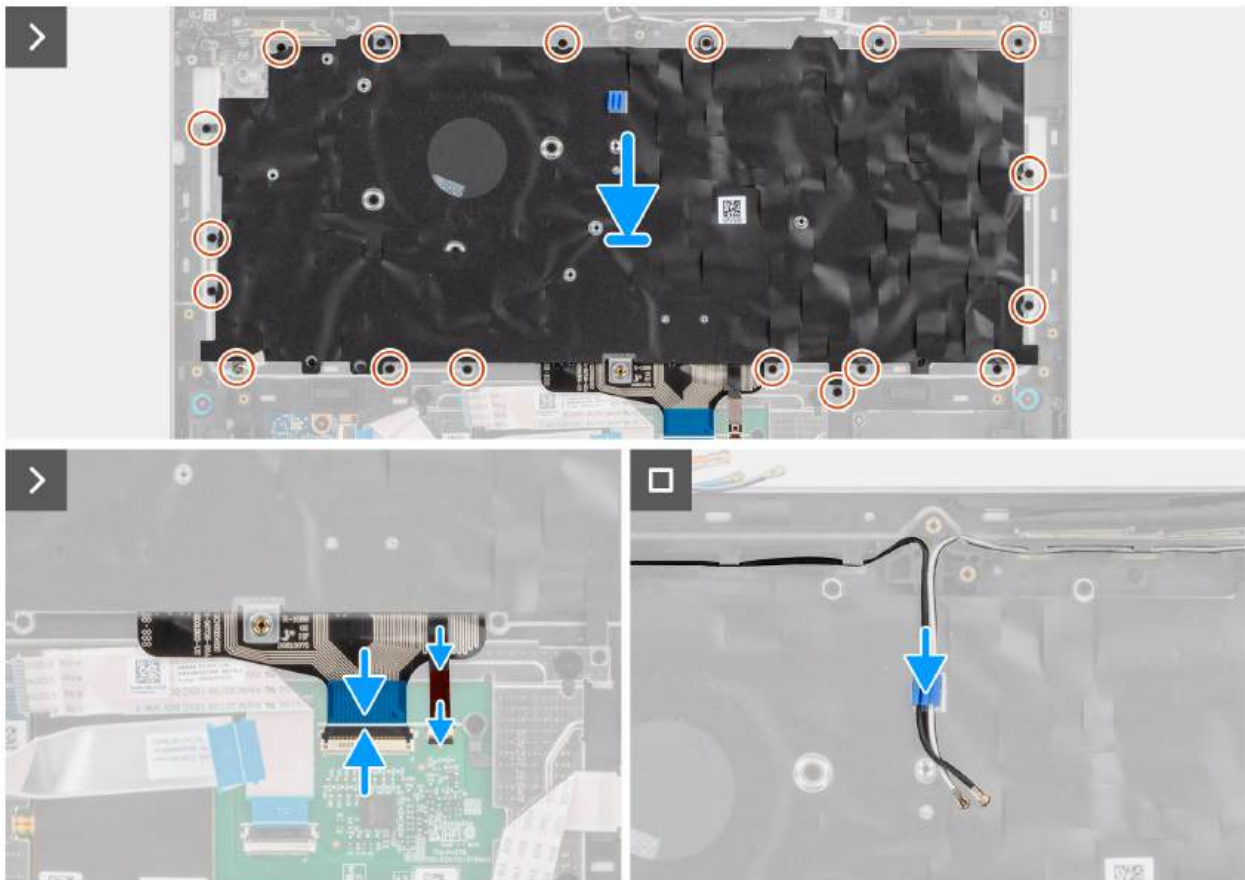
Rysunek 100. Instalowanie klawiatury
