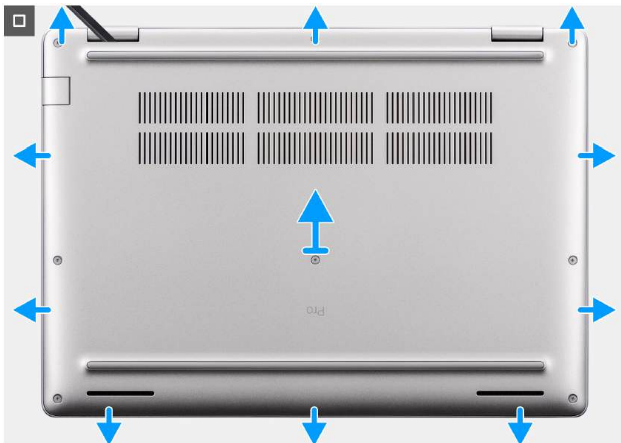
Rysunek 18. Wymontowywanie pokrywy dolnej
