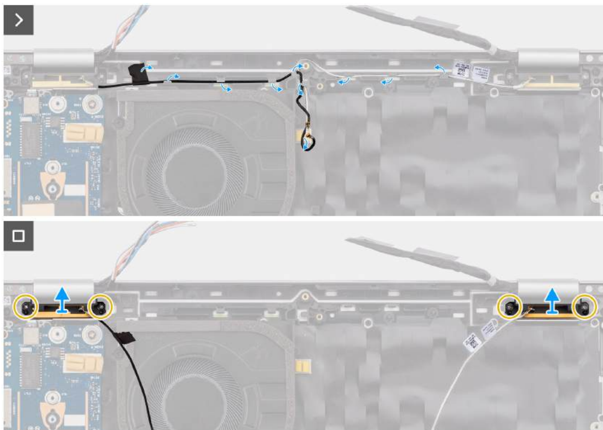
Rysunek 52. Wymontowywanie modułów anten sieci WLAN
