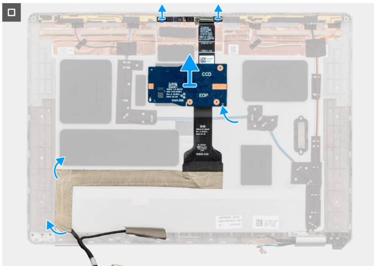
Rysunek 86. Odłączenie wyświetlacza kamery RGB/IR
