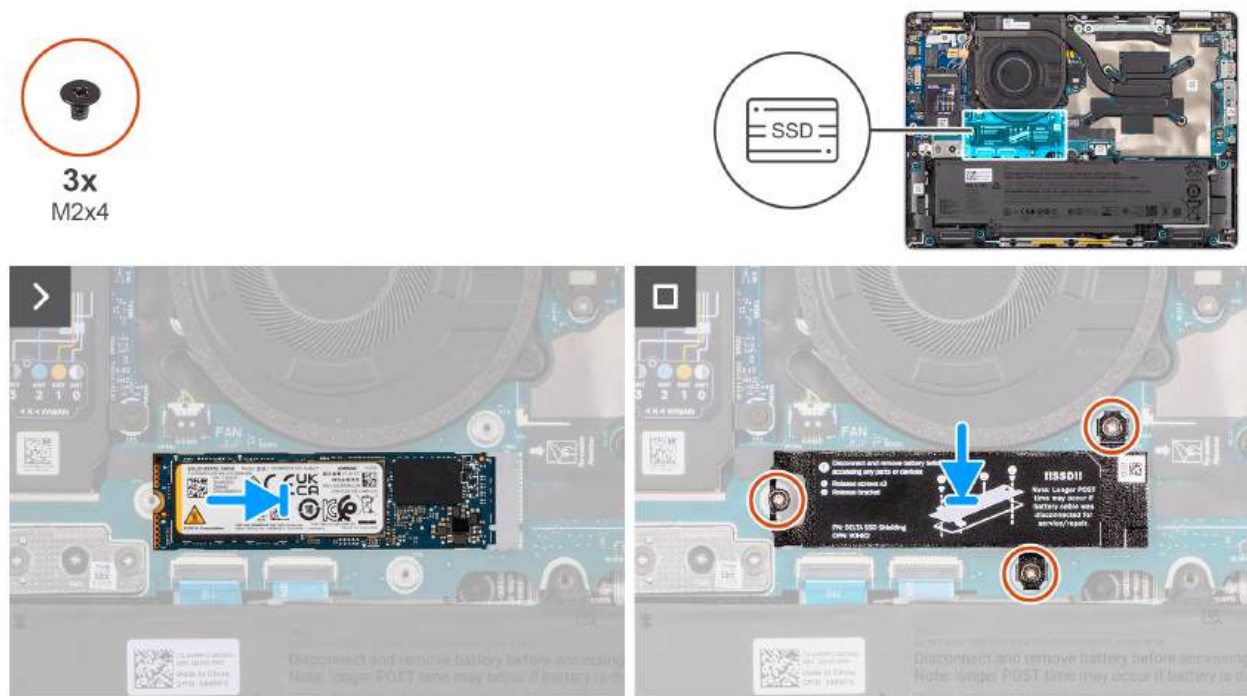
Rysunek 34. Instalowanie dysku SSD M.2 2280
