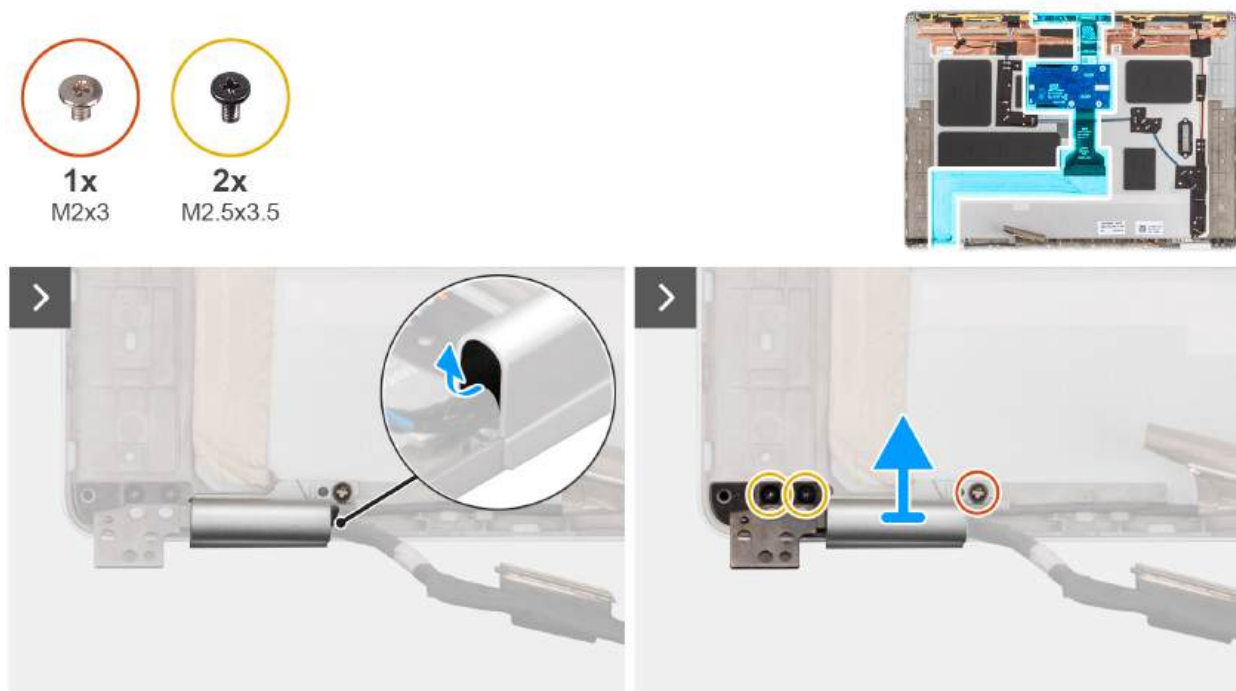
Rysunek 85. Odłączanie wyświetlacza kamery RGB/IR
