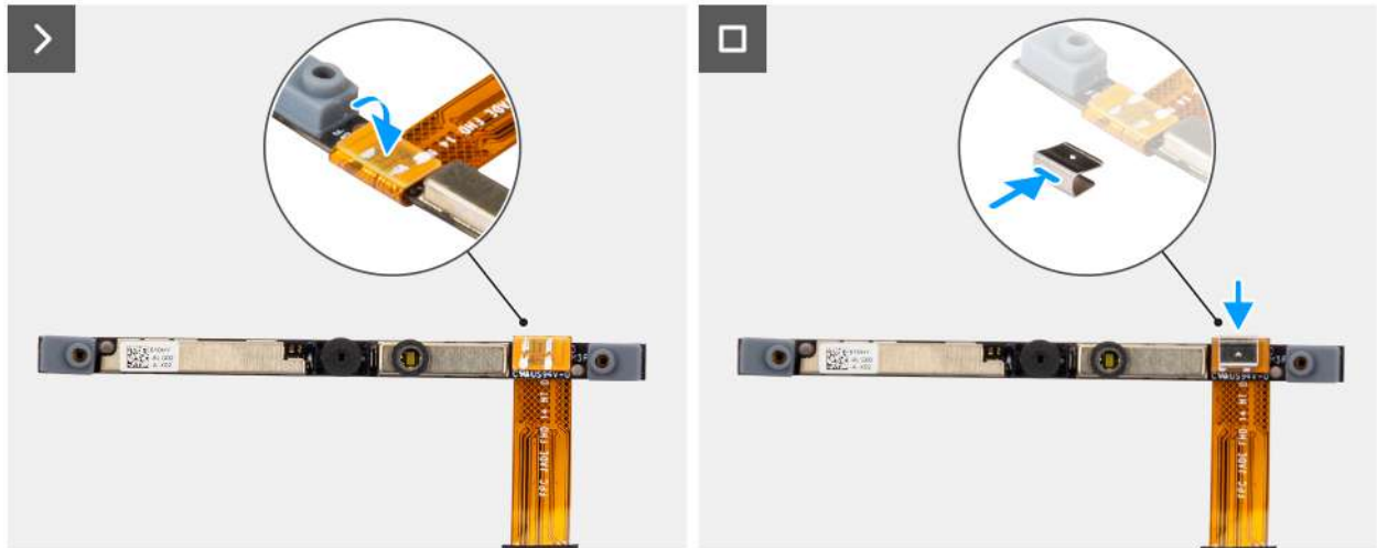
Rysunek 120. Instalowanie kamery
