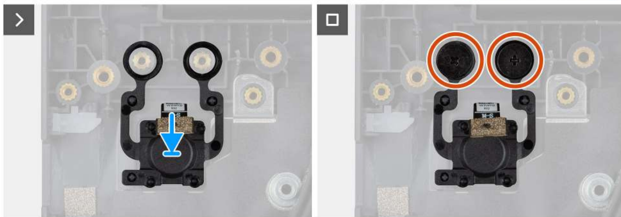
Rysunek 56. Instalowanie przycisku zasilania z czytnikiem linii papilarnych
