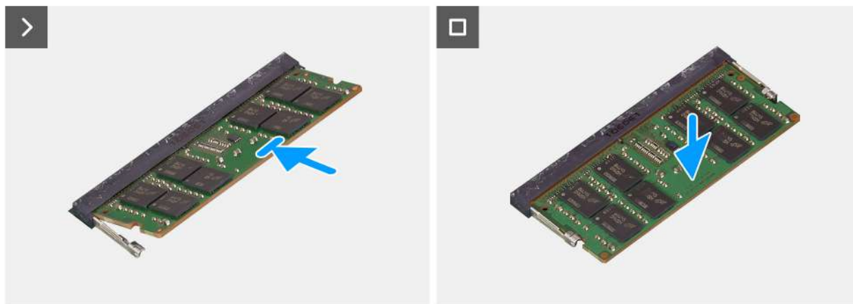
Rysunek 22. Instalowanie modułów pamięci
