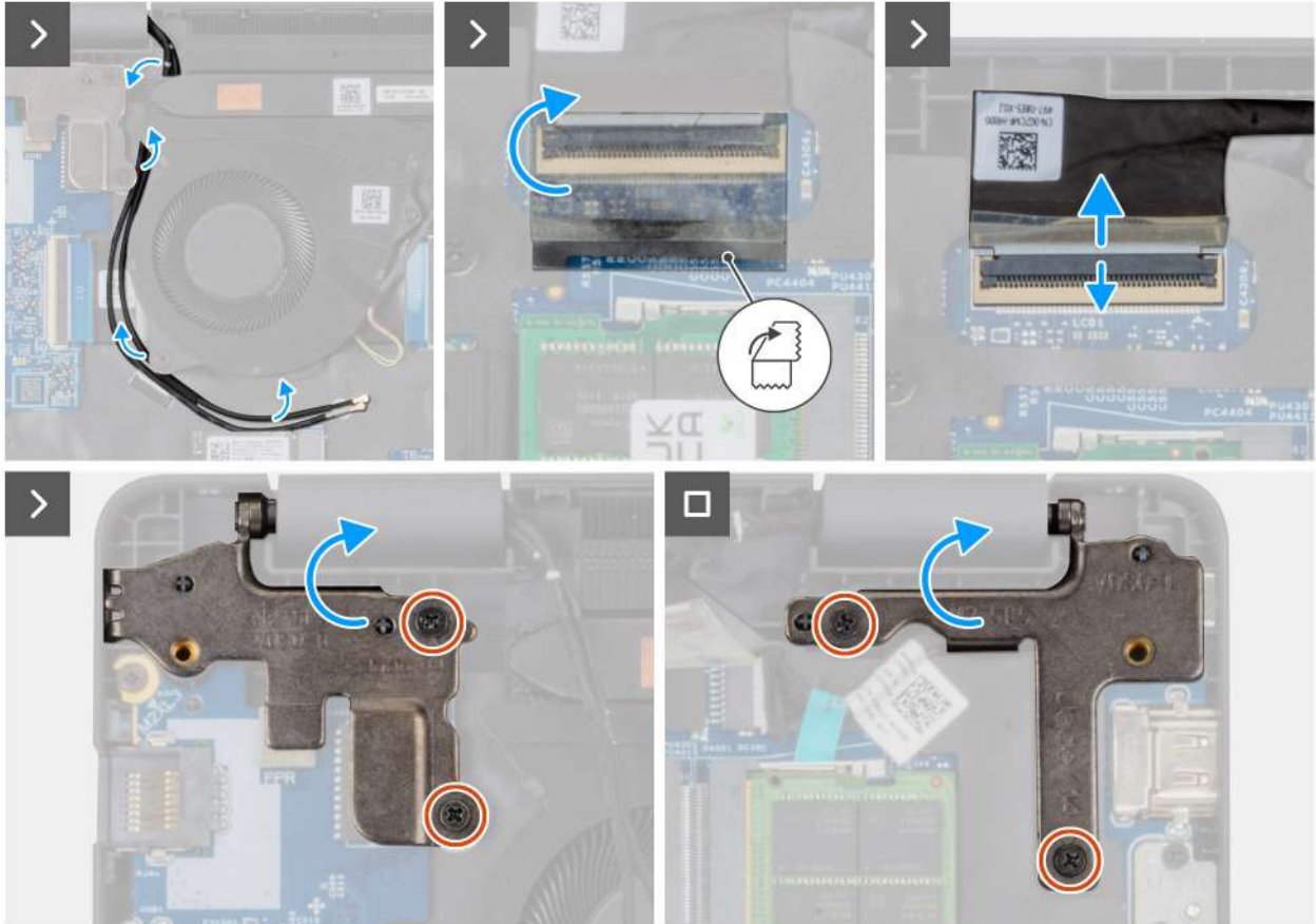
Rysunek 99. Wymontowywanie zestawu wyświetlacza
