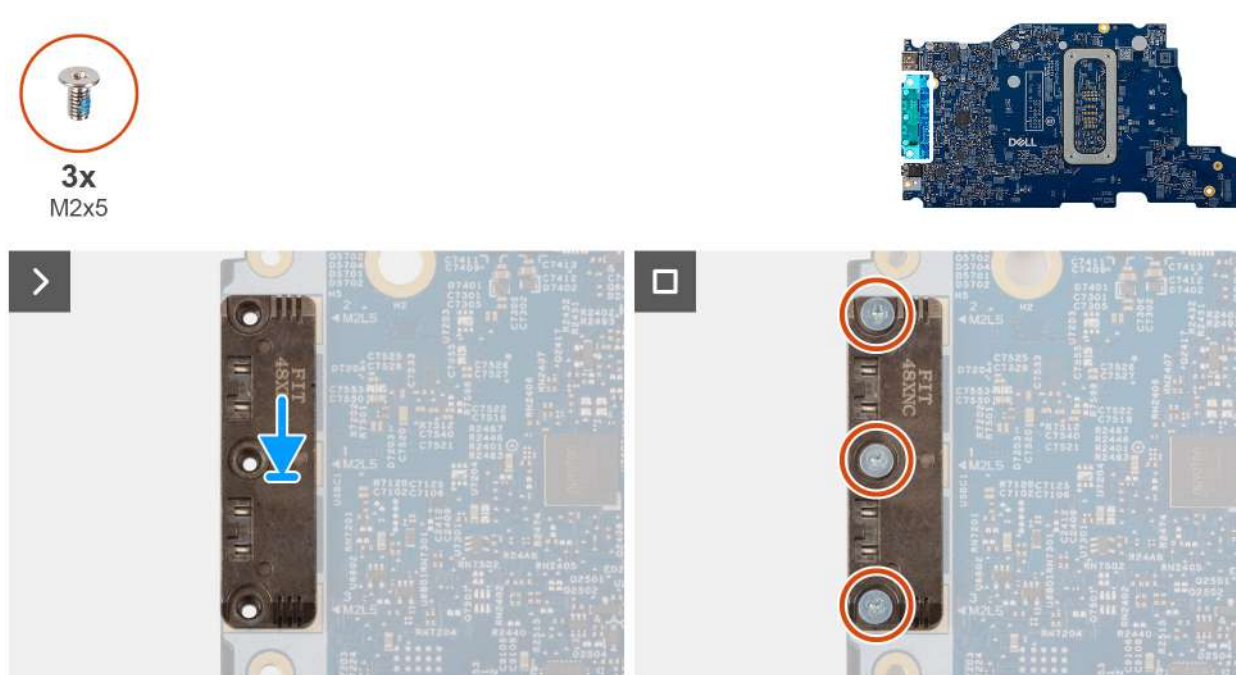
Rysunek 76. Instalowanie modułu USB Type-C
