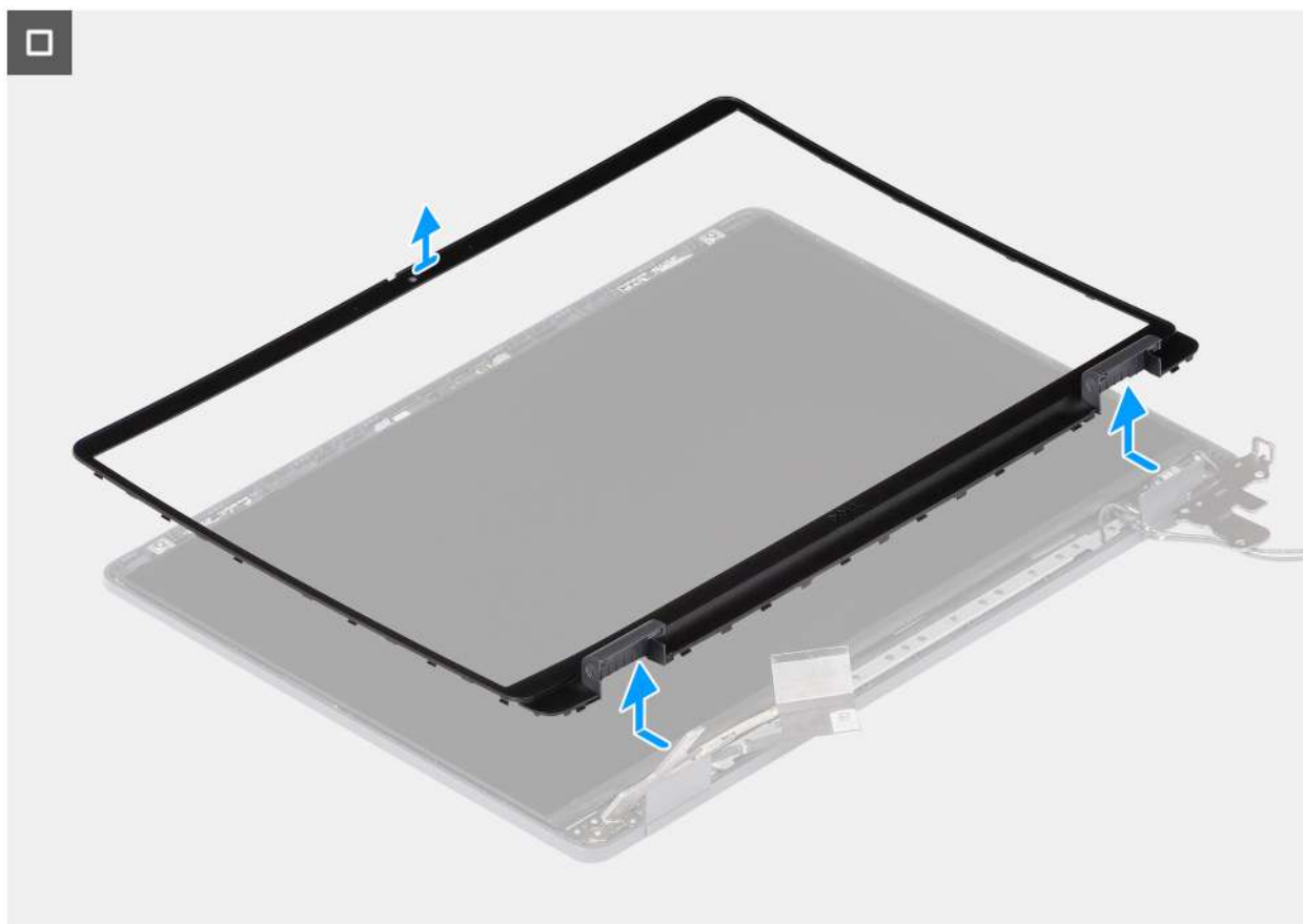
Rysunek 108. Wymontowywanie ramki wyświetlacza
