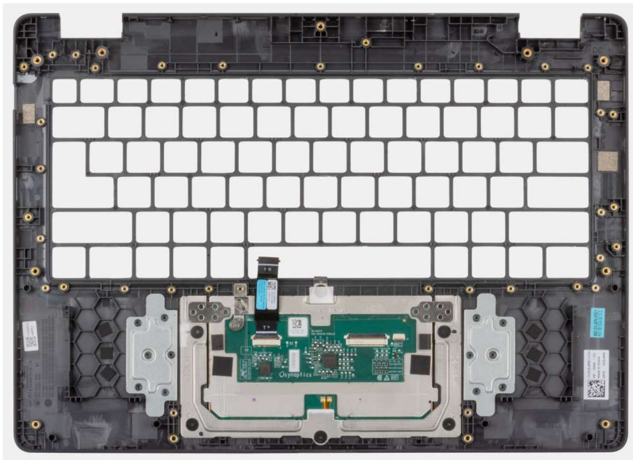
Rysunek 95. Wymontowywanie podpórki na nadgarstek i zestawu
