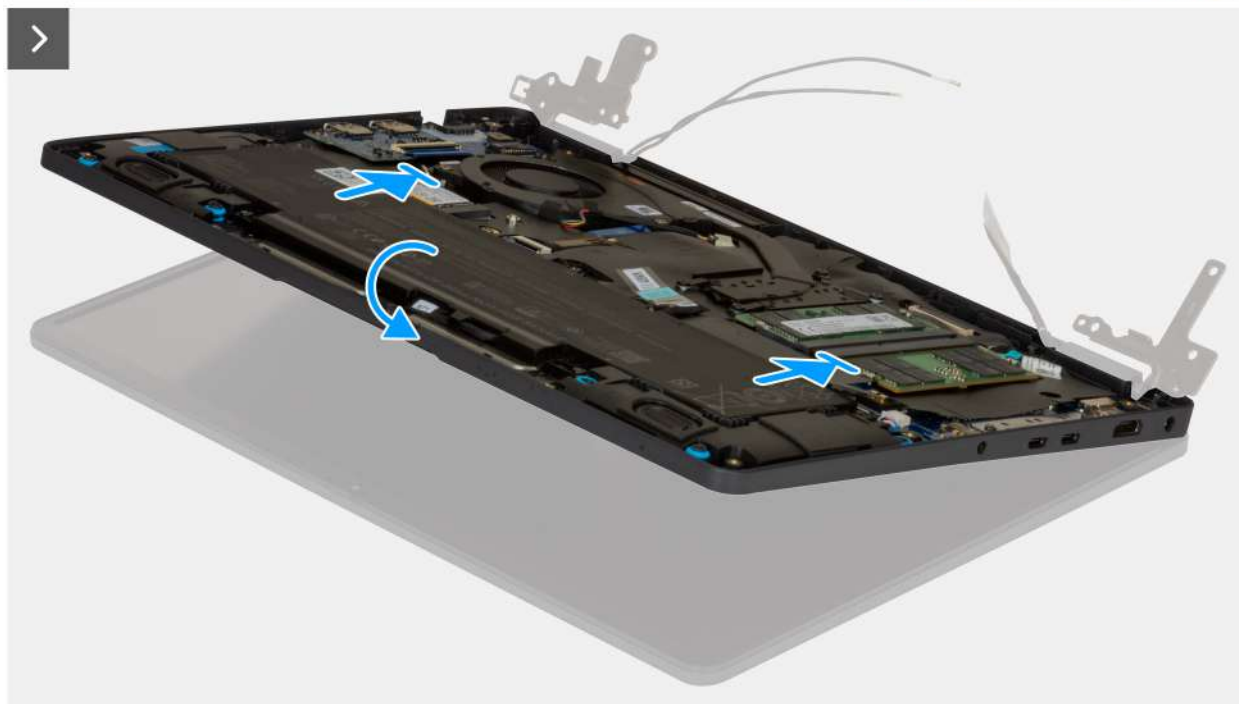
Rysunek 102. Instalowanie zestawu wyświetlacza
