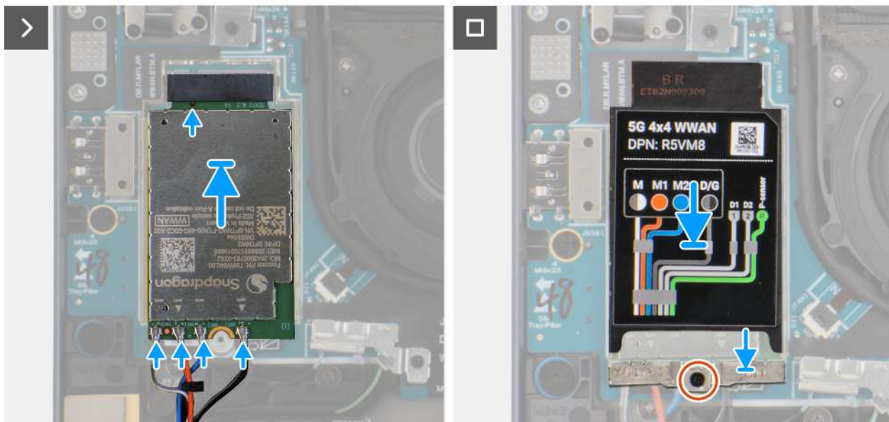
Rysunek 29. Instalowanie karty sieci WWAN
