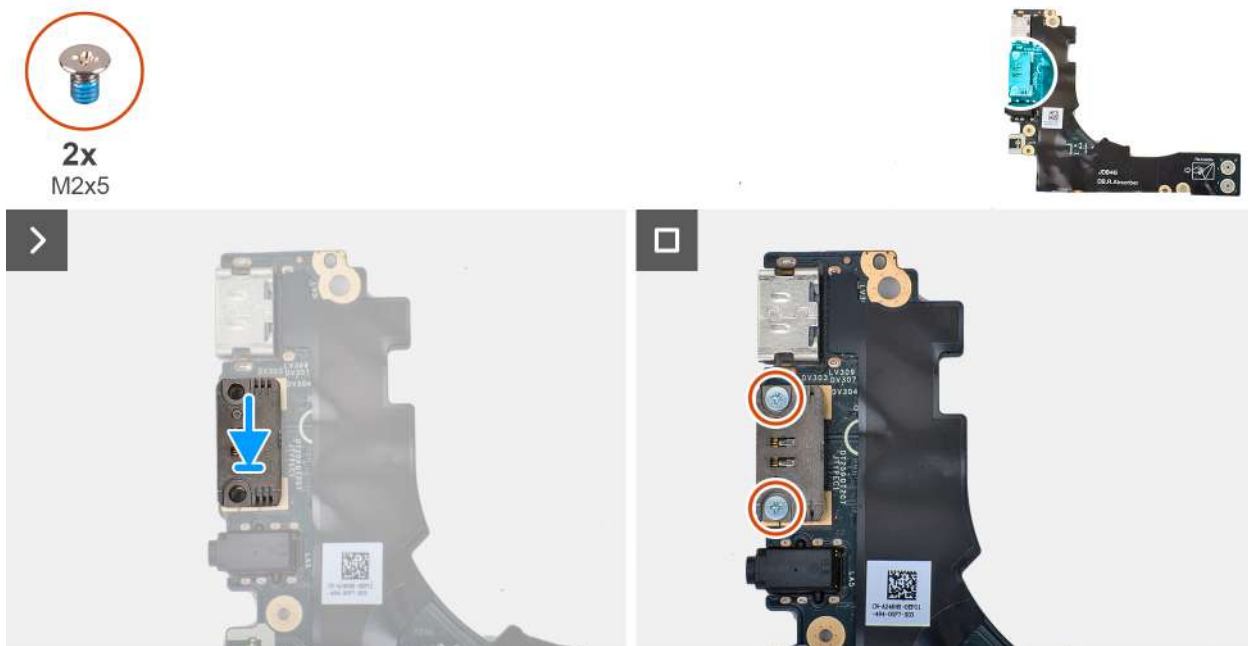
Rysunek 58. Wymowanie prawego modułu USB typu C
