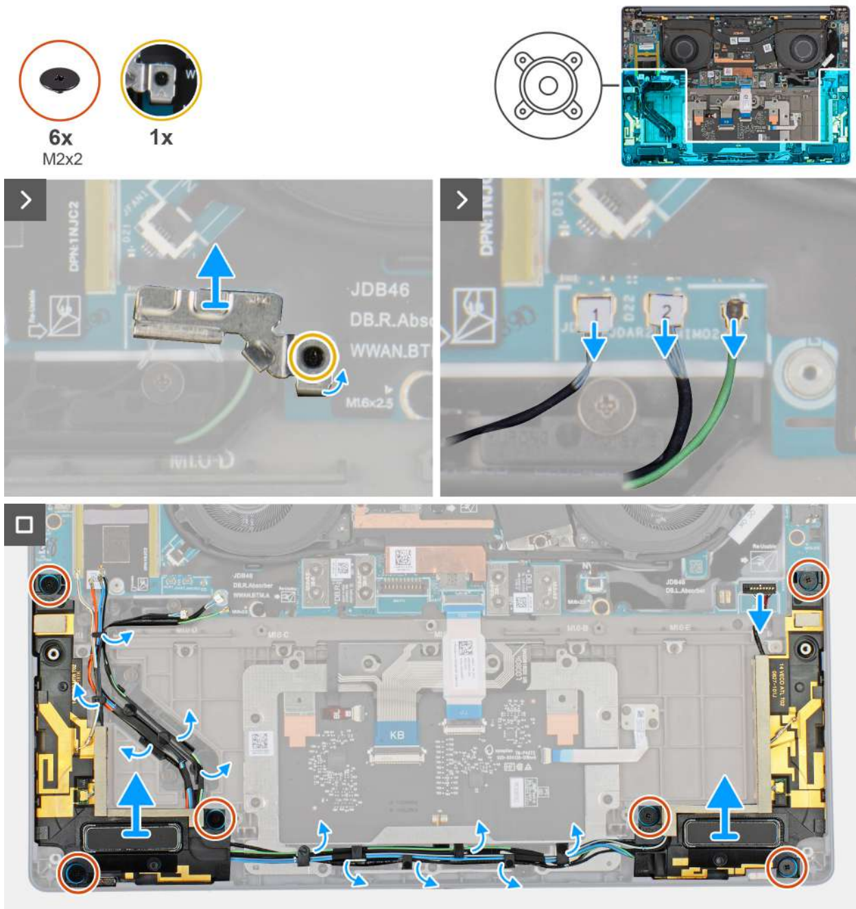
Rysunek 36. Wymontowanie głośników z antenami (konfiguracja WWAN)
