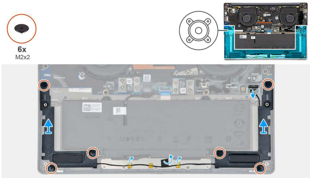
Rysunek 34. Wymontowanie głośników bez anteny (konfiguracja WLAN)
