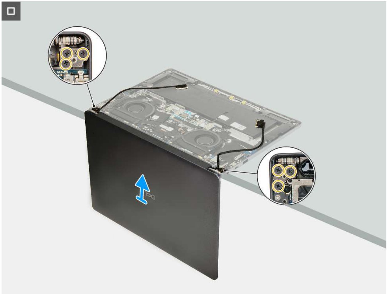
Rysunek 63. Wymontowywanie zestawu wyświetlacza
