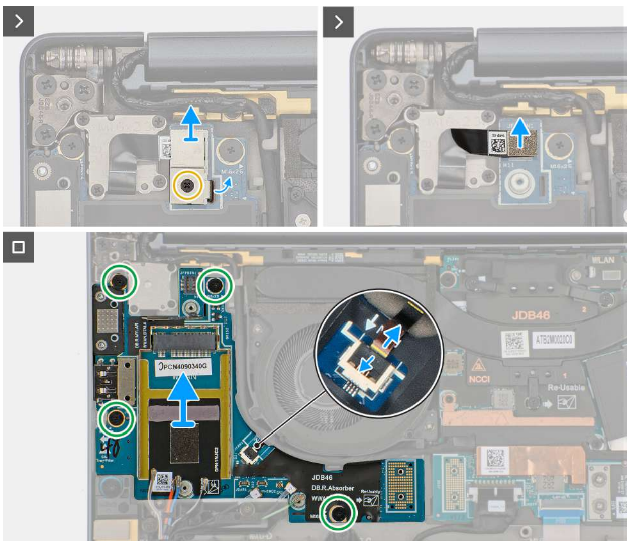
Rysunek 51. Wymowanie prawej płyty we/wy (z WWAN)
