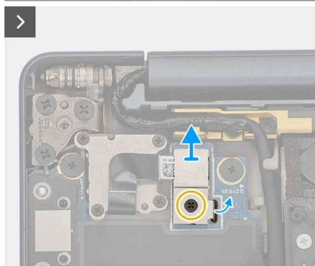
Rysunek 44. Wykręcanie śrub
