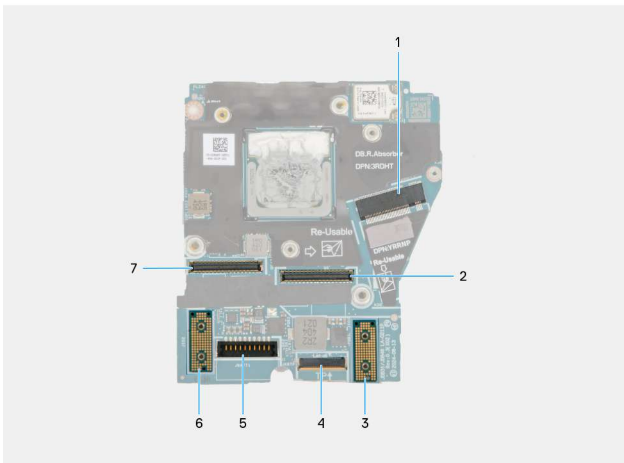
Rysunek 67. Elementy płyty głównej
