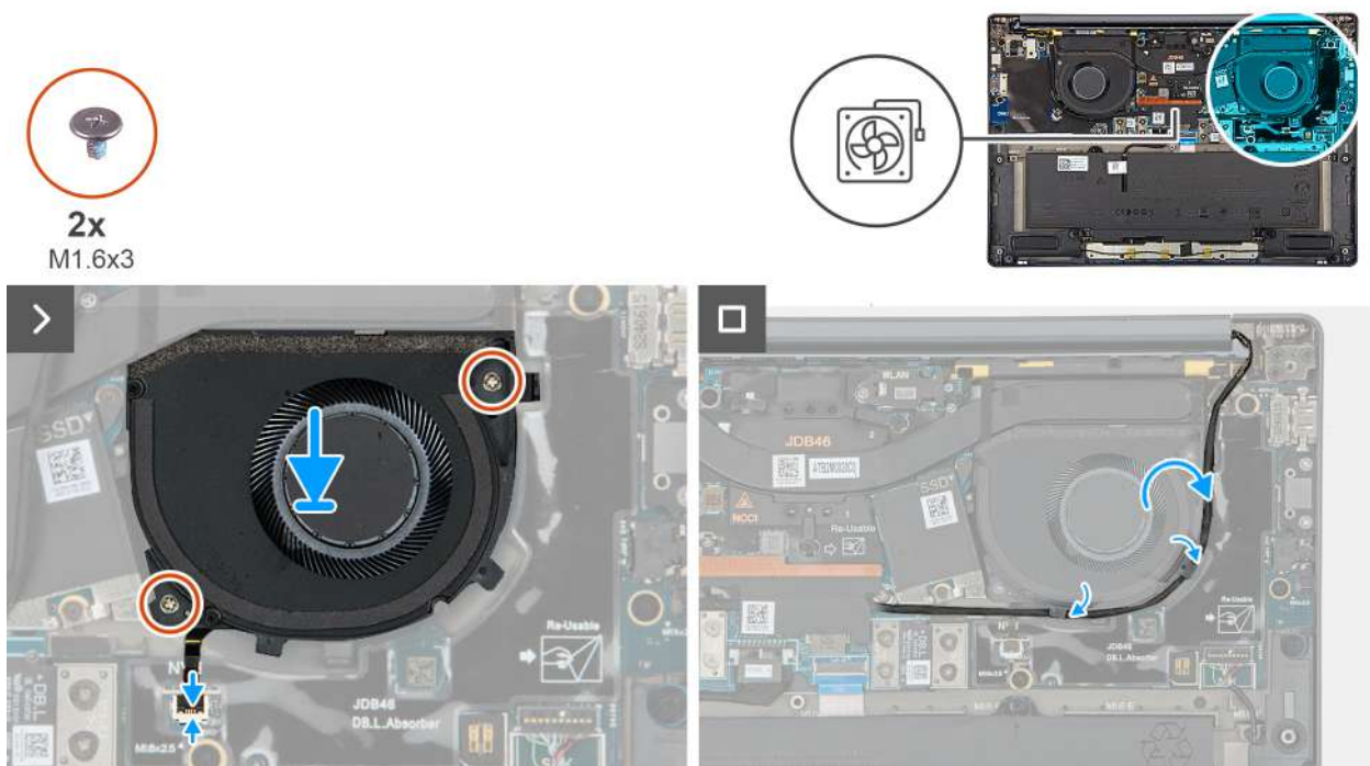
Rysunek 31. Instalowanie lewego wentylatora
