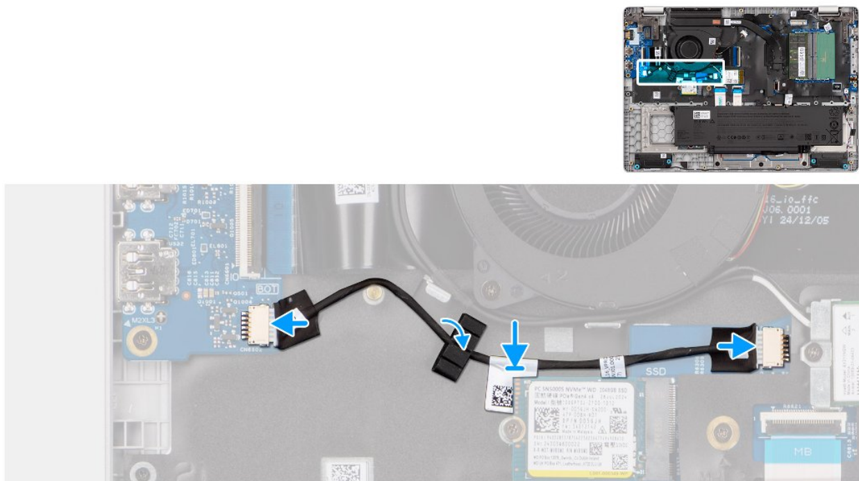
Rysunek 48. Instalowanie vPro
