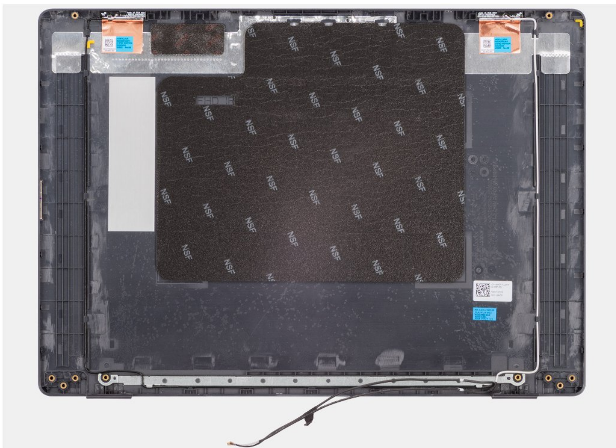
Rysunek 118. Instalowanie zestawu pokrywy tylnej wyświetlacza
