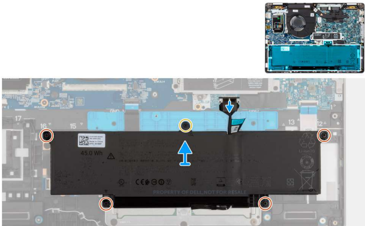
Rysunek 15. Odłączenie kabla baterii
