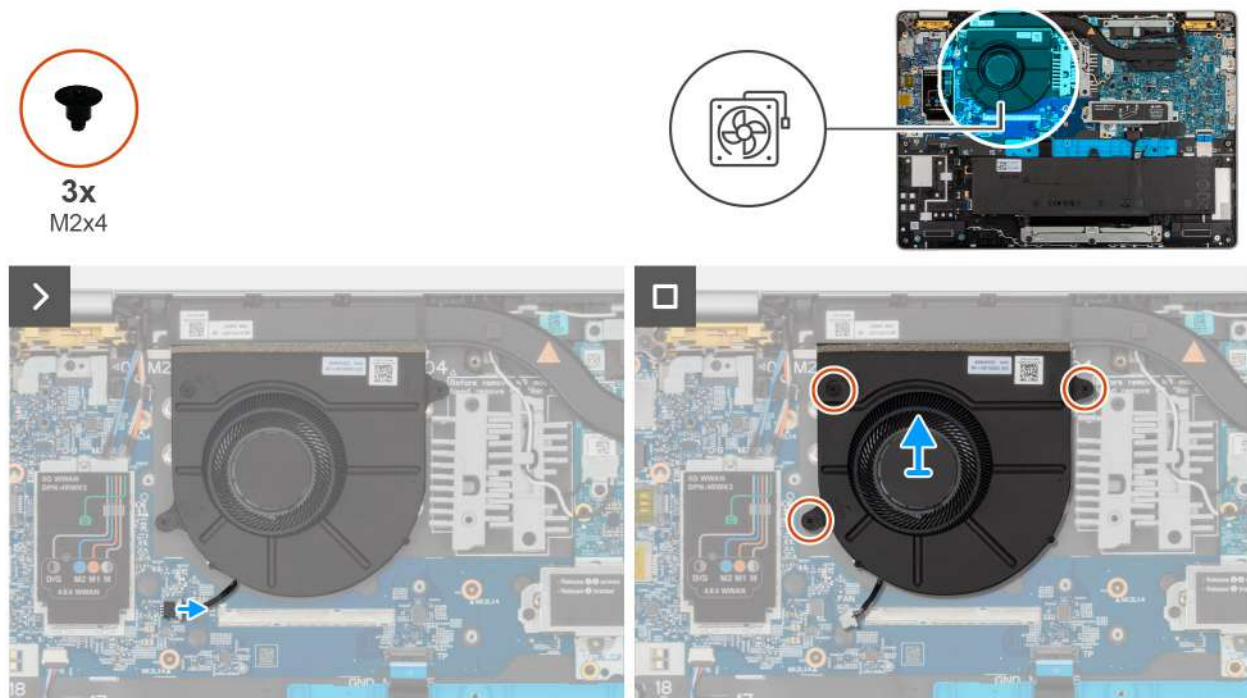
Rysunek 28. Wymontowywanie wentylatora
