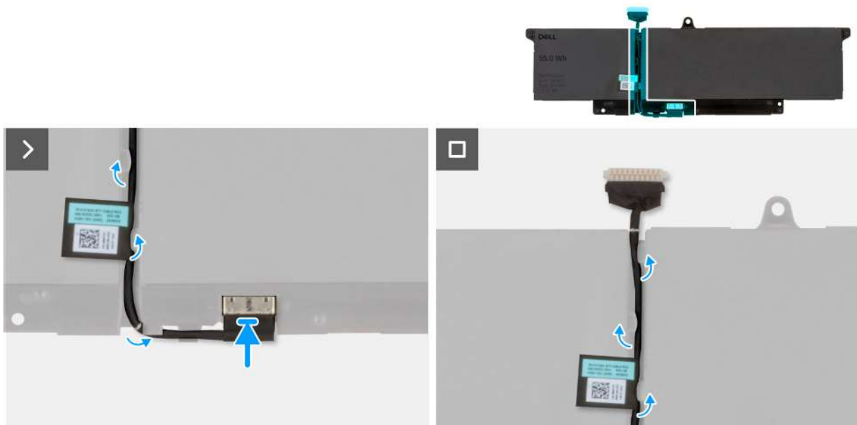
Rysunek 21. Instalowanie kabla baterii
