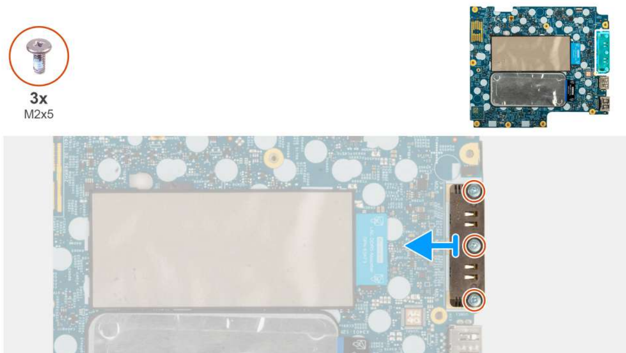
Rysunek 77. Wymontowywanie modułu łącznika USB Type-C
