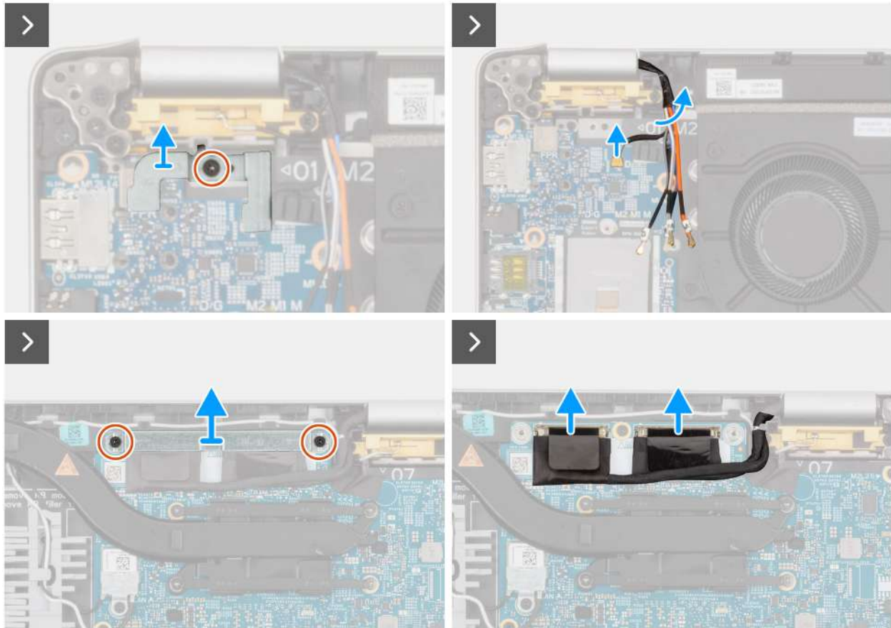
Rysunek 33. Wymontowywanie anteny sieci WLAN
