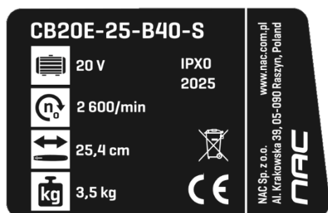
Tabliczka znamionowa
