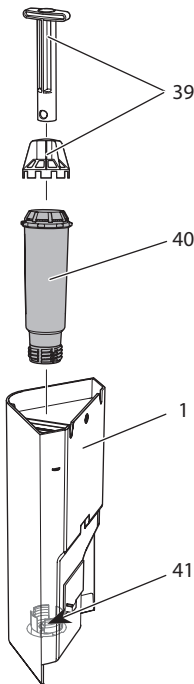
Рис. 20: Завинчивание и отвинчивание фильтра для воды
