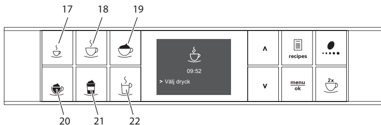
Bild 3: Snabbknappar
