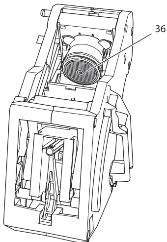
Kuva 18: Suodatusyksikön puhdistaminen
