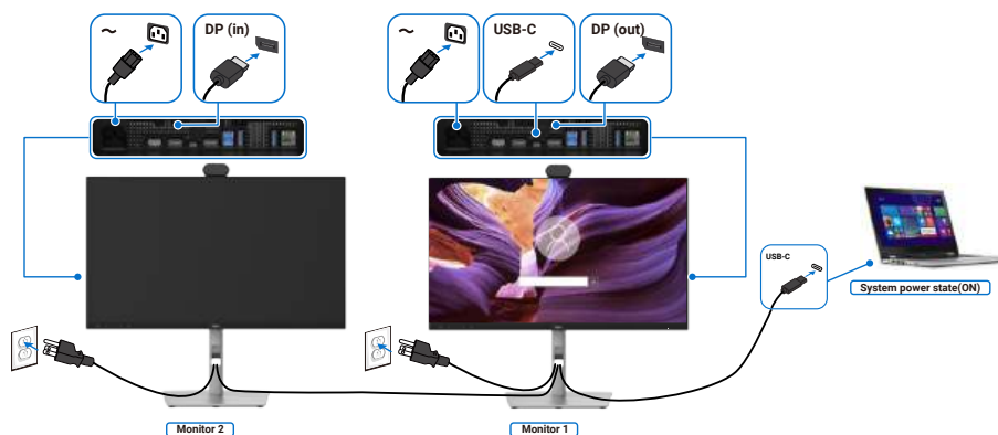
Rysunek 51. Podłączenie monitora w konfiguracji USB-C MST (Multi-Stream Transport) – włączenie
