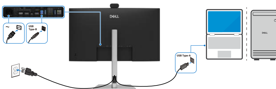
Rysunek 33. Podłączenie przewodu USB-A/USB-B
