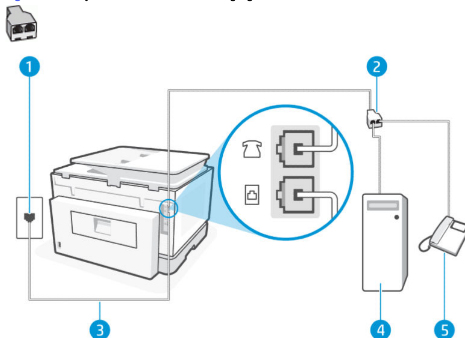
Figure 7-2 Przykład rozdzielacza równoległego
